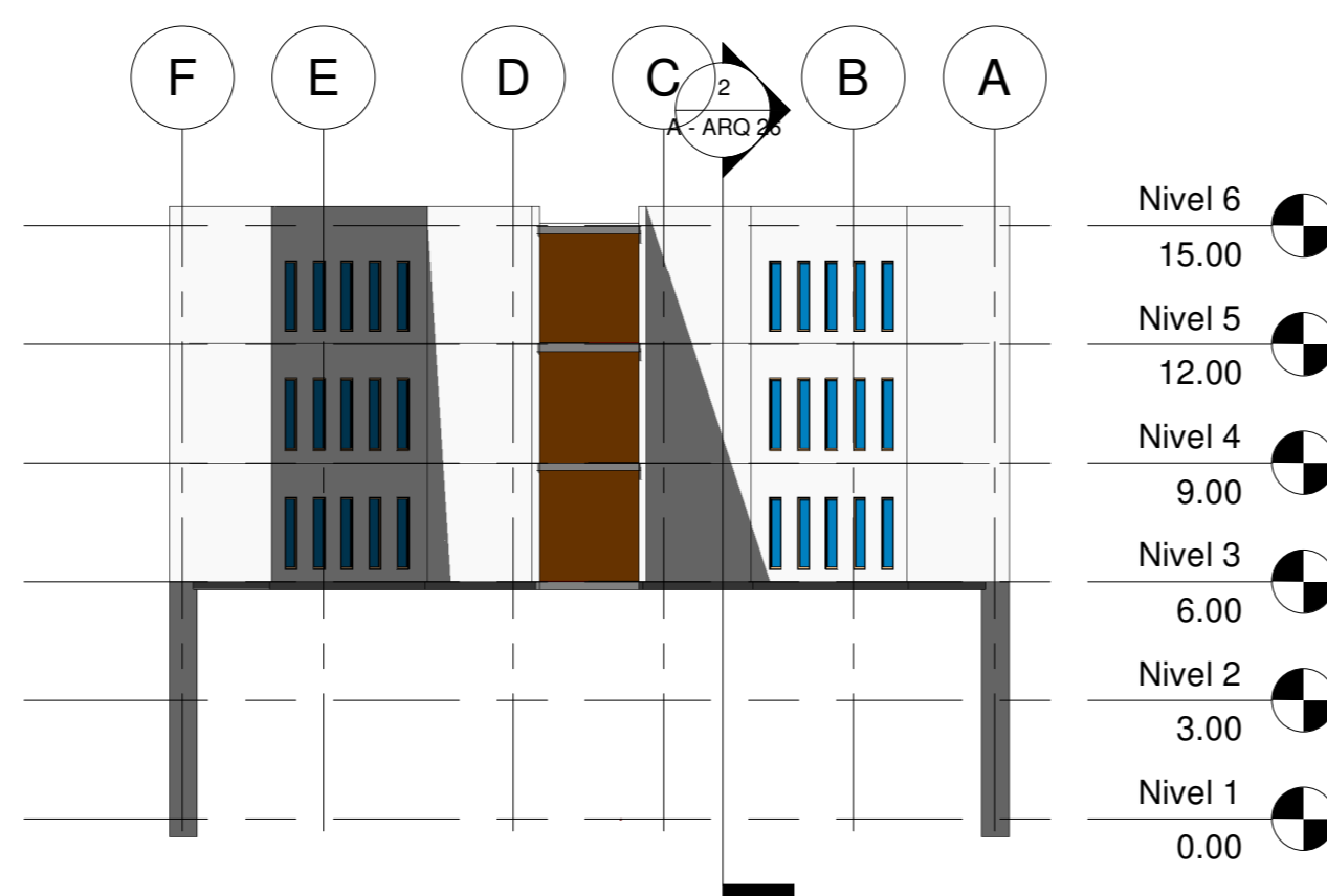
1 Este 1 : 200
