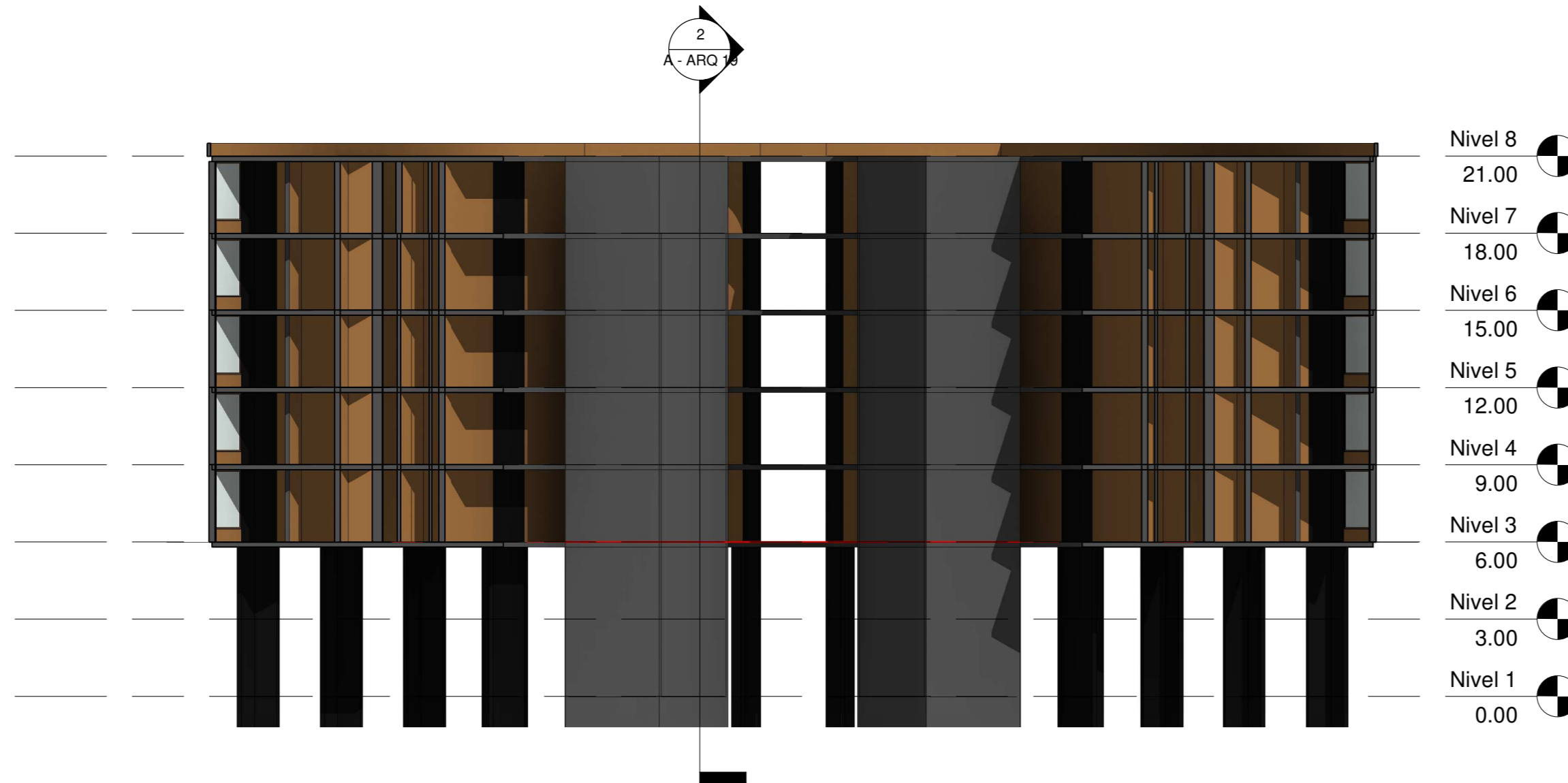
1 Sección 1 1 : 200
