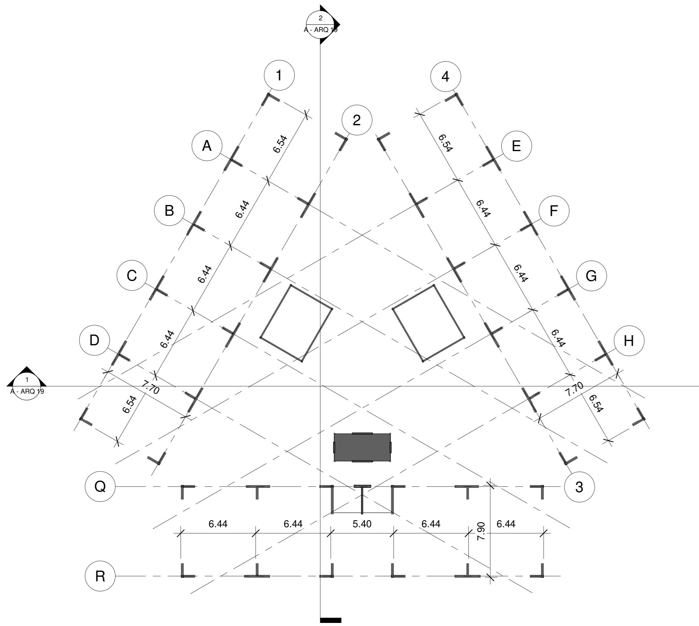
1 Nivel 1 1 : 200
