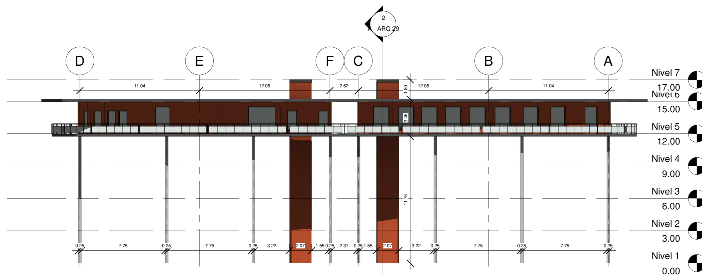
2 Norte 1 : 200
