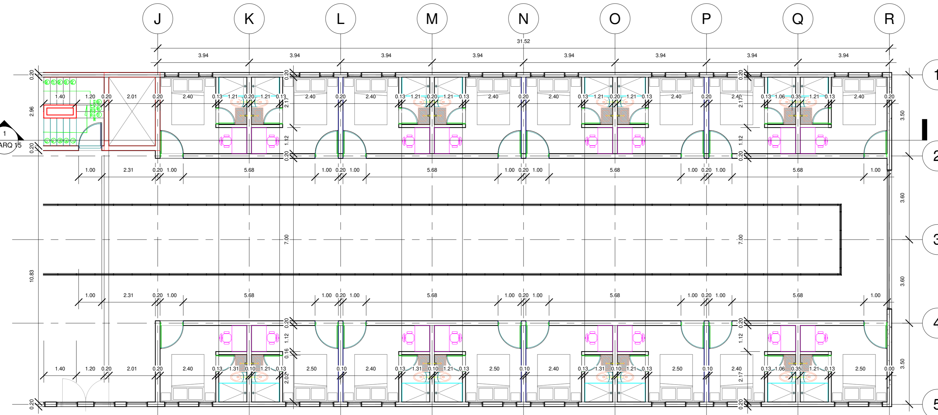
2 Nivel 2 Copia 1 1 : 100
