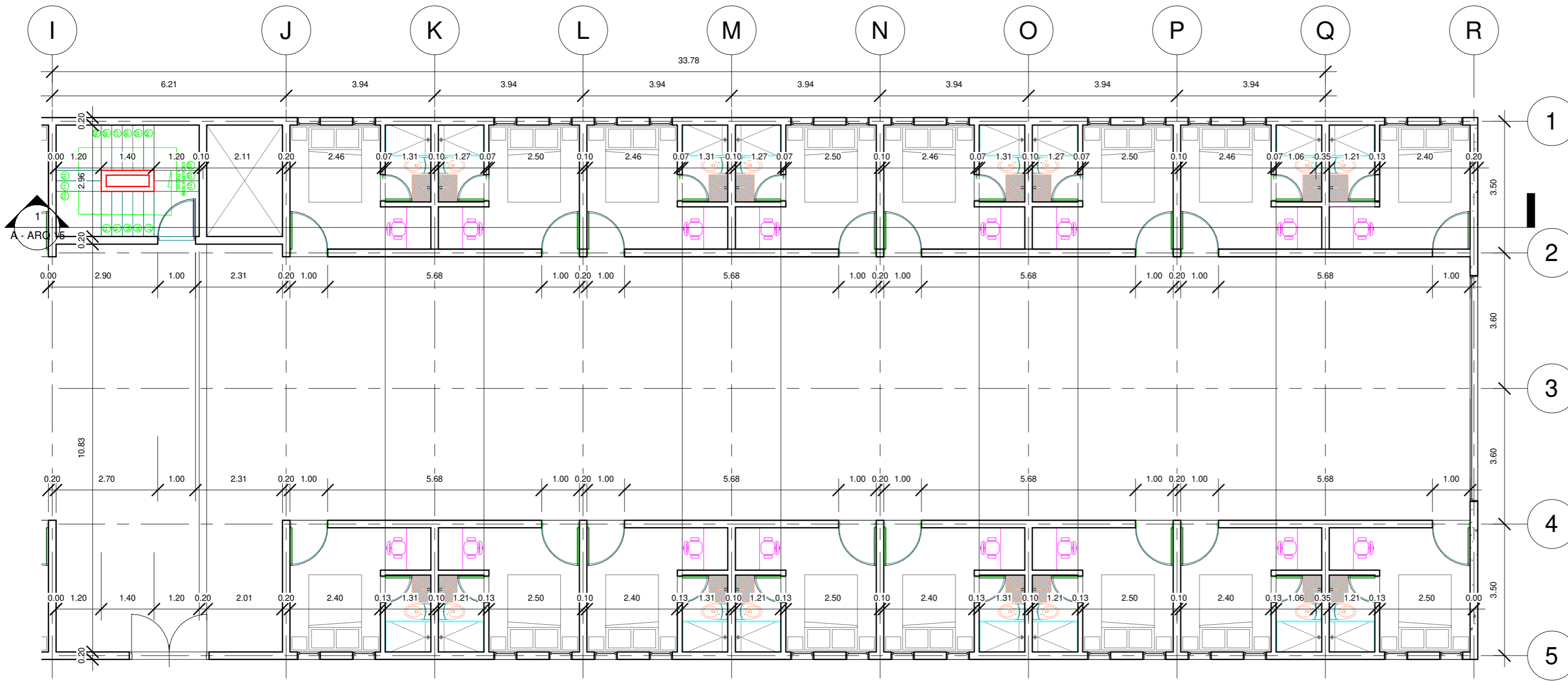
2 Nivel 1 Copia 1 1 : 100
