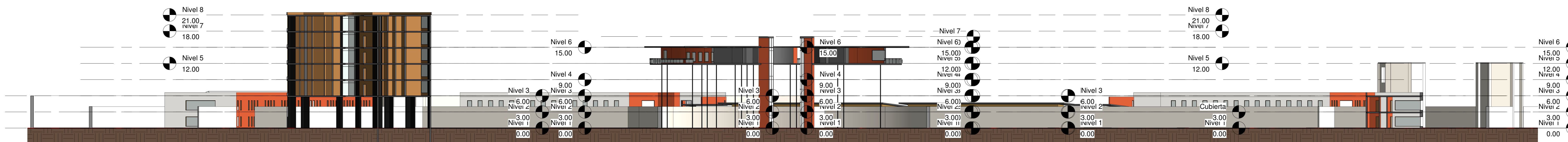
1 Este 1 : 300
