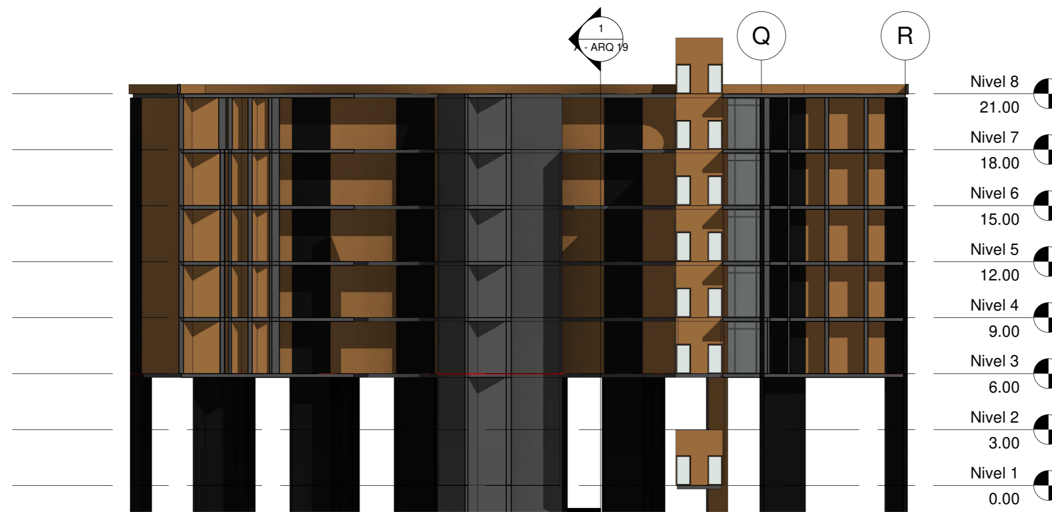
2 Sección 2 1 : 200
