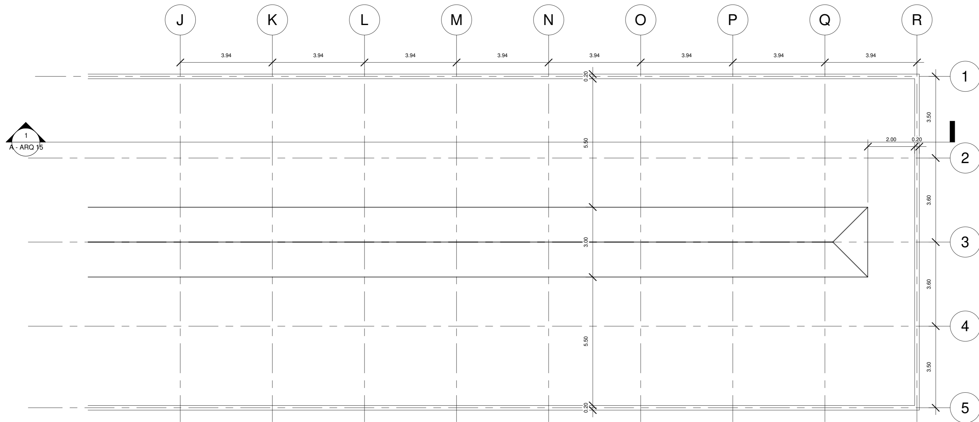
2 Nivel 3 Copia 1 1 : 100
