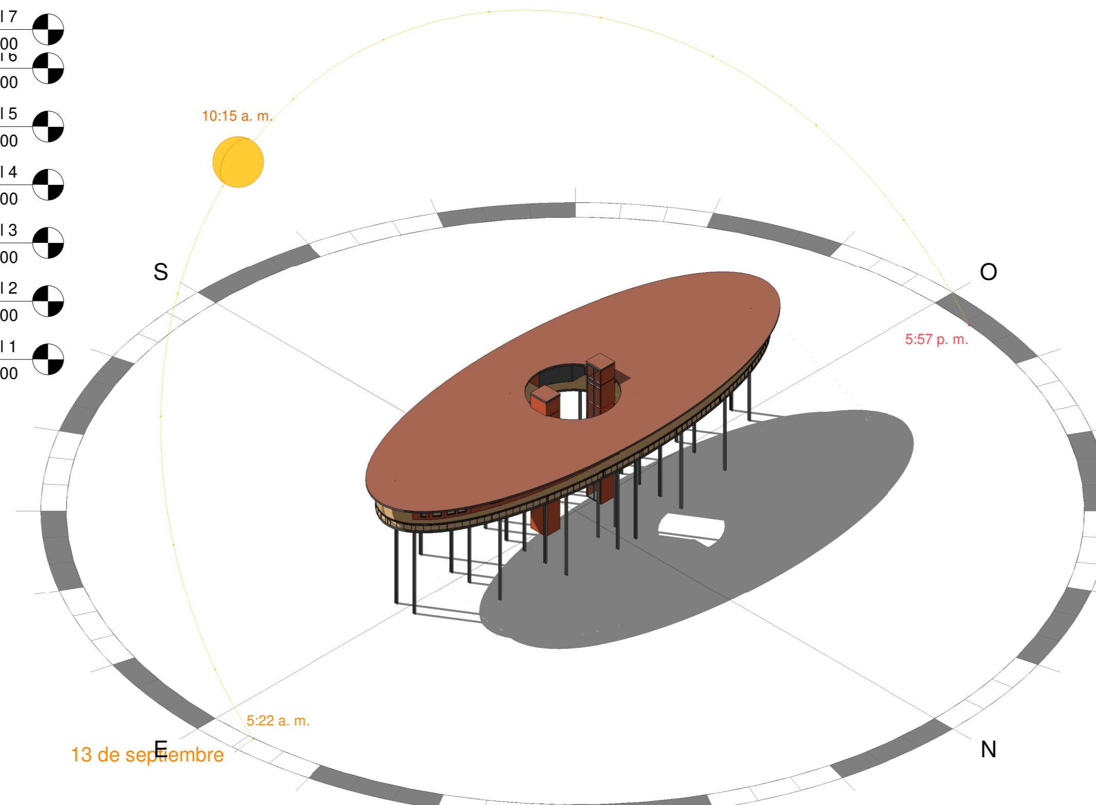
3 Isometrico
