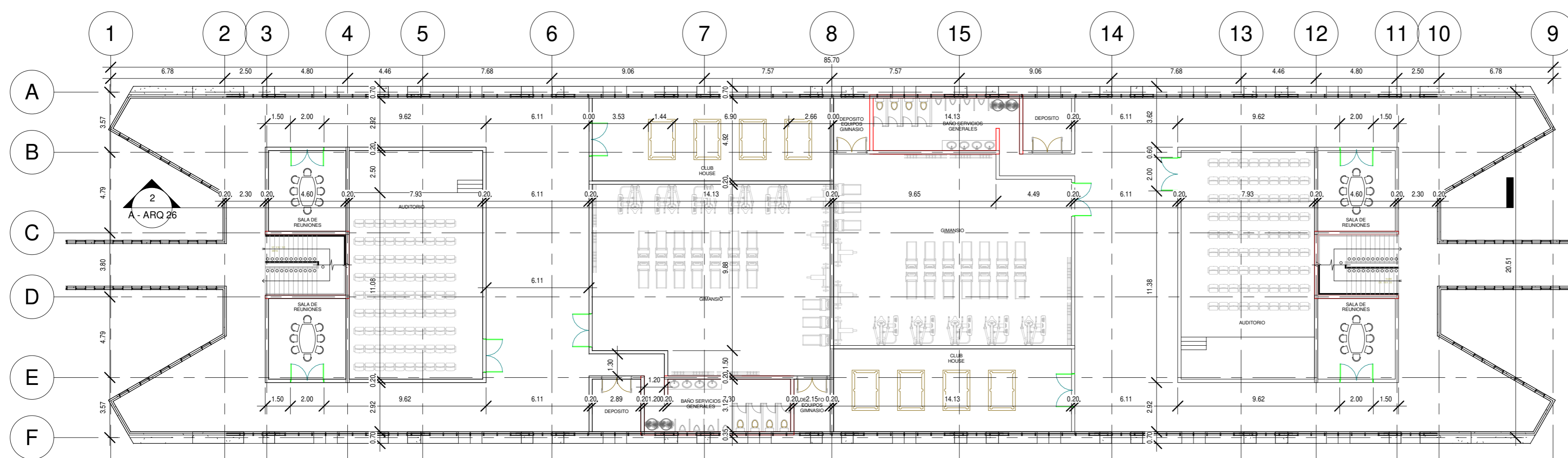
1 Nivel 5 1 : 200
