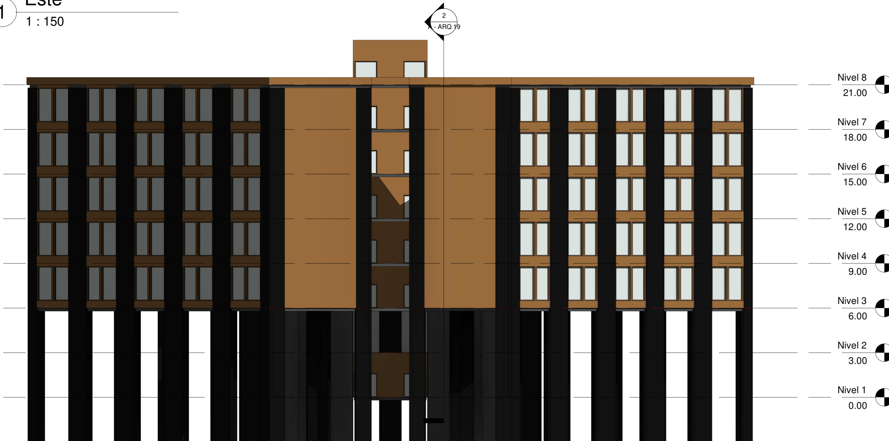
2 Norte 1 : 150
