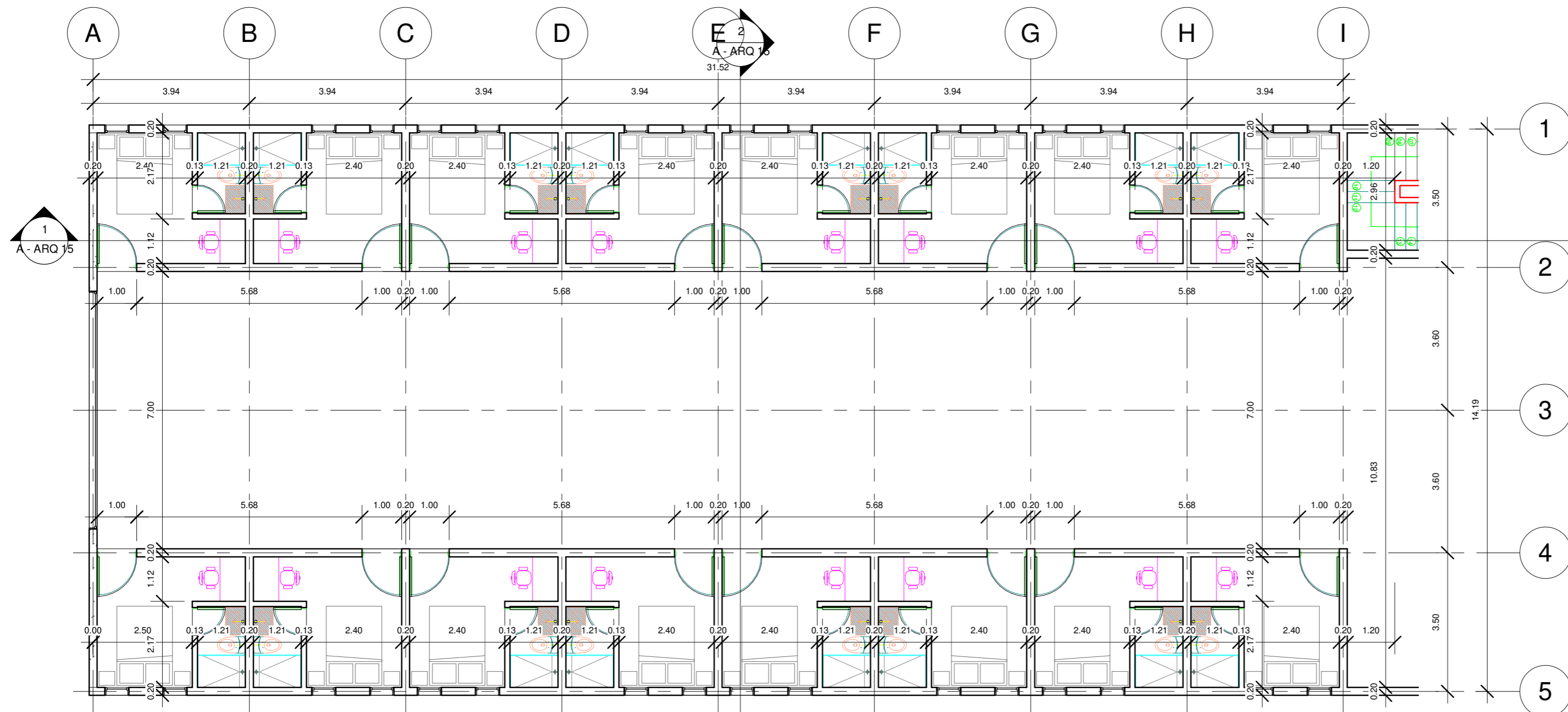
1 Nivel 1 1 : 100
