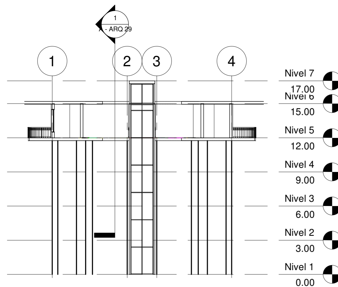
2 Sección 2 1 : 200
