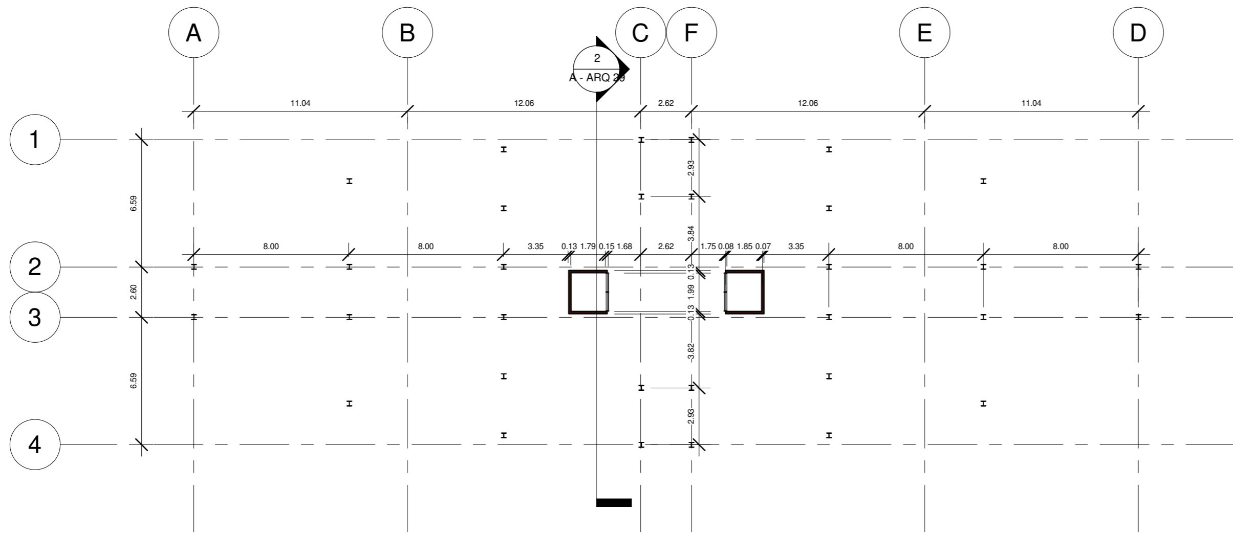
1 Nivel 1 1 : 200
