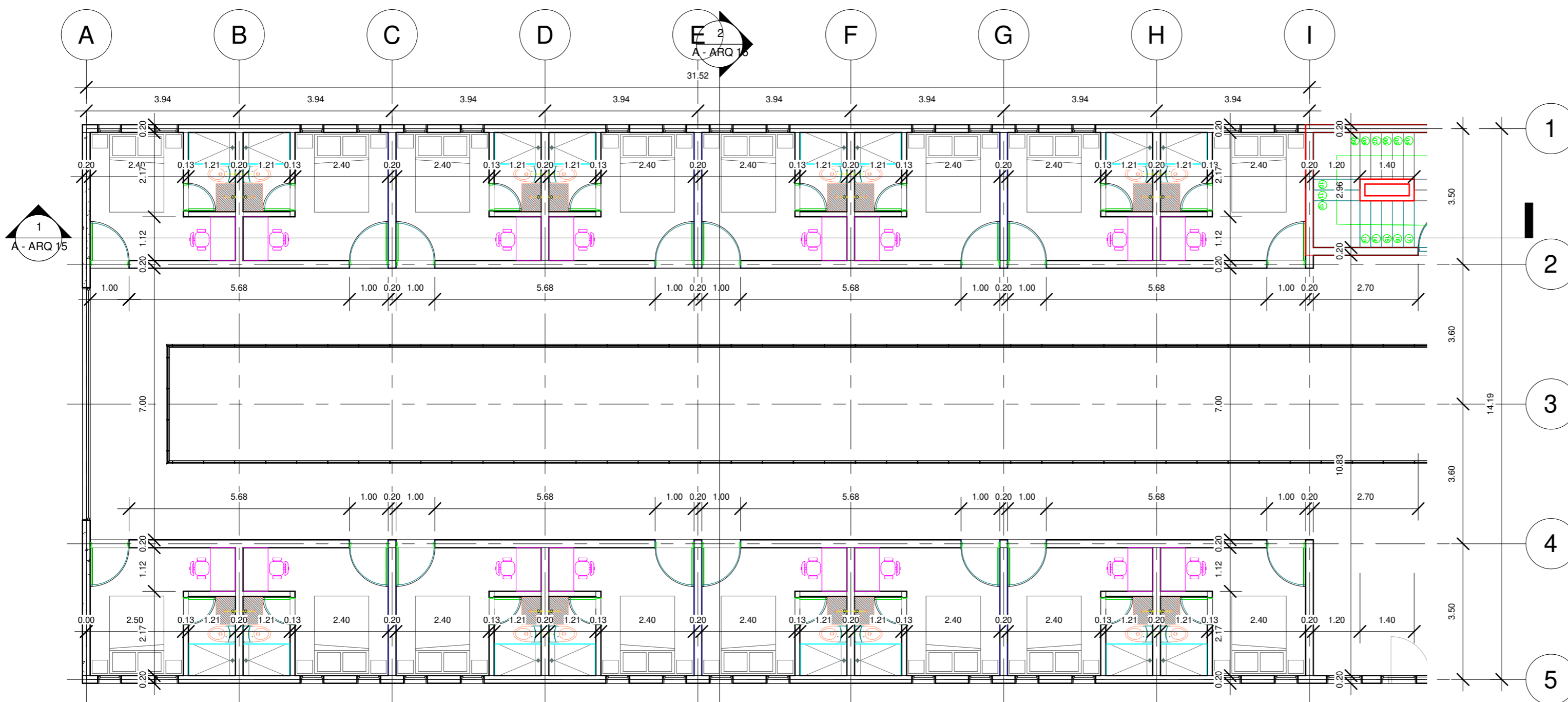
1 Nivel 2 1 : 100
