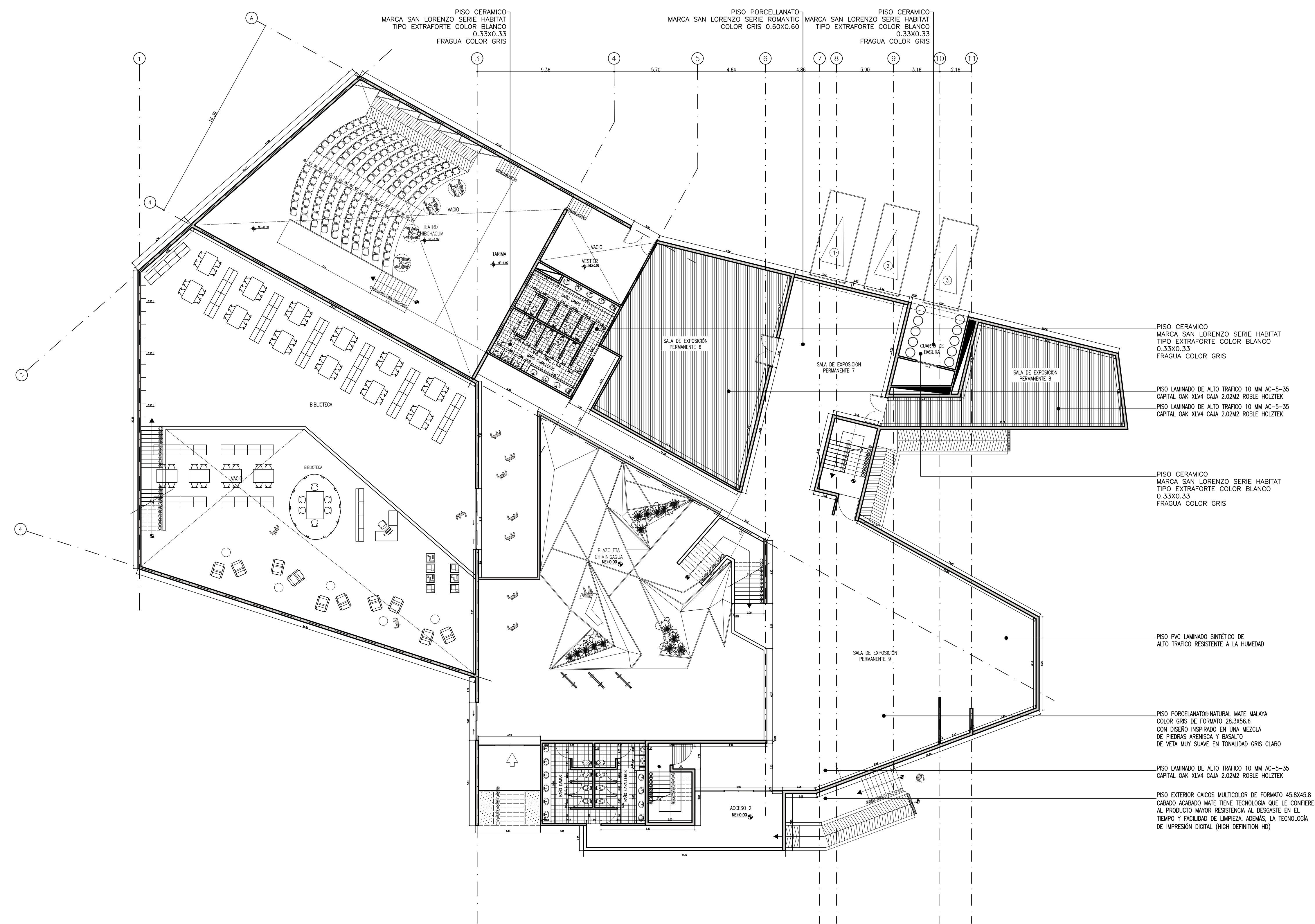
PT PLANTA TERCER PISO A-104 ESC: 1:150
