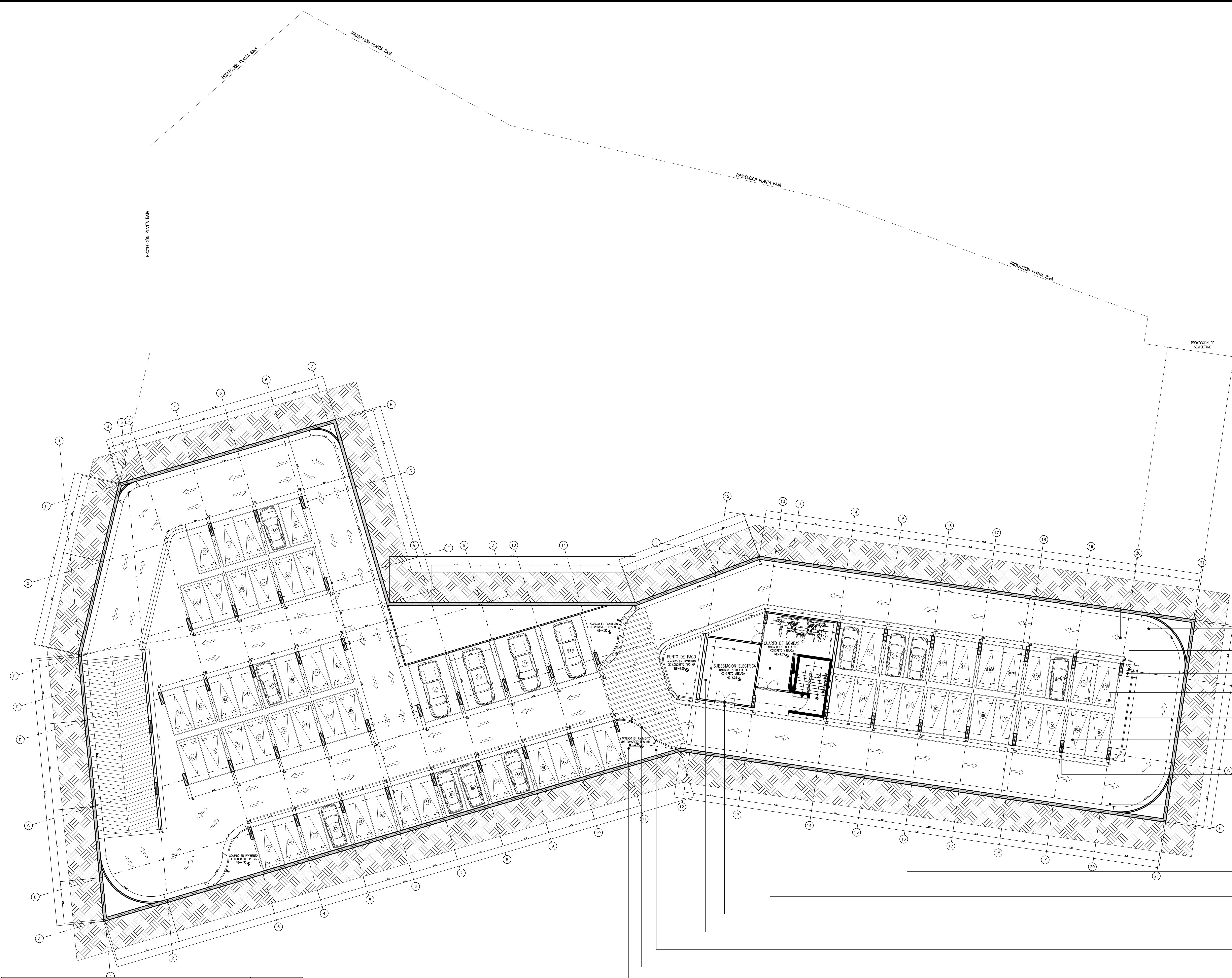
PS1 PLANTA SOTANO 1 A-100 ESC: 1:150
