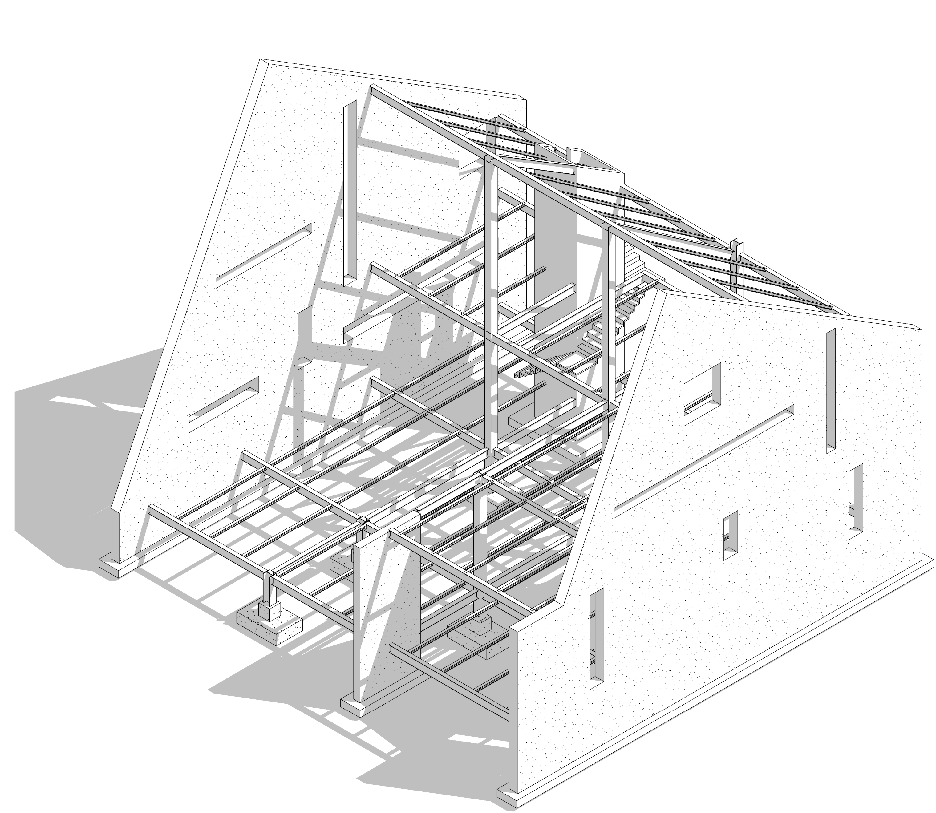
1 ISOMETRICO LATERAL
