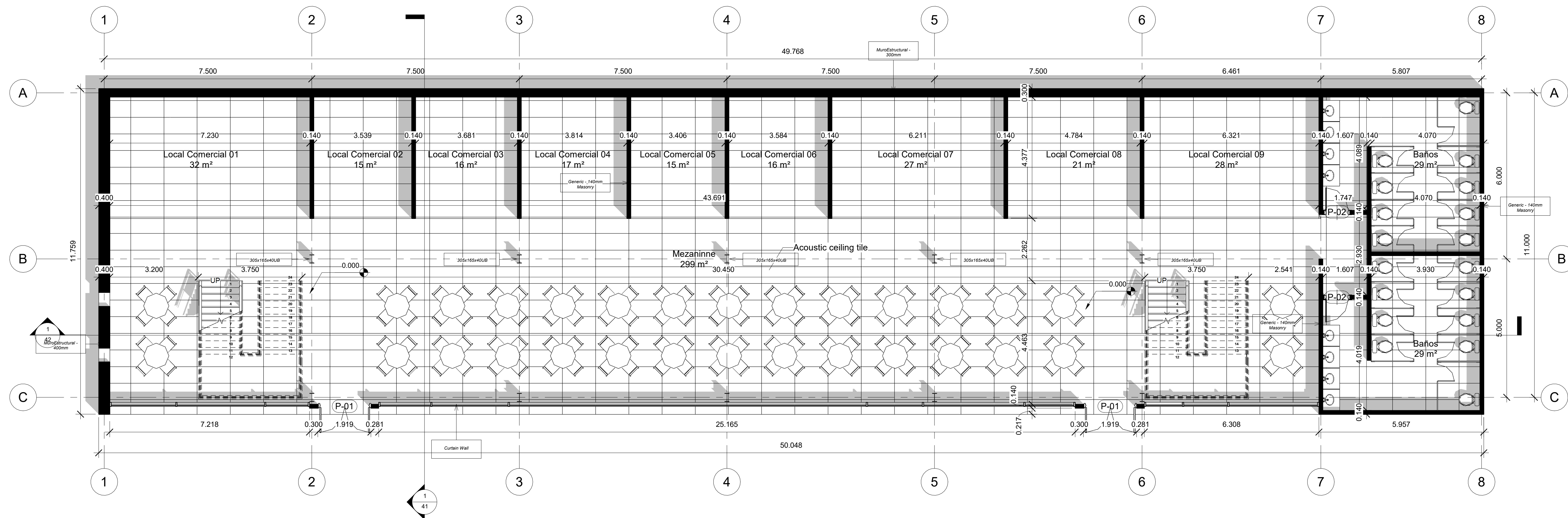
1 Planta 01 1 : 75
