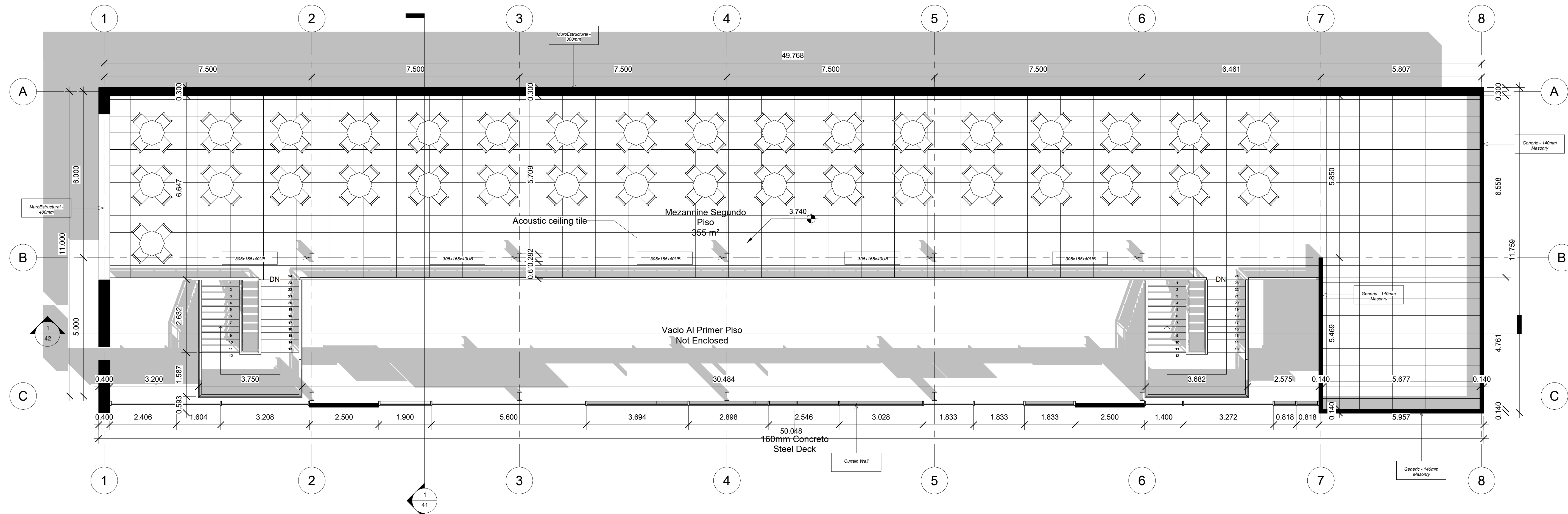
2 Planta 02 1 : 75
