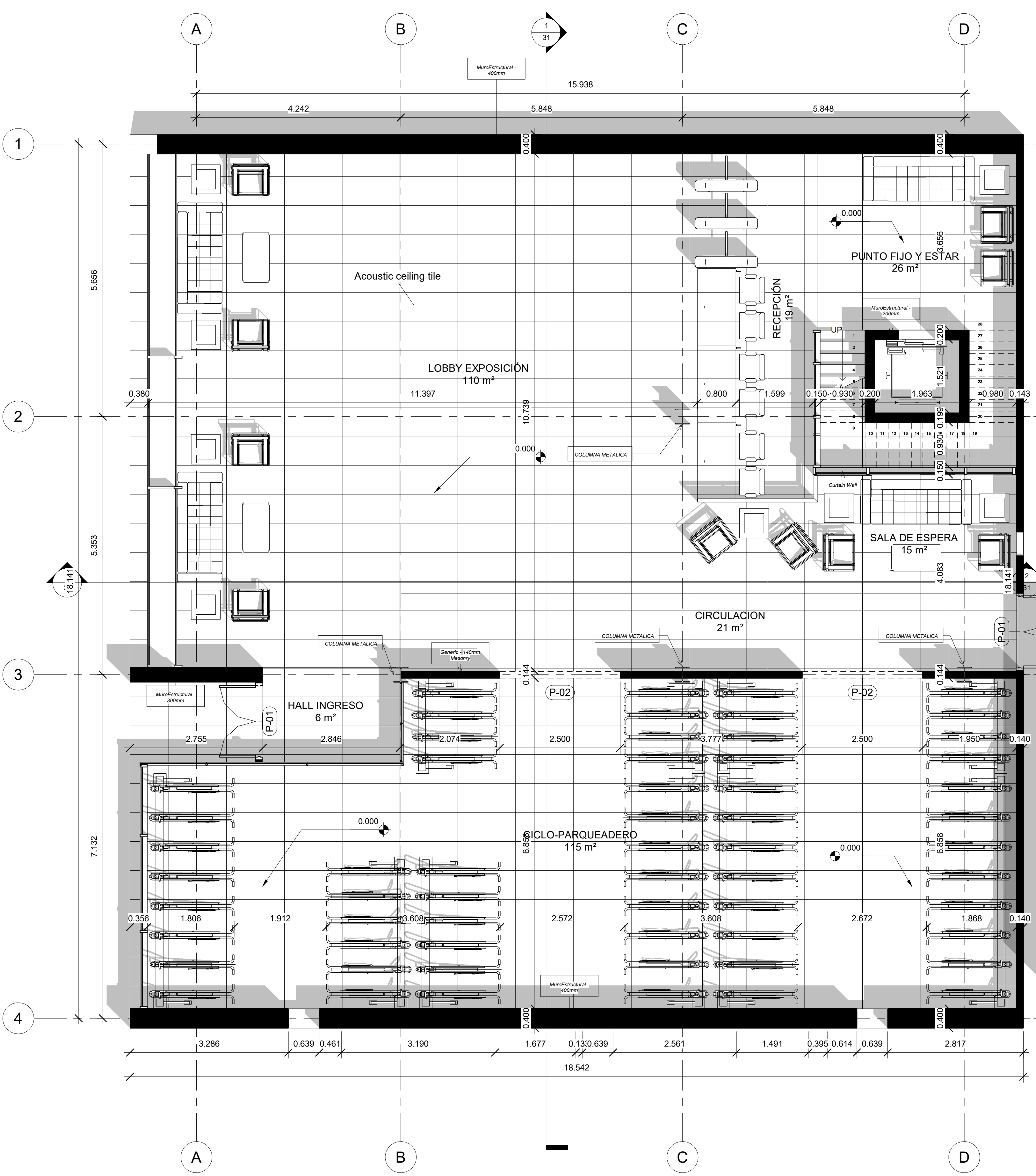
1 Level 1 1 : 50
