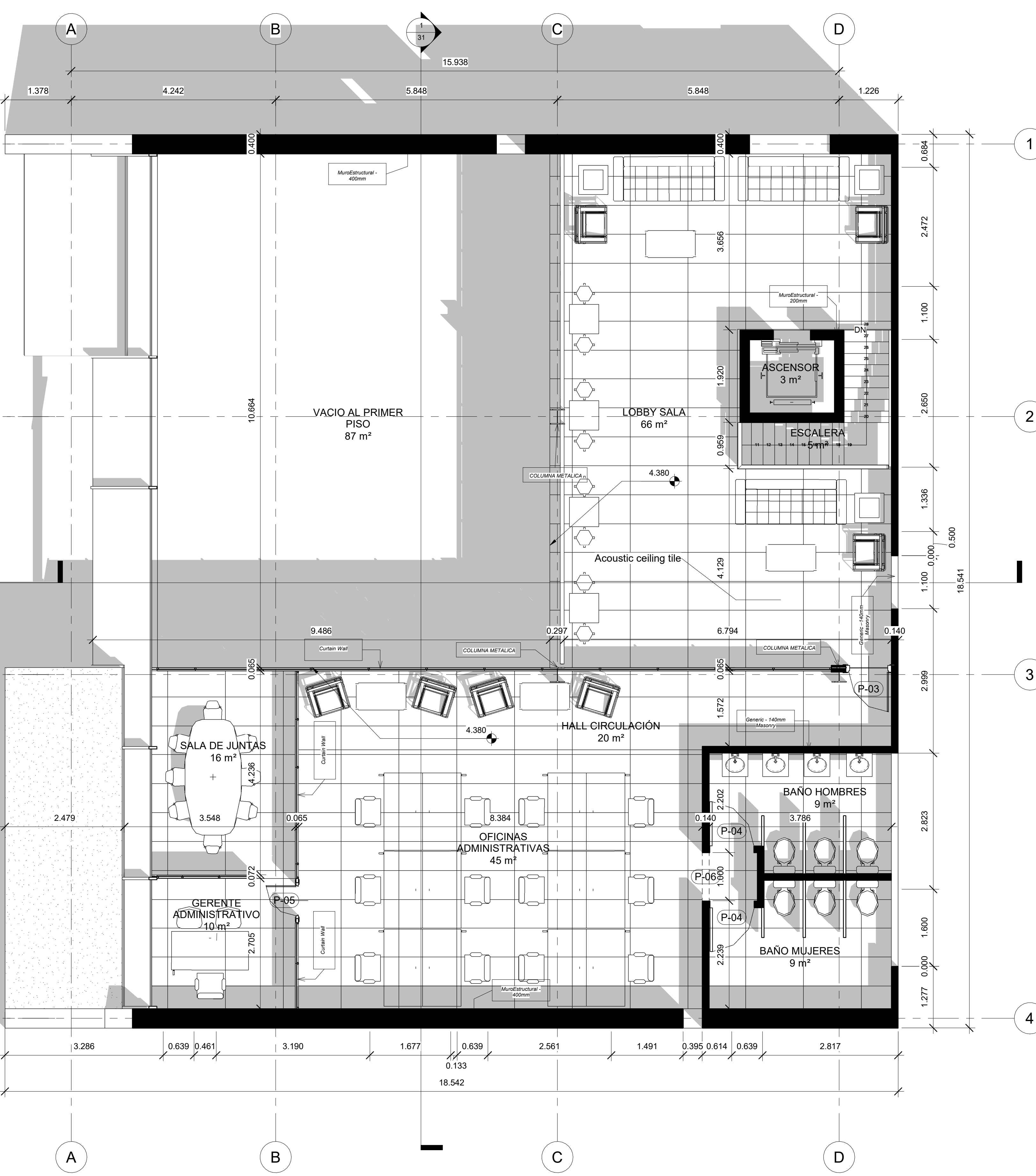
2 Level 2 1 : 50
