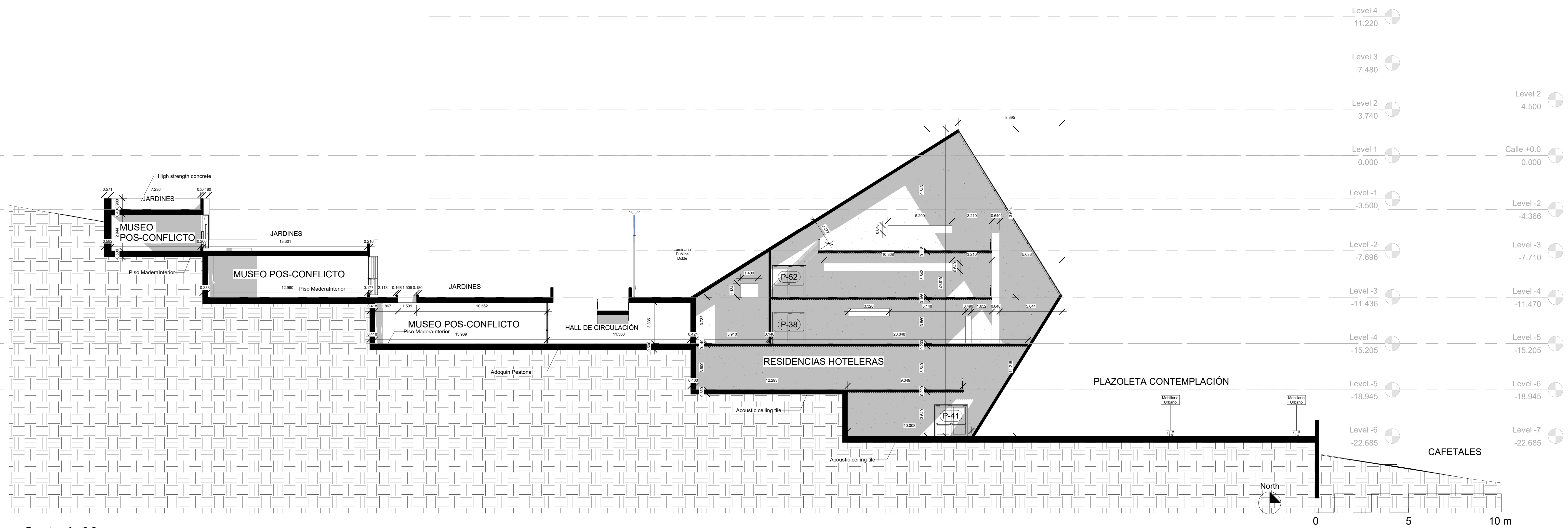
1 Corte A-03 1 : 150
