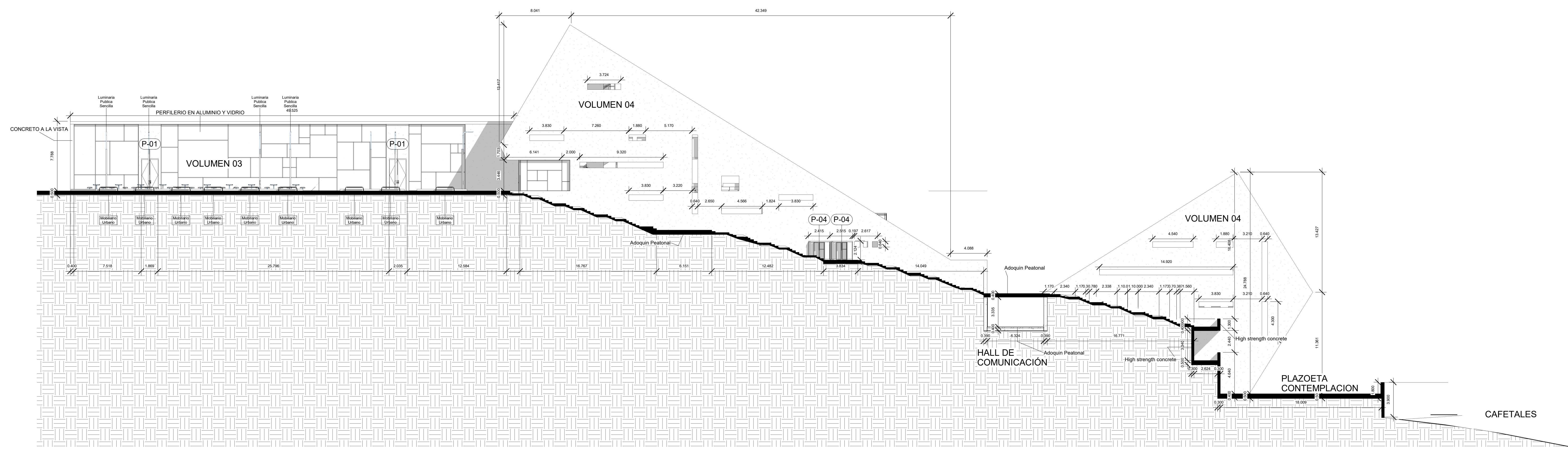
1 Corte A-01 1 : 200
