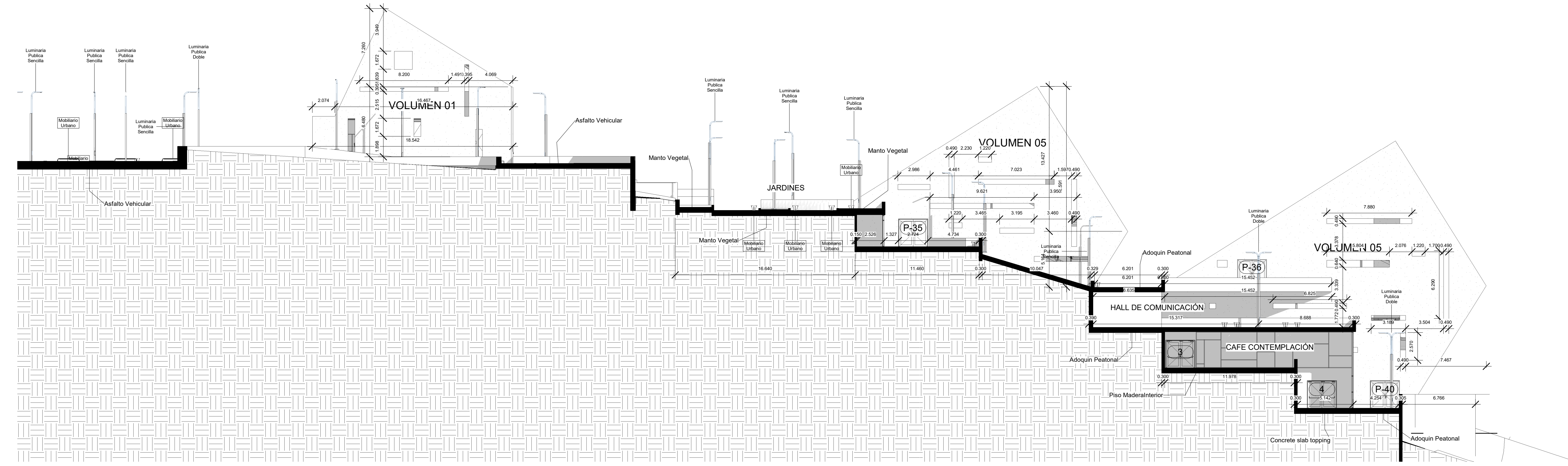
2 Corte A-02 1 : 200
