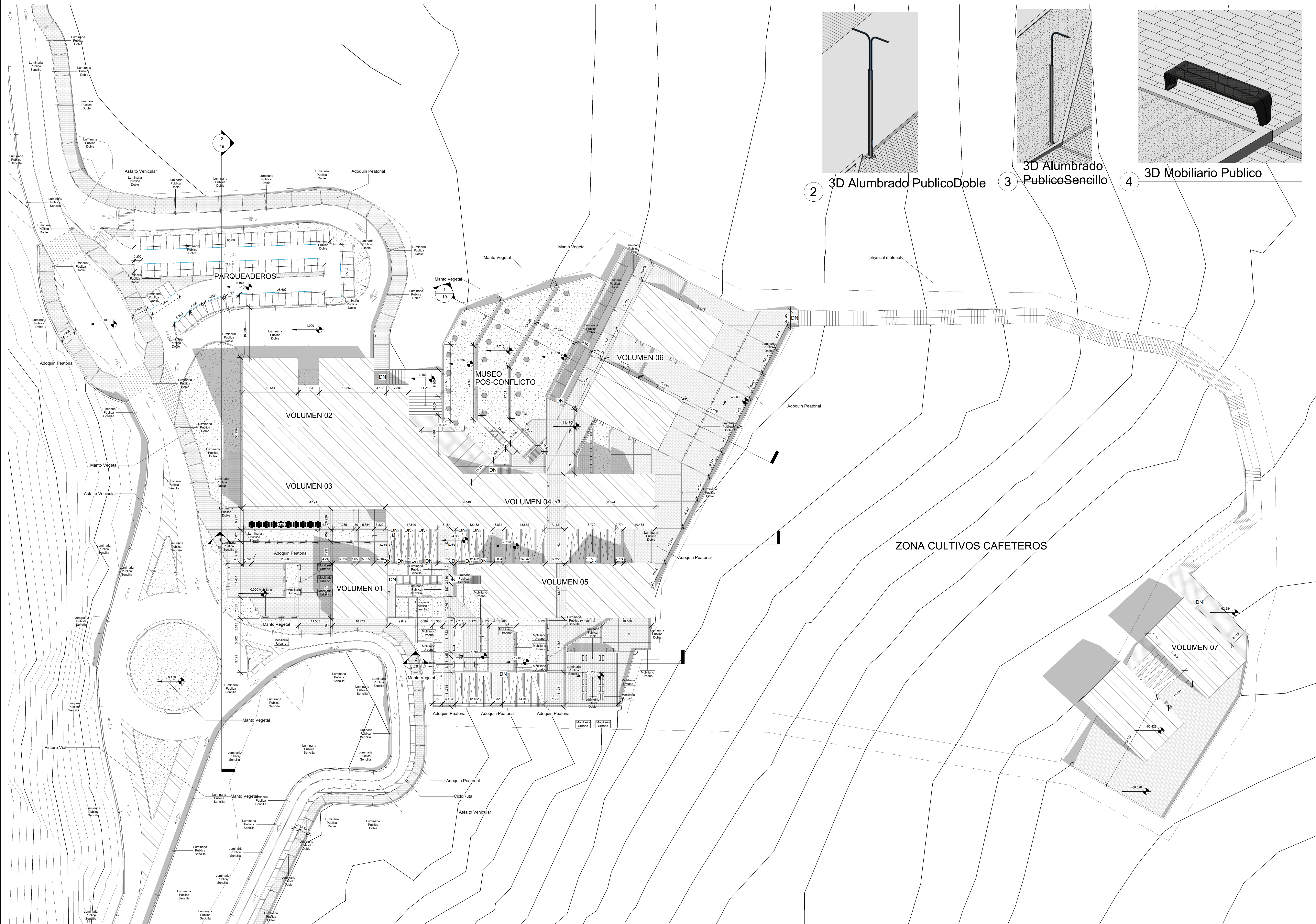
1 Planta General - Espacio Publico 1 : 500
