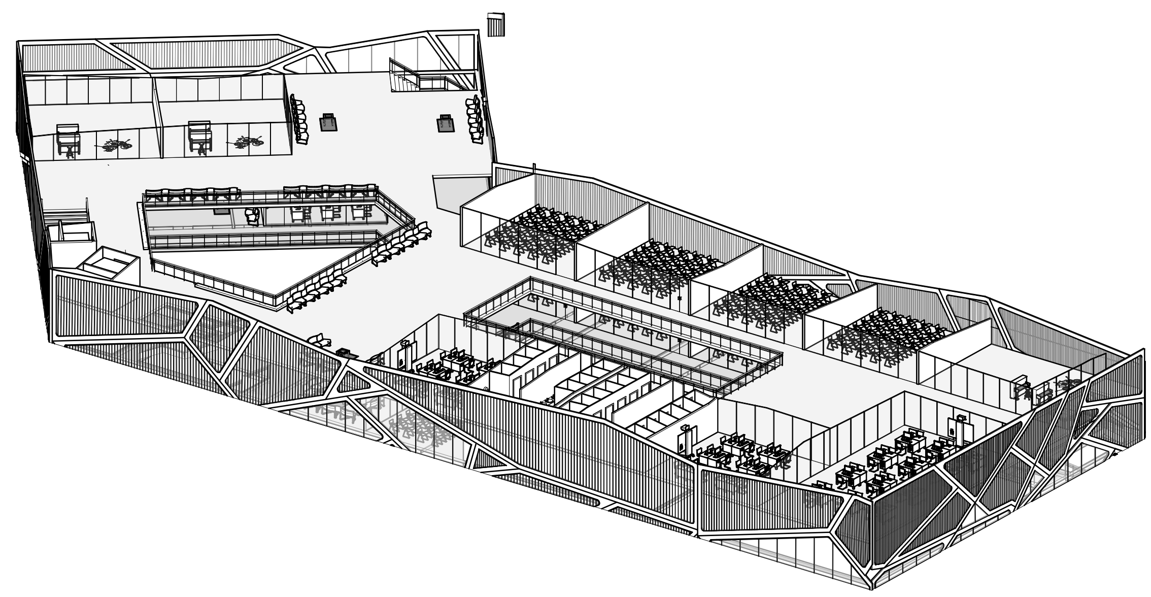
2 ISOMETRICO PLANTA 3
