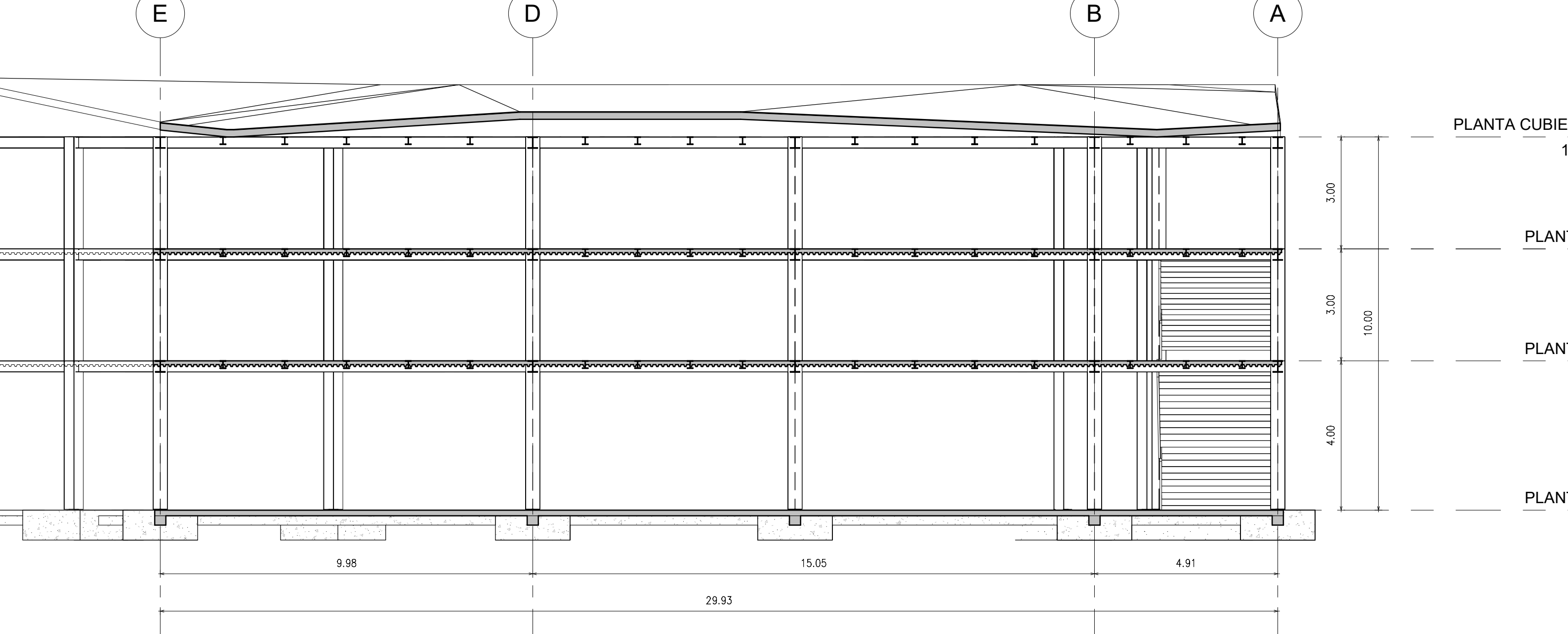
CORTE A-A
