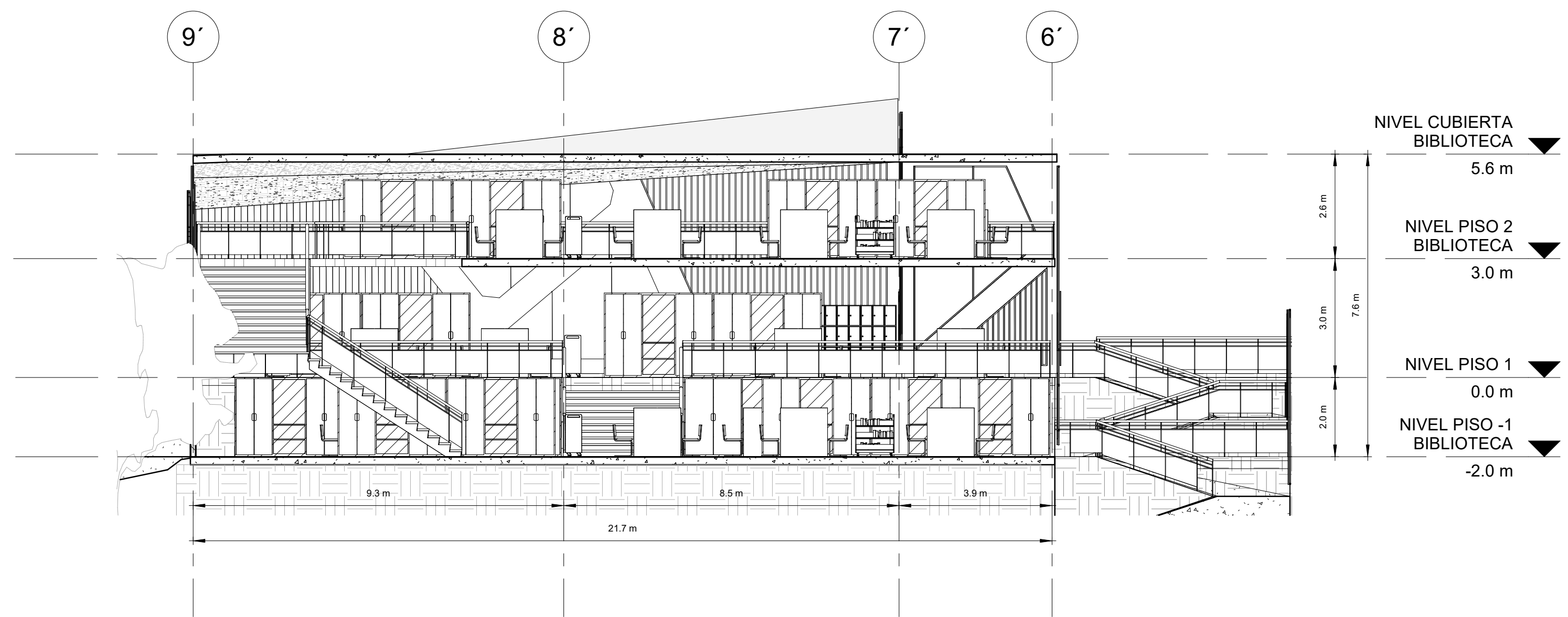
1 CORTE F-F 1:100
