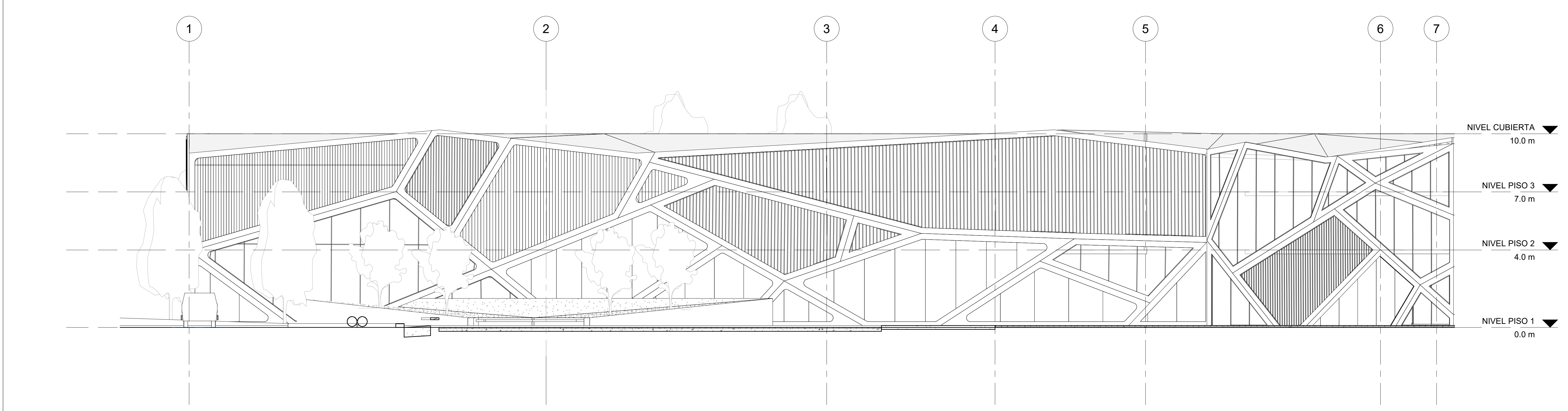
4 ALZADO ORIENTE 1:100
