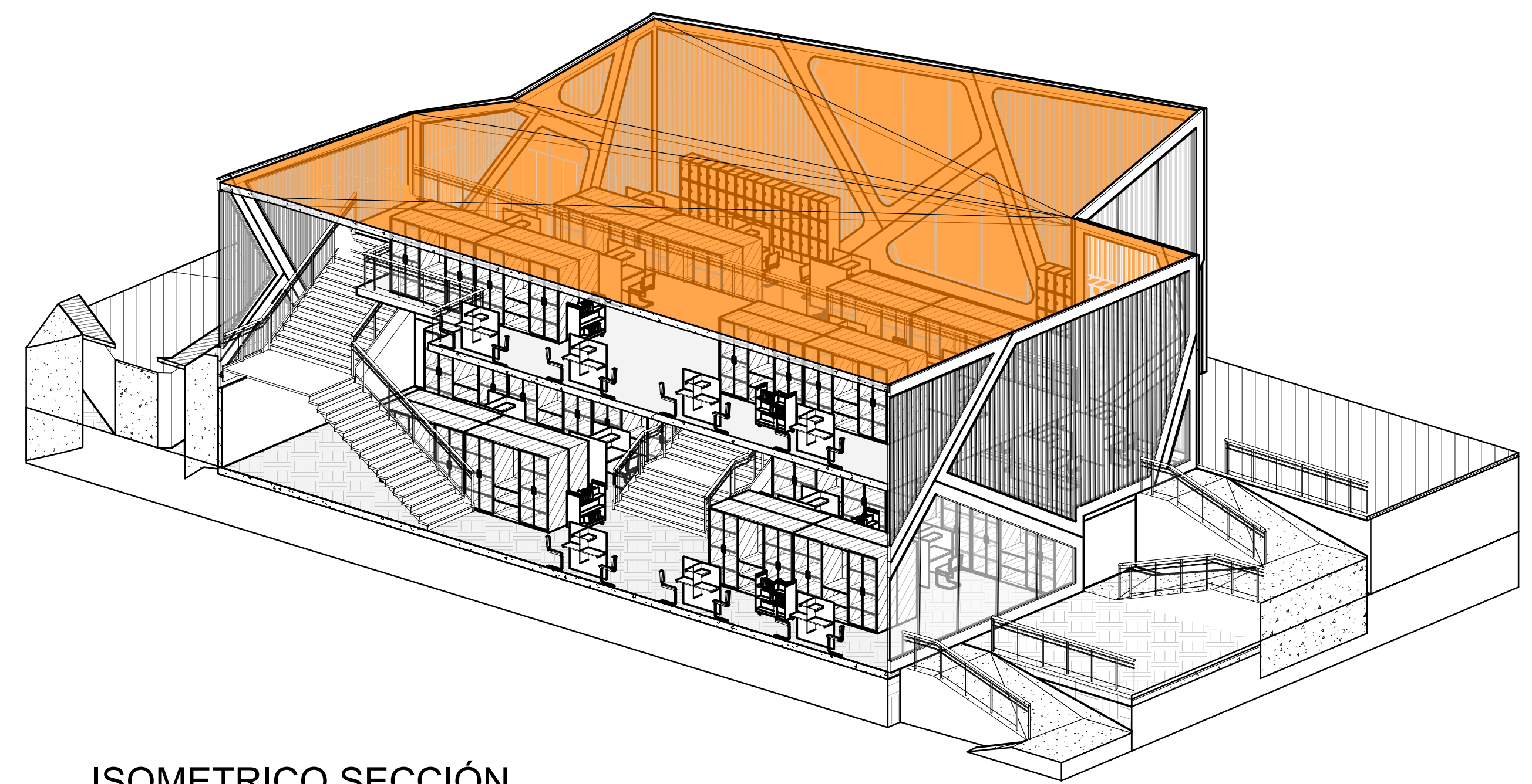
5 ISOMETRICO SECCIÓN F-F
