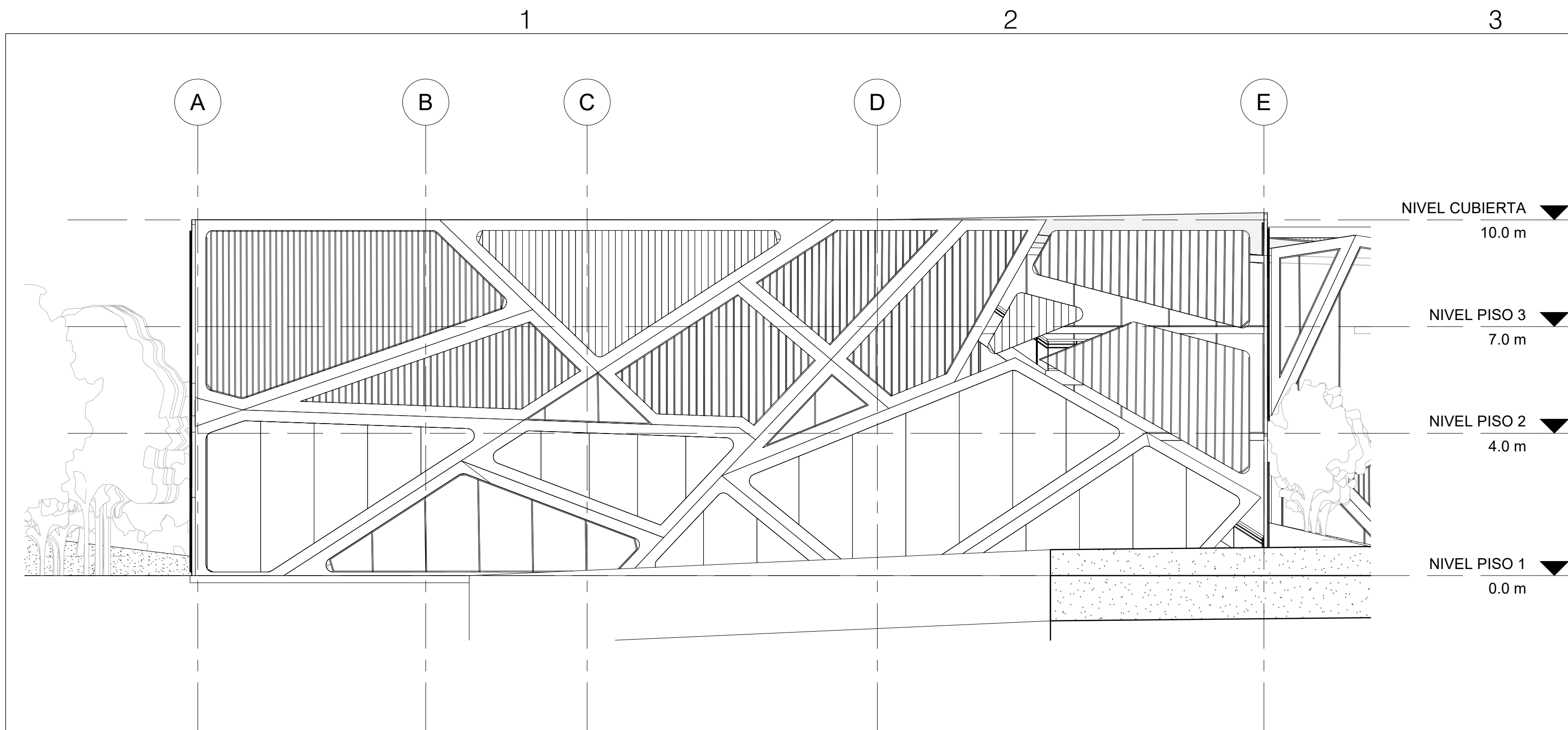
1 ALZADO NORTE 1:100
