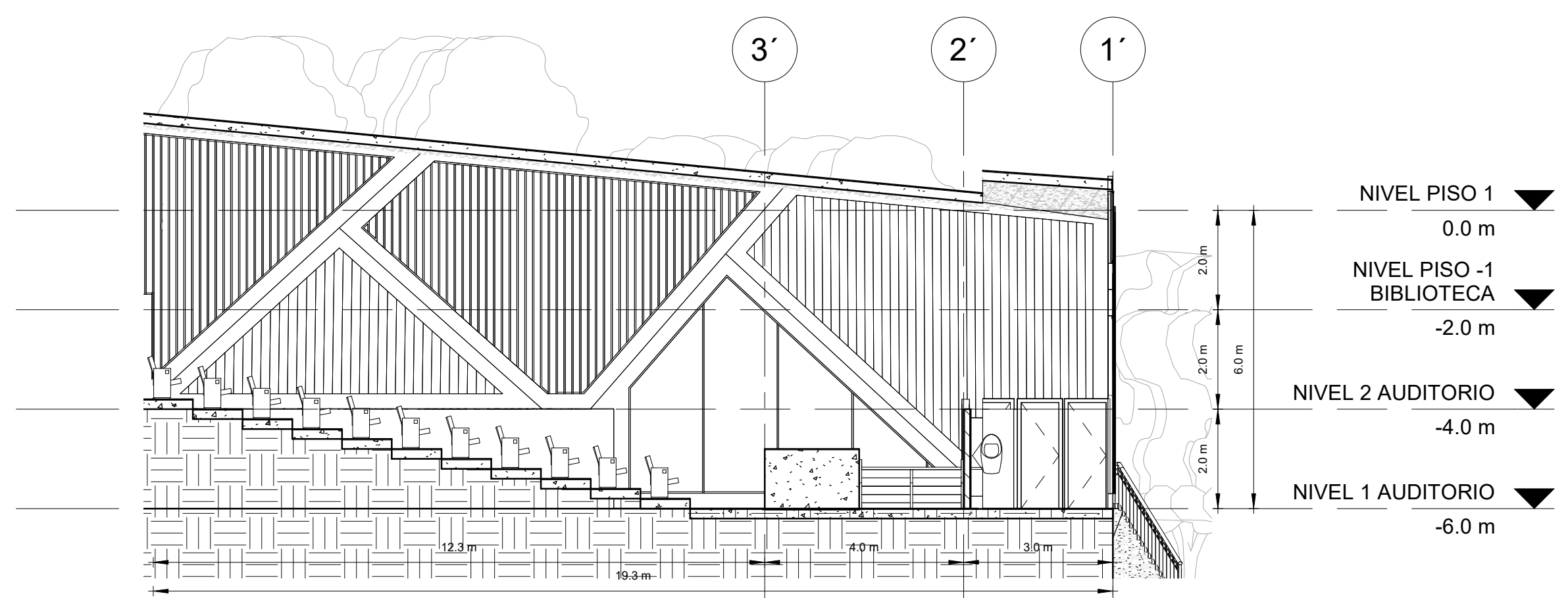
2 CORTE G-G 1:100
