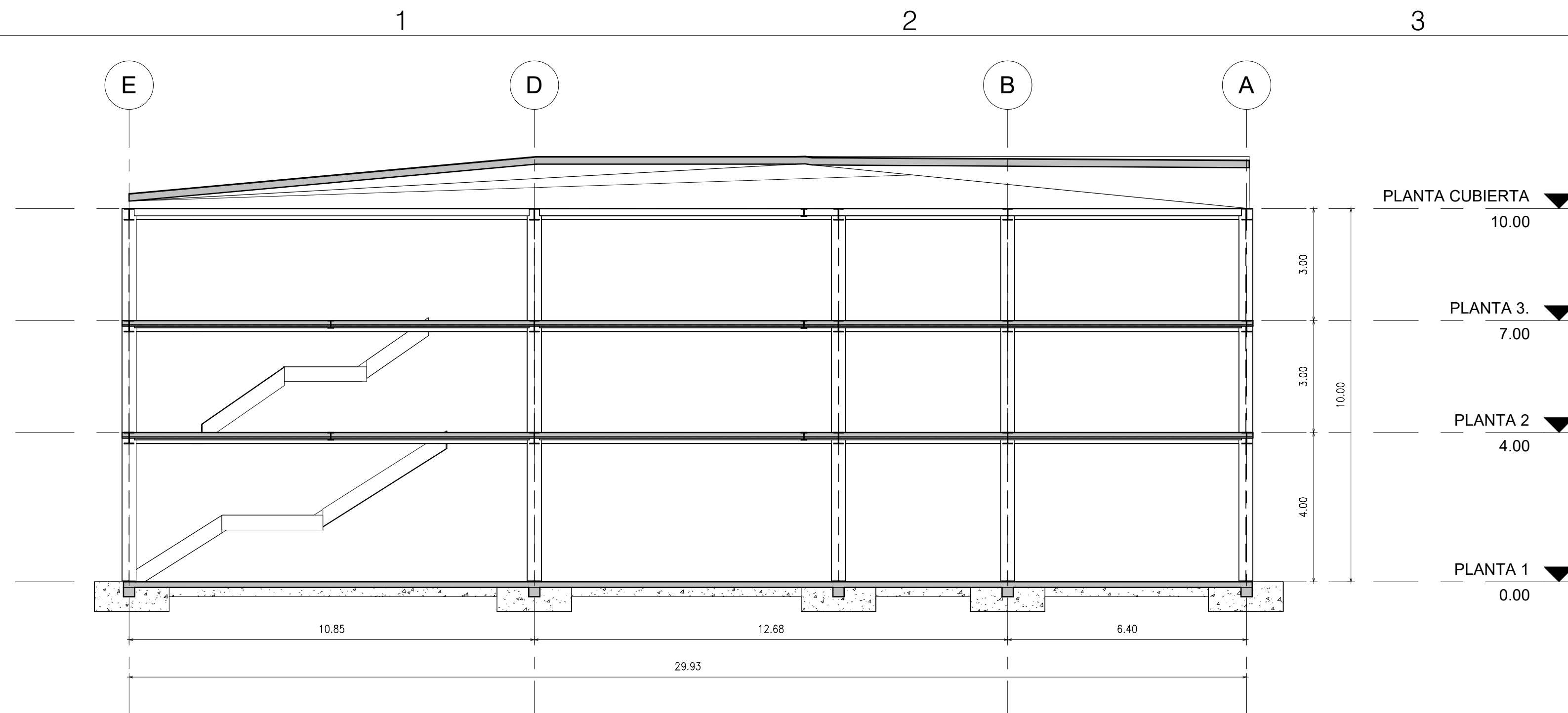
CORTE A-A
