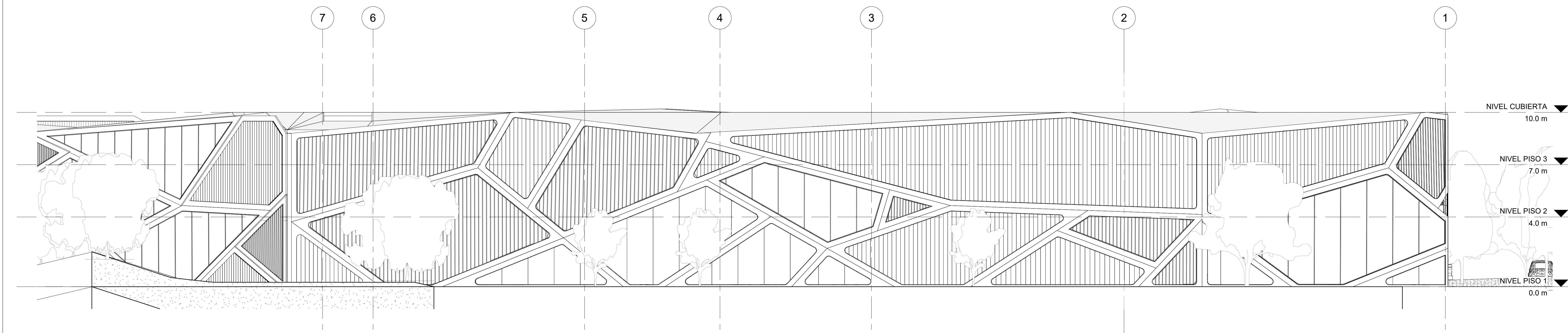
3 ALZADO OCCIDENTE 1:100
