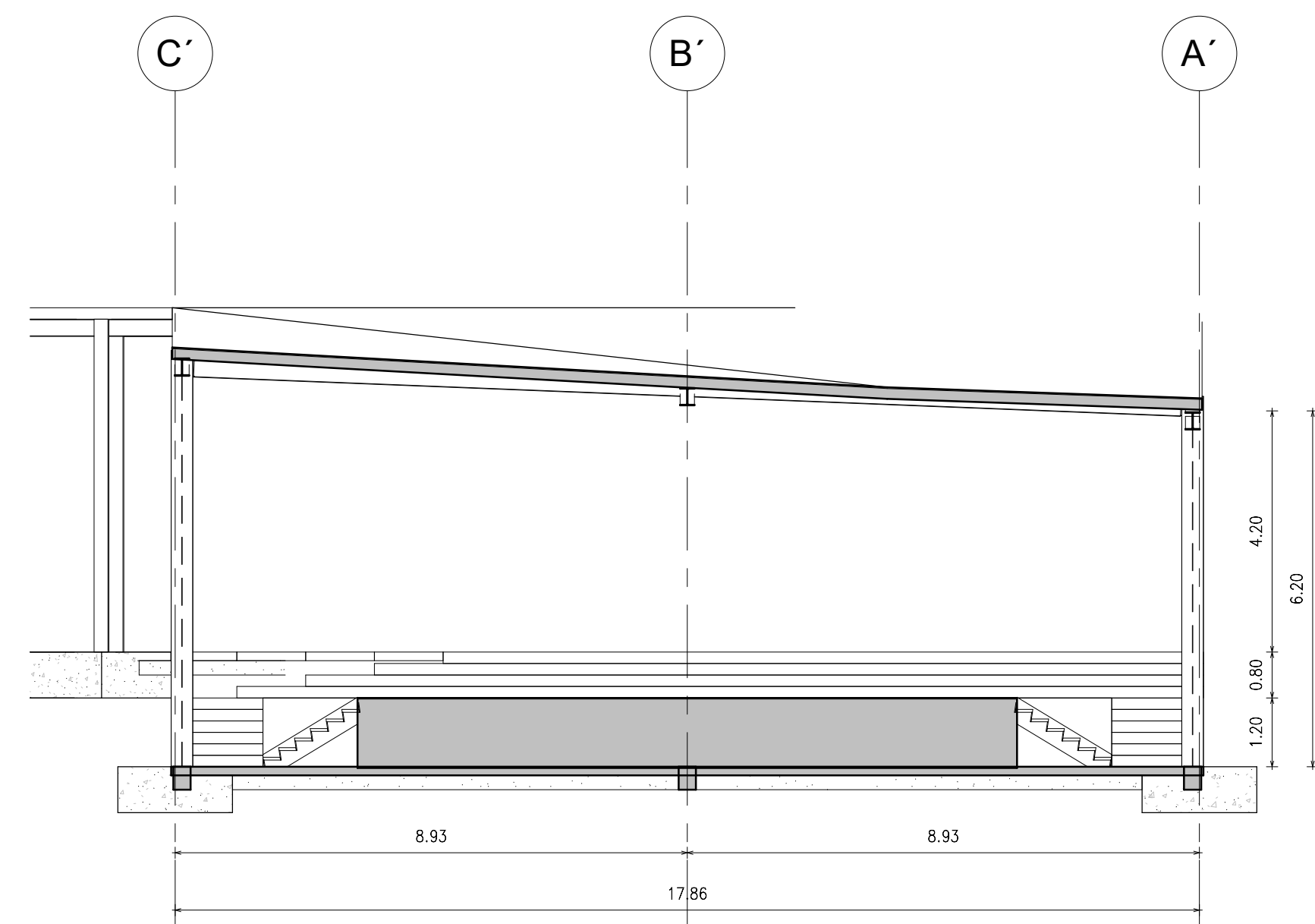
CORTE E-E 1 : 100
