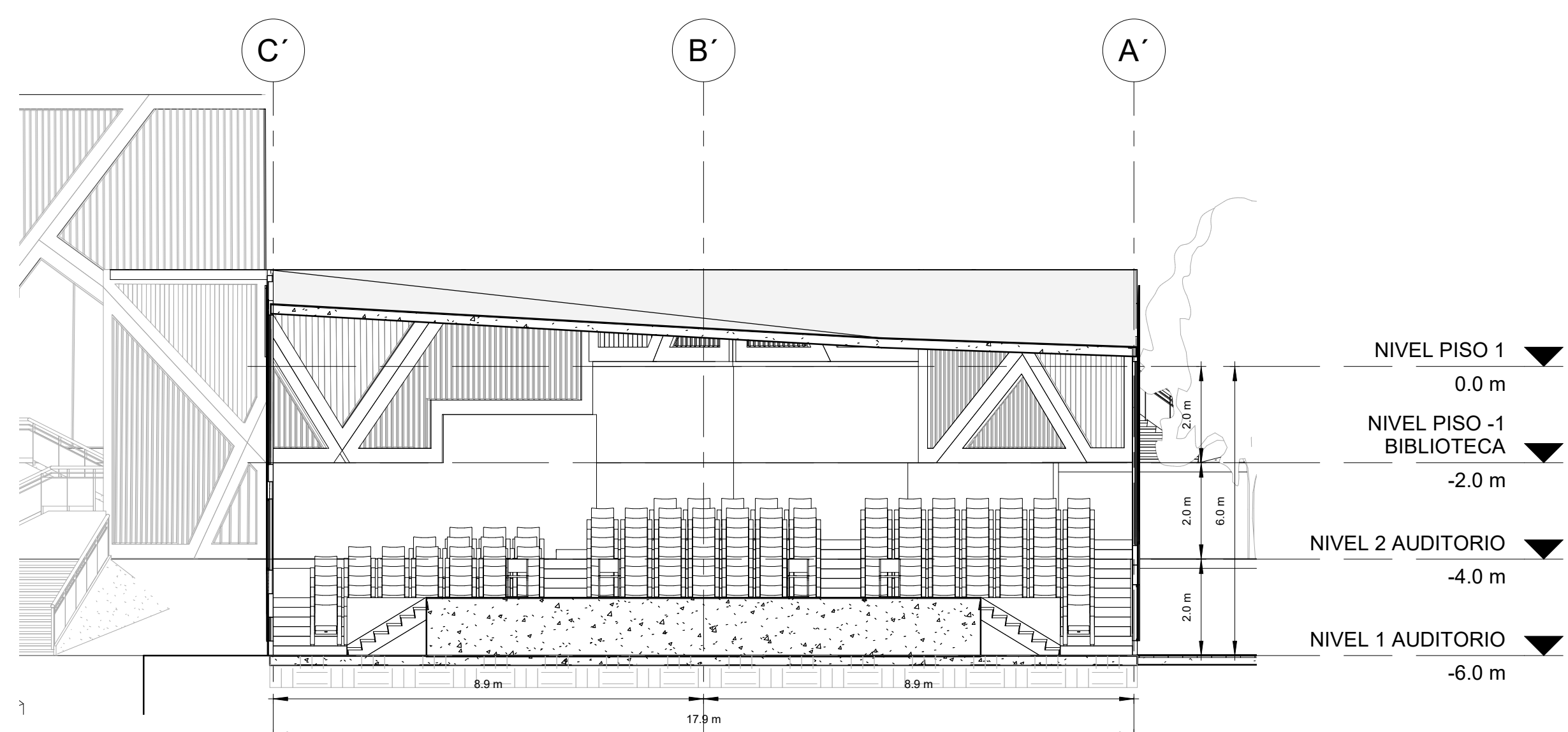
3 CORTE H-H 1:100
