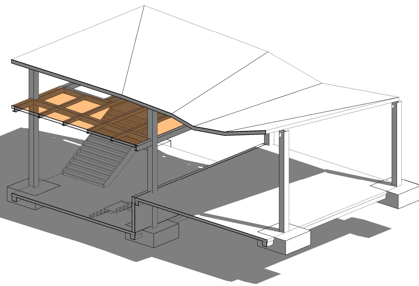
ISOMETRICO CORTE D-D
