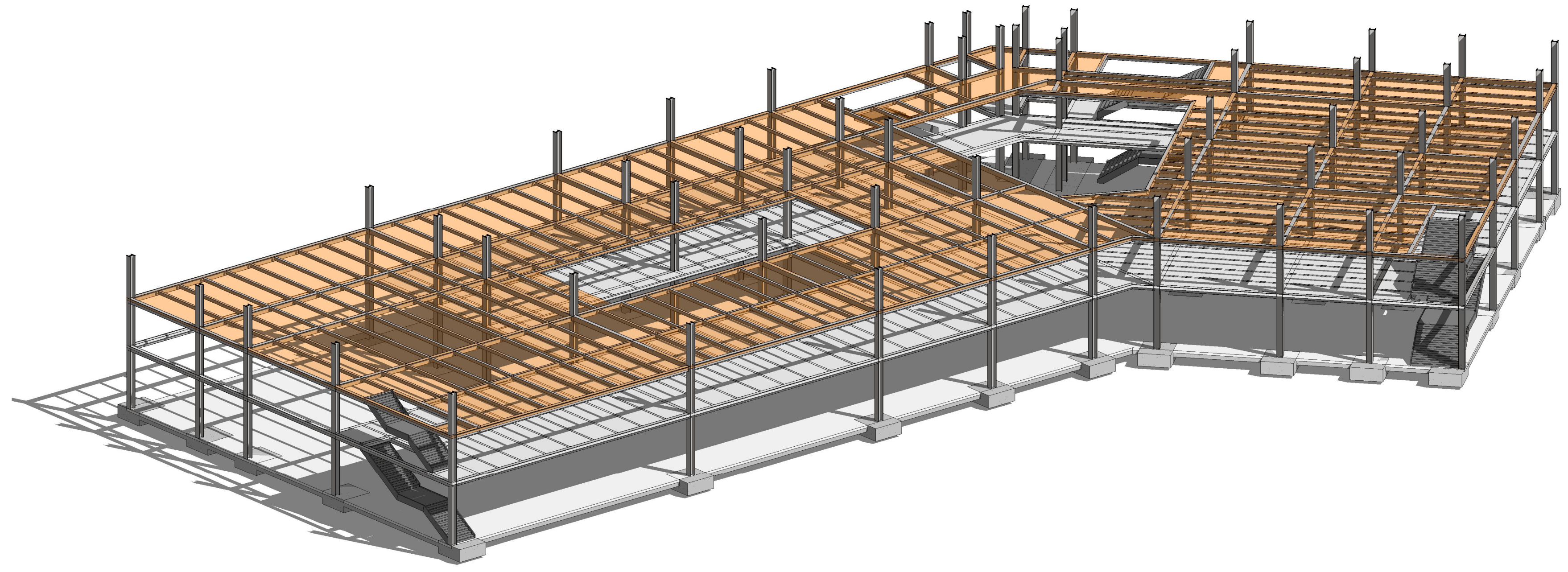
ISOMETRICO TERCER PISO
