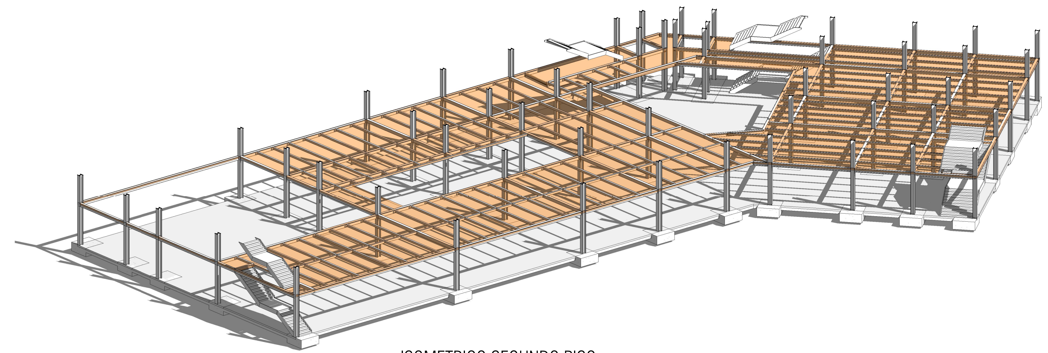
ISOMETRICO SEGUNDO PISO
