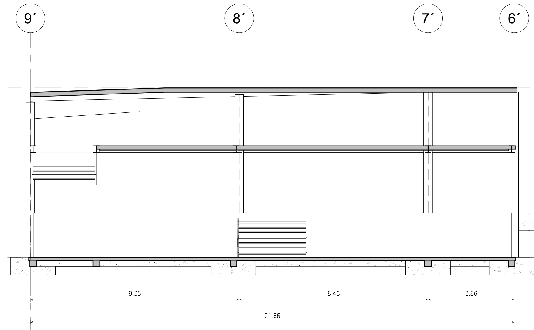
CORTE G-G 1 : 100
