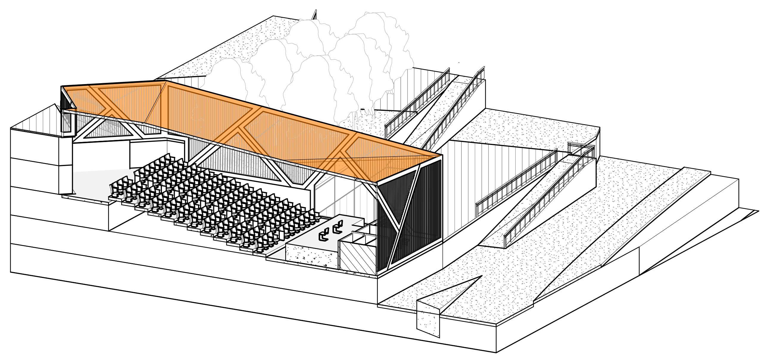
4 ISOMETRICO SECCIÓN G-G
