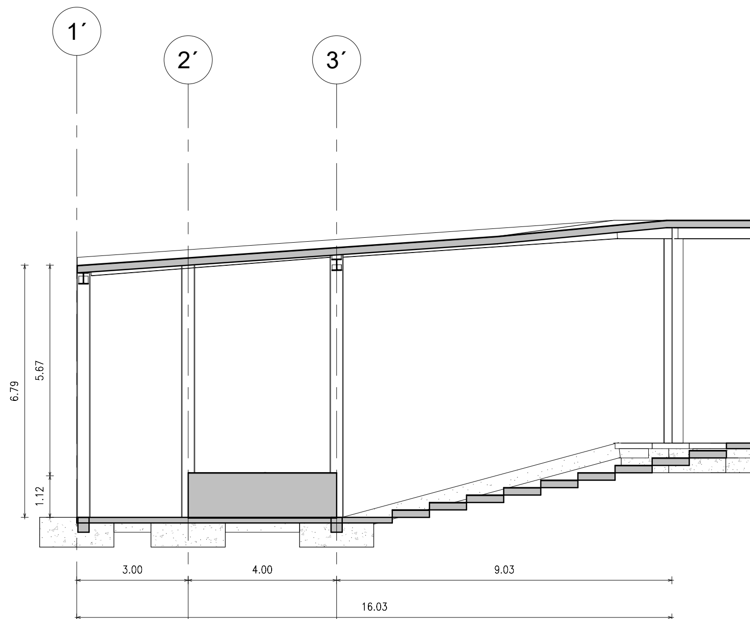
CORTE F-F 1 : 100
