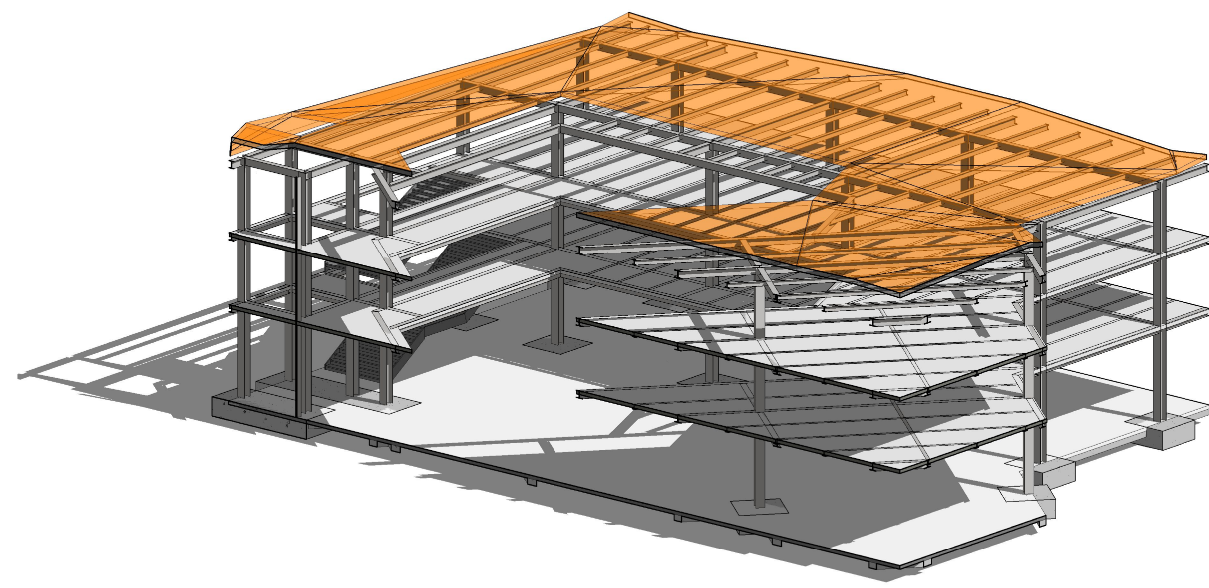
ISOMETRICO CORTE B-B
