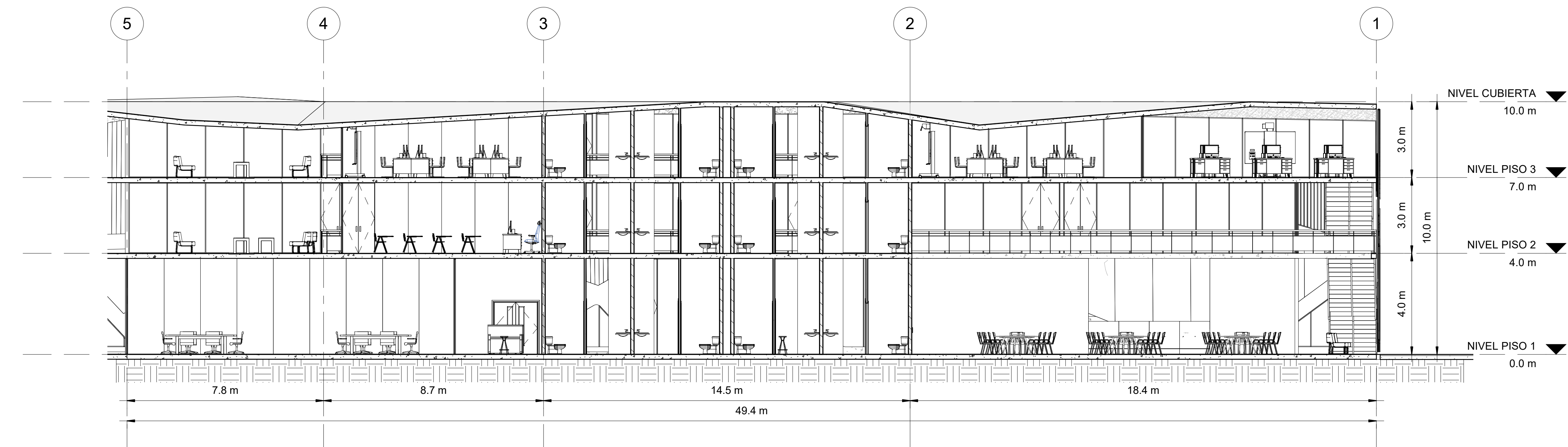
4 CORTE D-D 1 : 100
