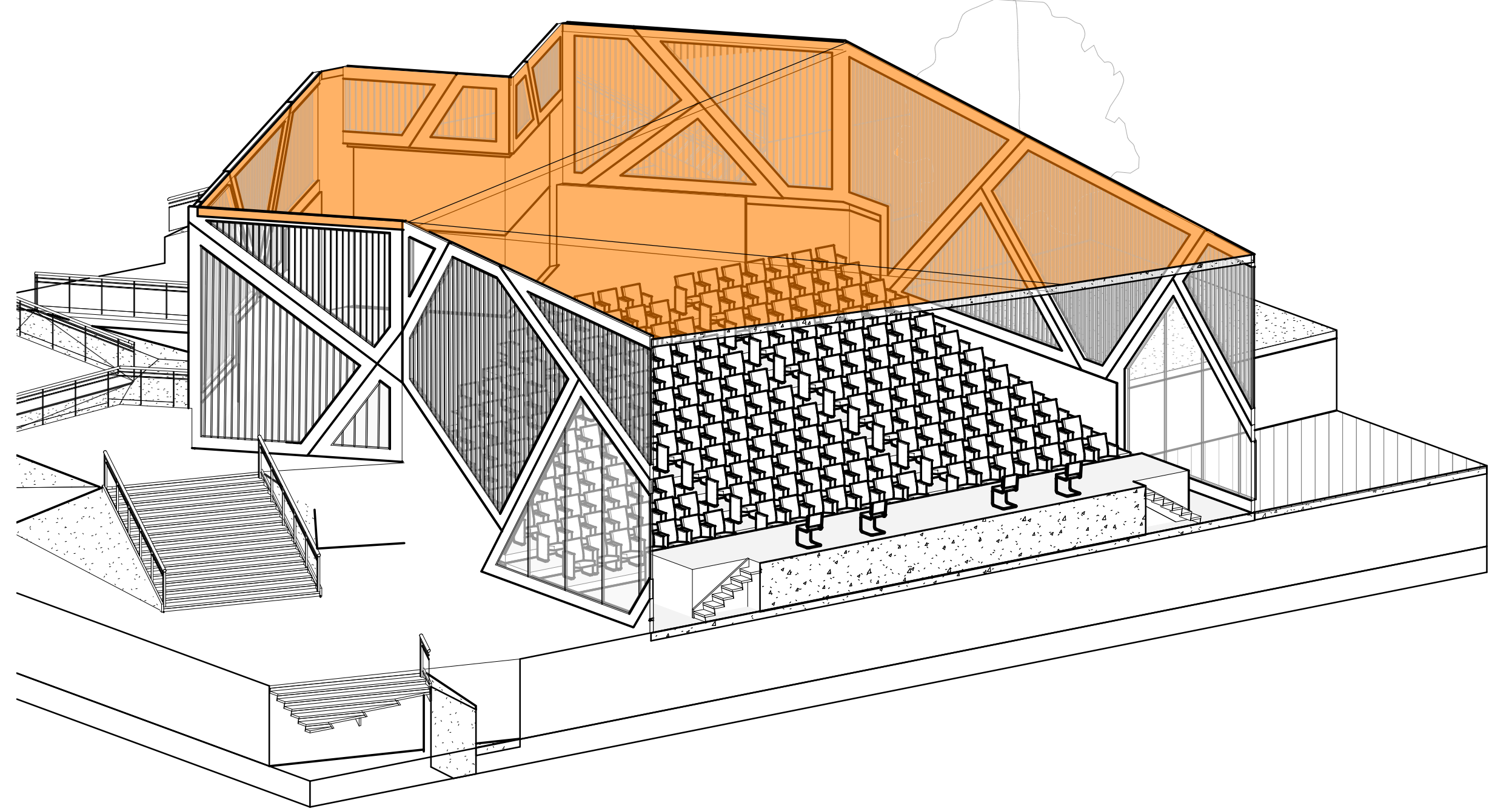
6 ISOMETRICO SECCIÓN H-H
