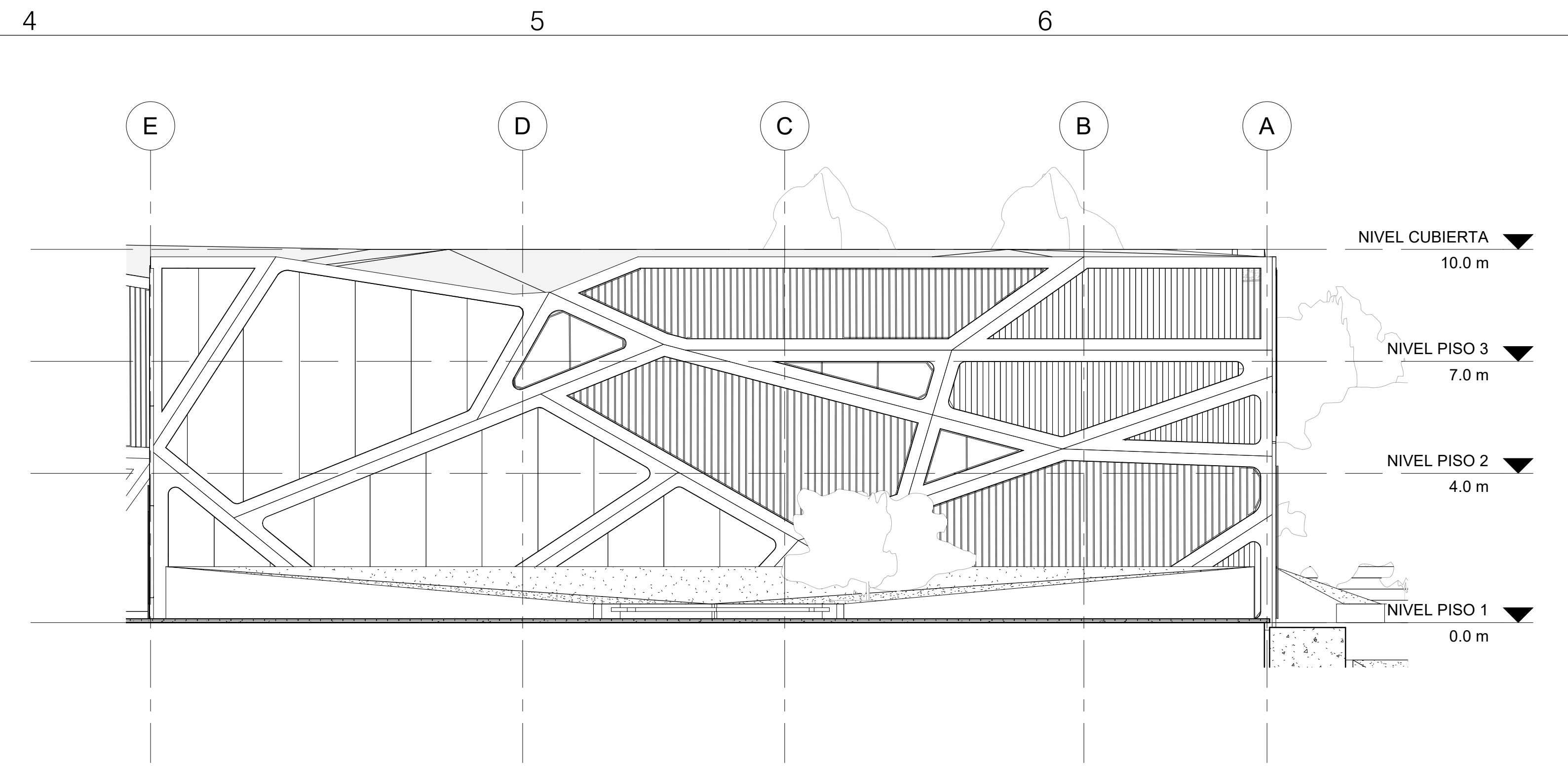
2 ALZADO SUR 1:100
