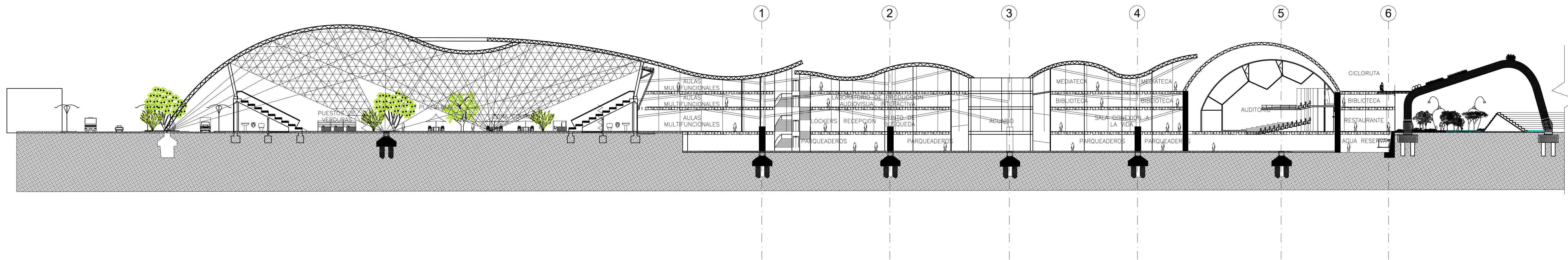
CORTE LONGITUDINAL B1
