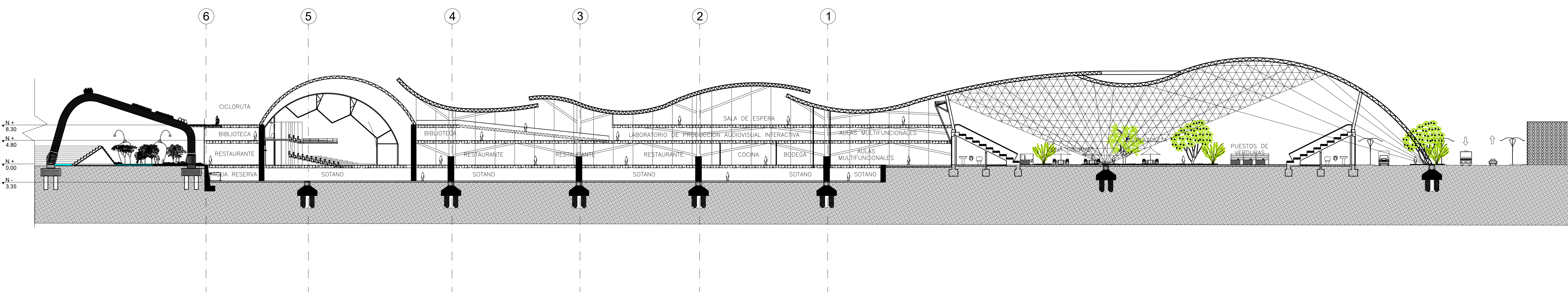
CORTE LONGITUDINAL B2
