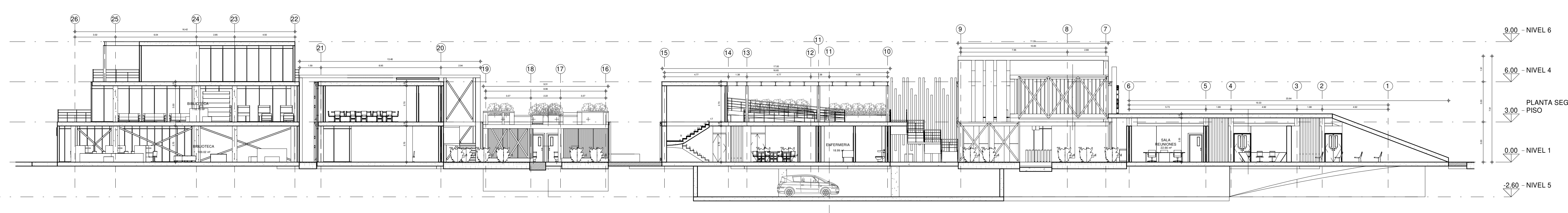
1 CORTE A-A 1:150
