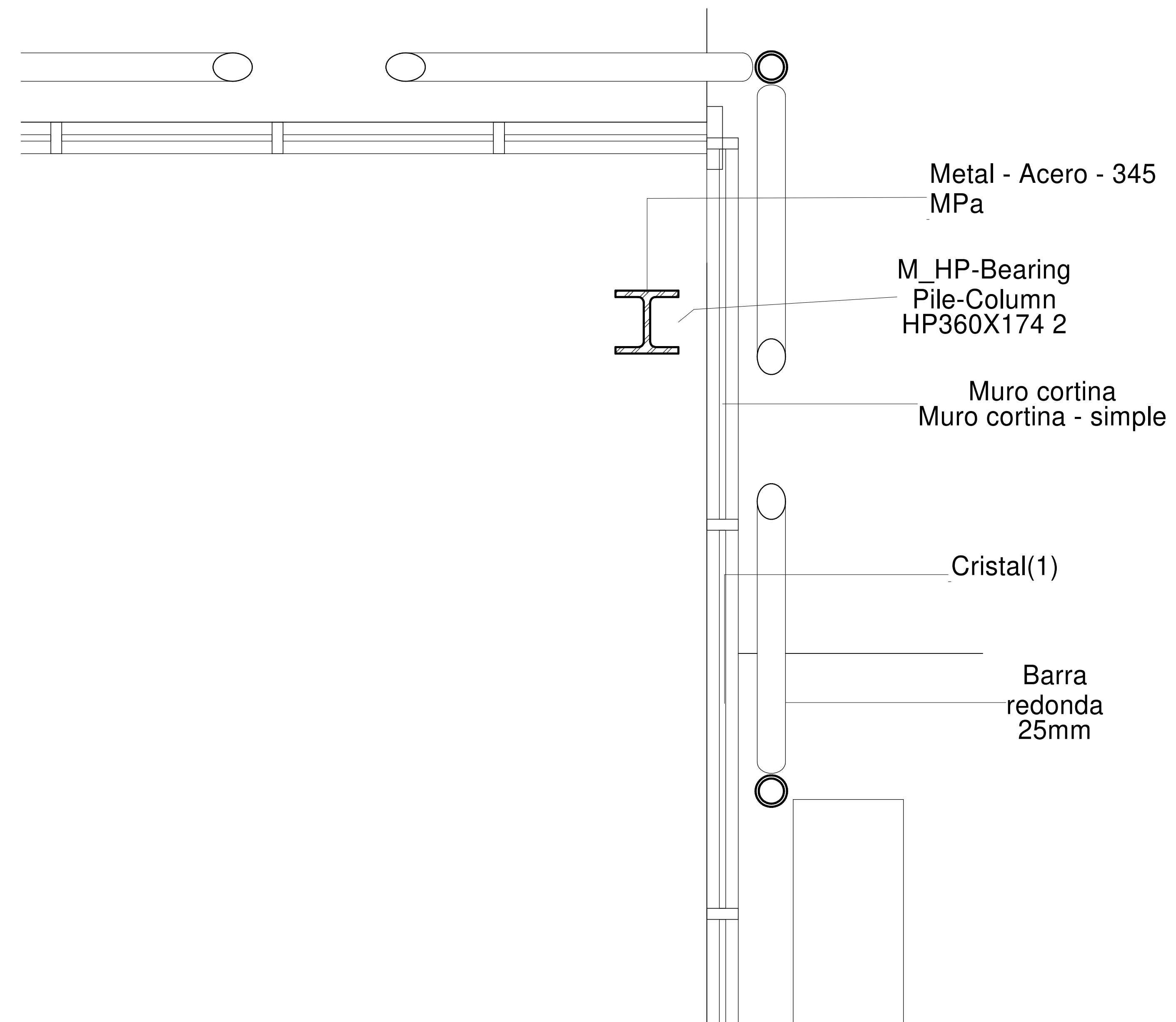
1 Detalle 3 1 : 10
