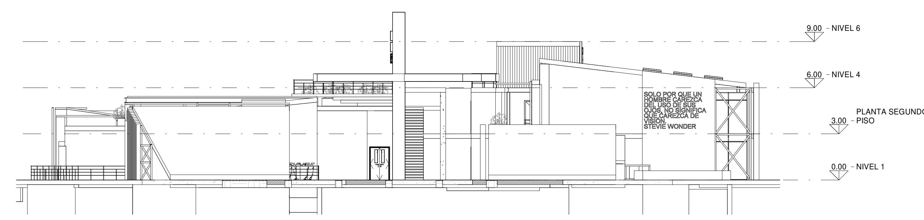
1 Este 1 : 150
