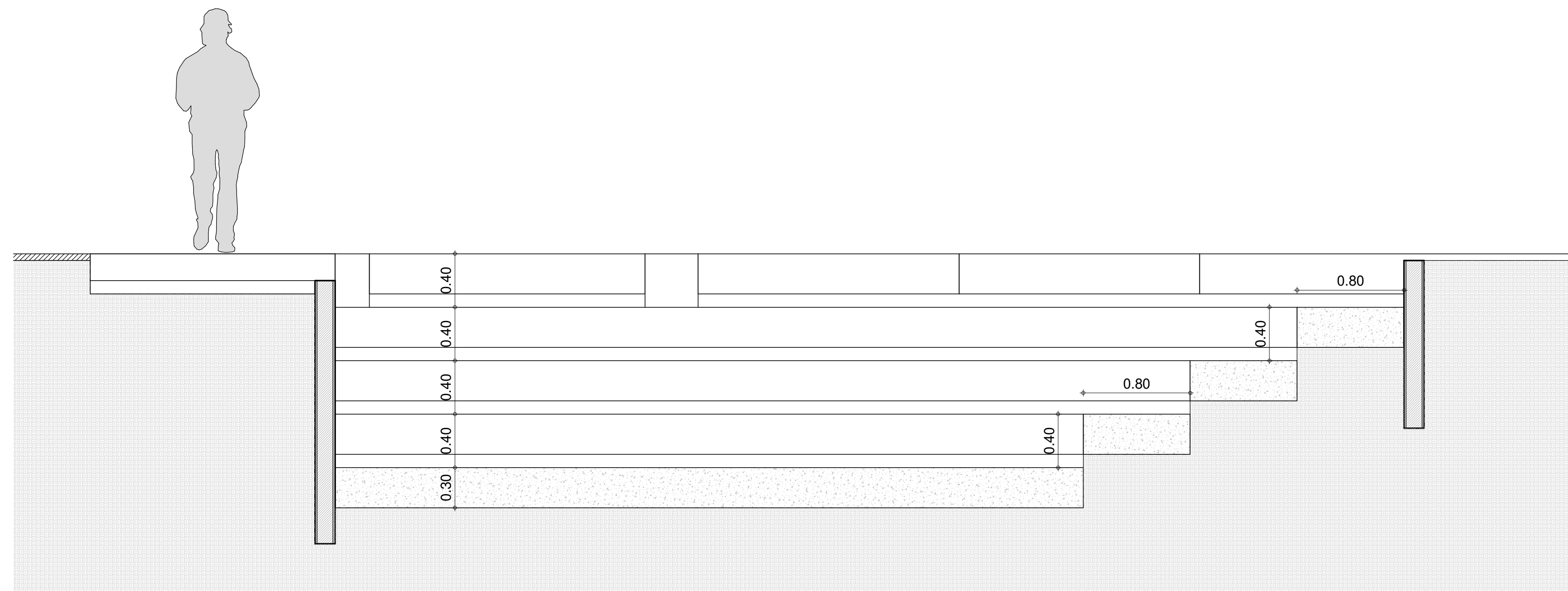
1 Detalle 9 1 : 50
