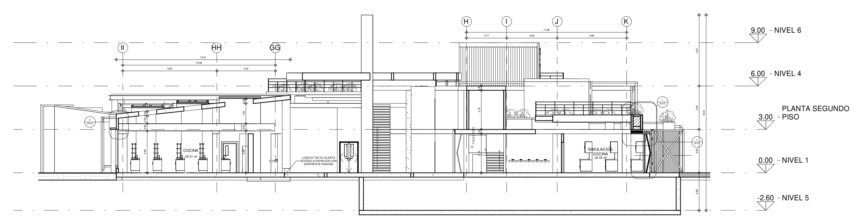
2 CORTE B-B 1:150
