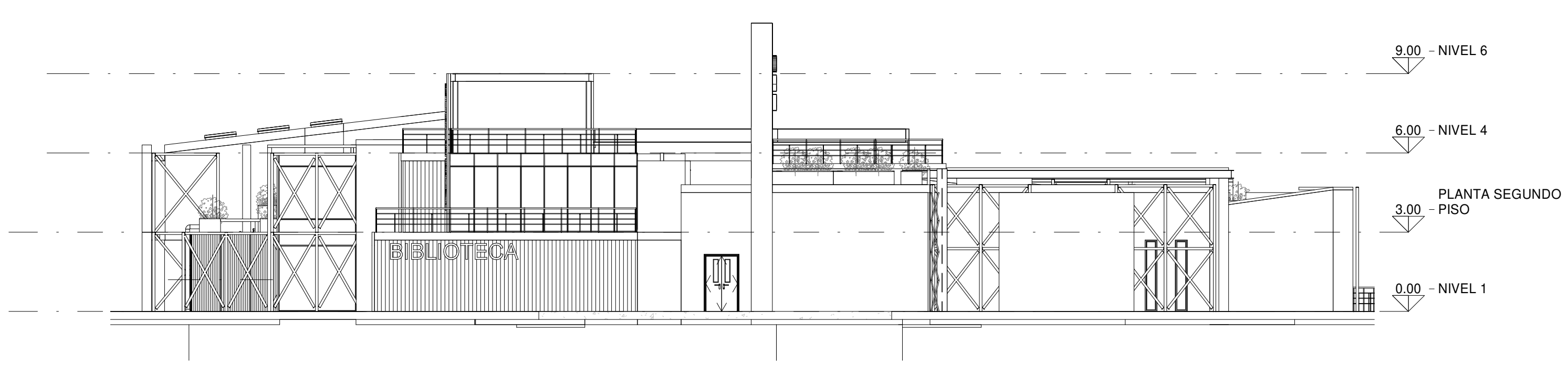
2 Oeste 1 : 150
