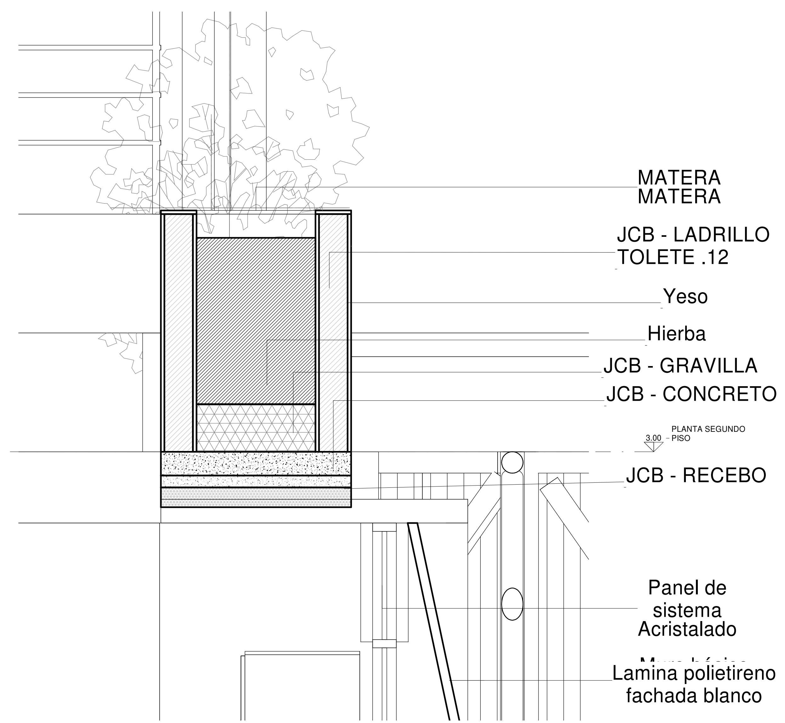
1 DETALLE MATERAS 1 : 10
