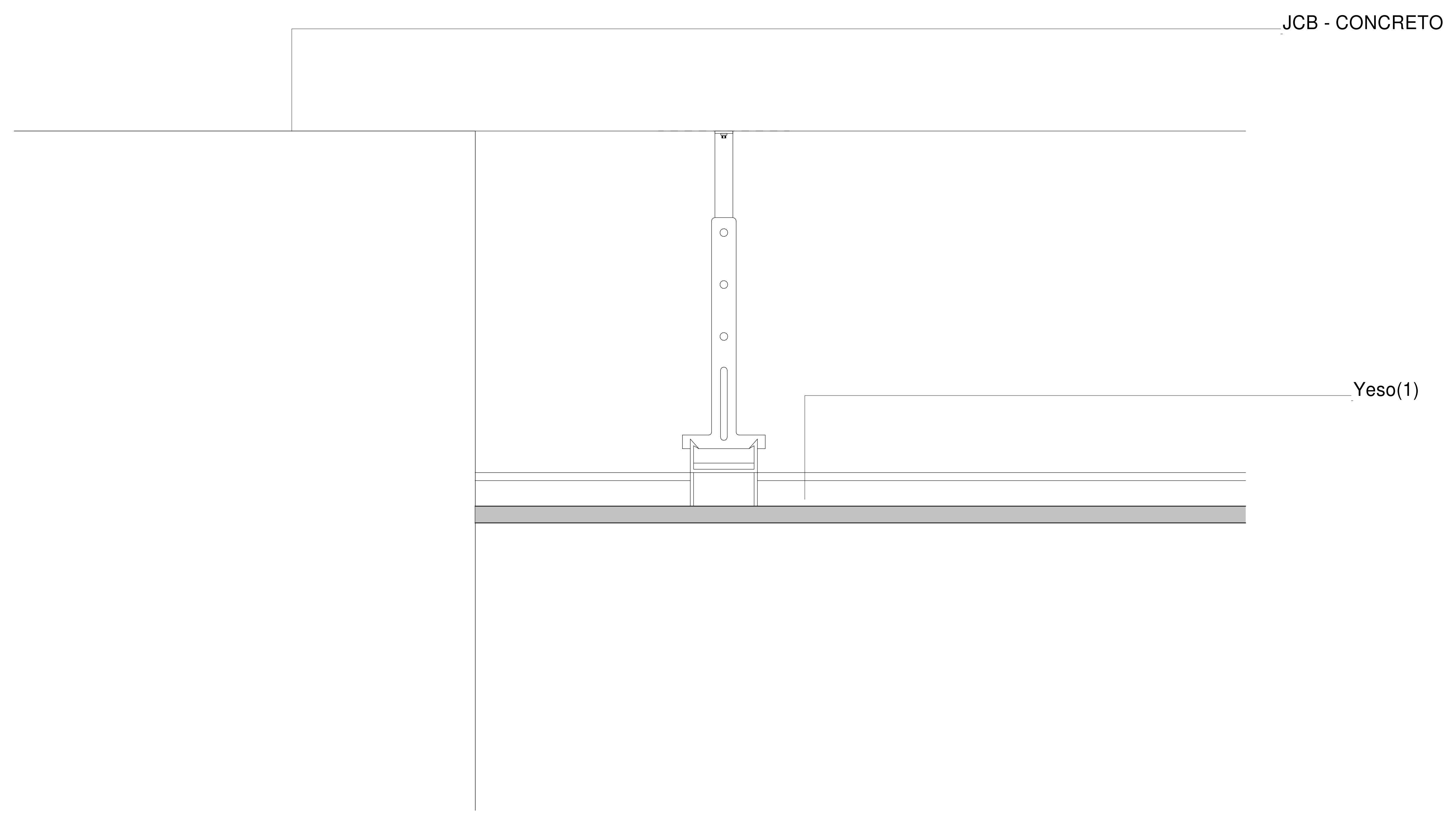
① DETALLE CIELO FALSO 1:2
