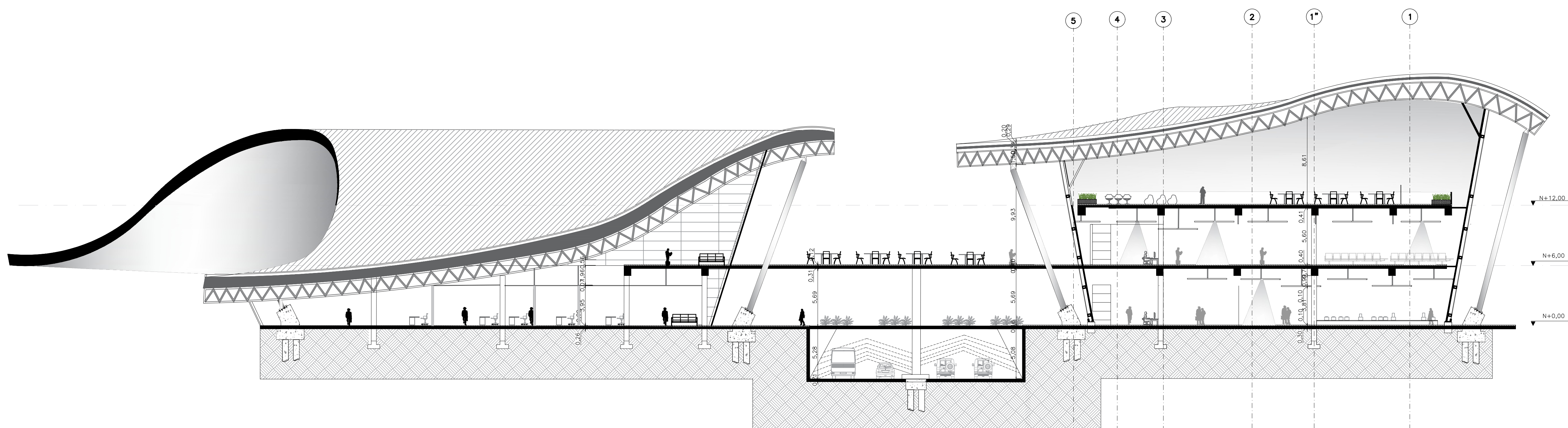
AA CORTE A-A ESCALA 1:250 ESCALA A 1:250
