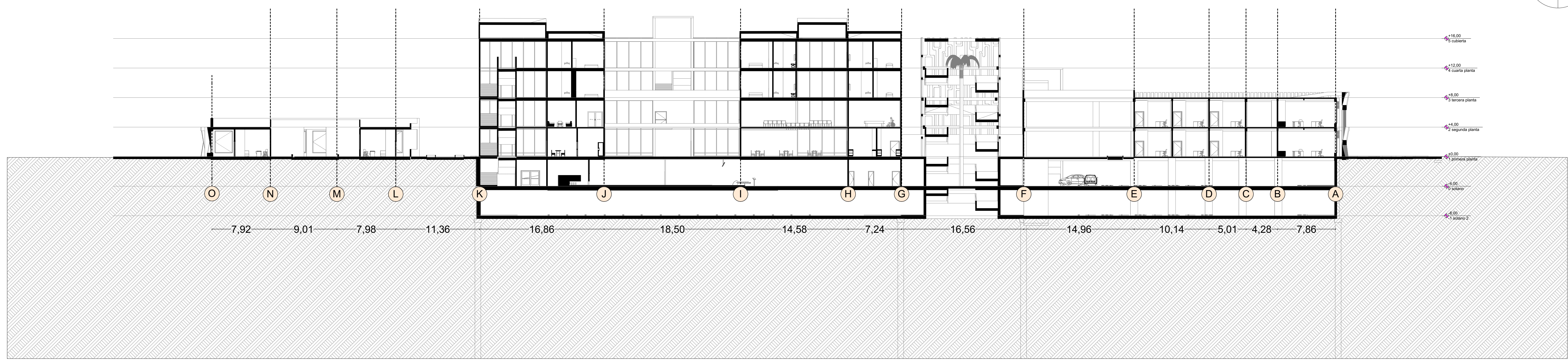
S-08 Seccion Modulo Bienestar Esc 1:250
