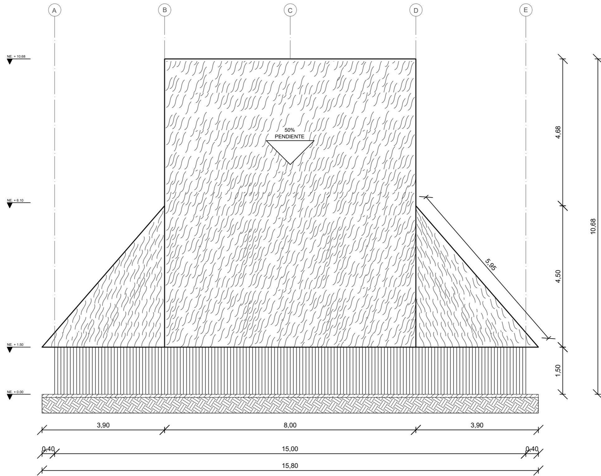
FACHADA LATERAL EJE 6 ESCALA: 1:75
