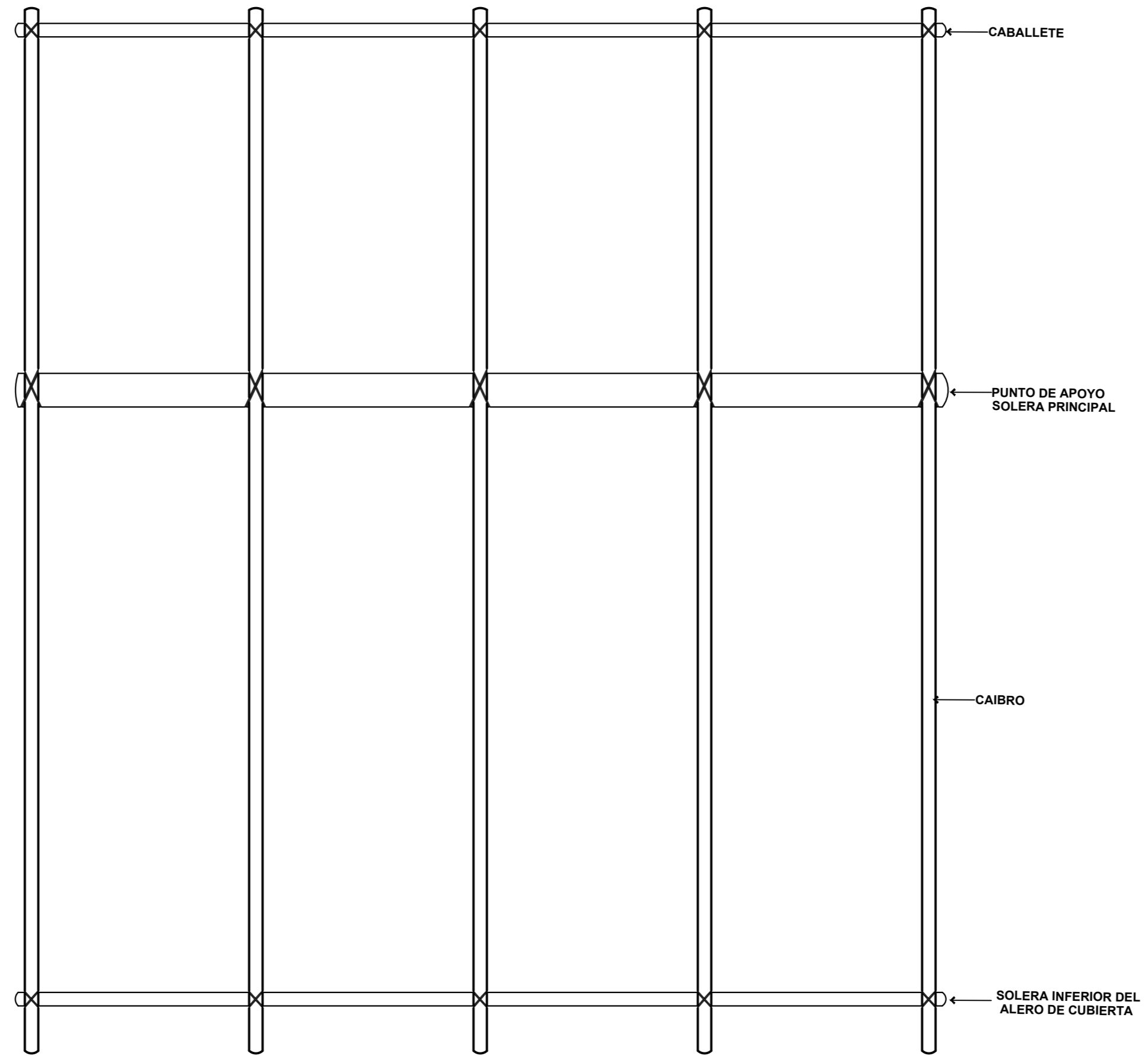
DETALLE PARTE DE ESTRUCTURA DE CUBIERTA ENTRE EJES B Y D ESCALA: 1:40
