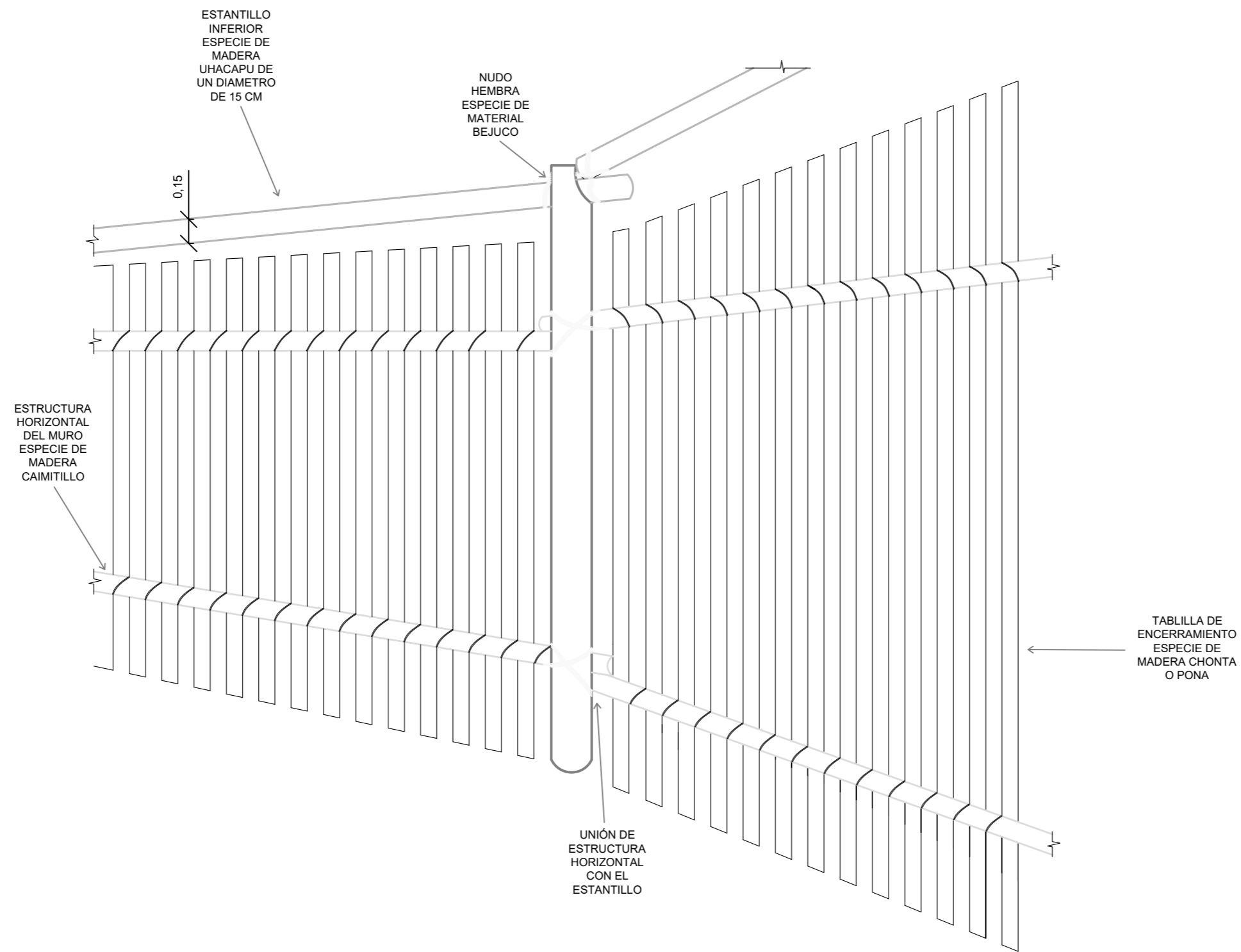
DETALLE DE MURO ESCALA: 1:30
