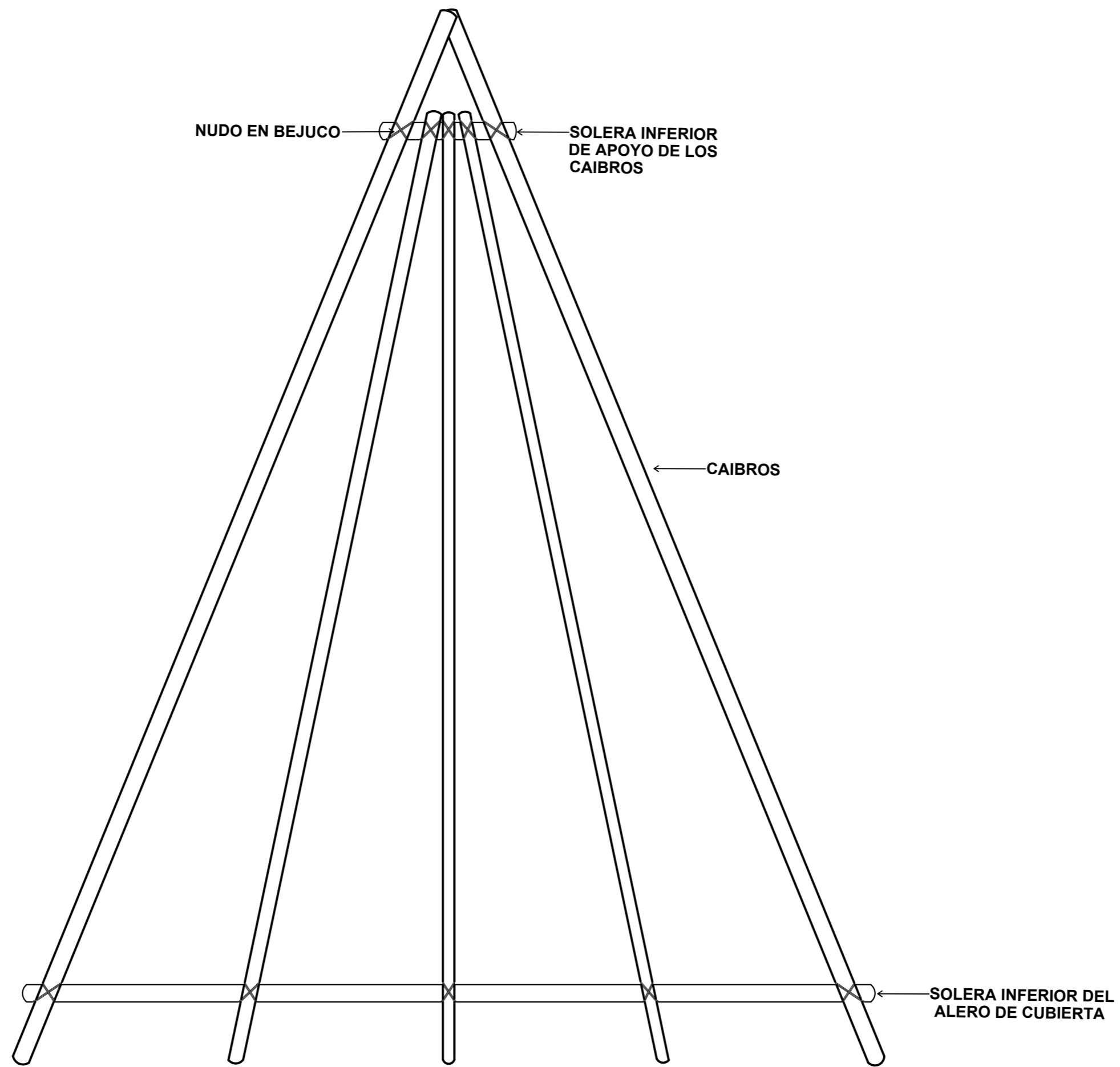
DETALLE PARTE DE ESTRUCTURA DE CUBIERTA VISTA DE ARRIBA ENTRE EJES 2 Y B ESCALA: 1:30
