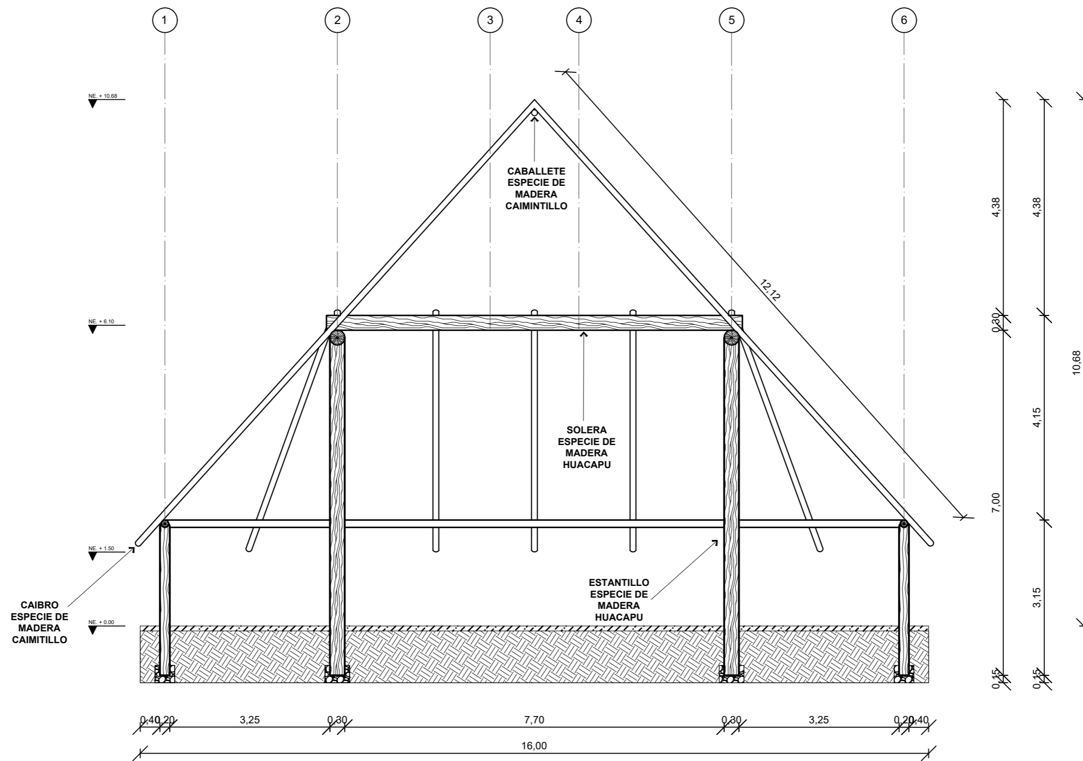
CORTE DE ESTRUCTURA DE MALOCA EJE C ESCALA: 1:75
