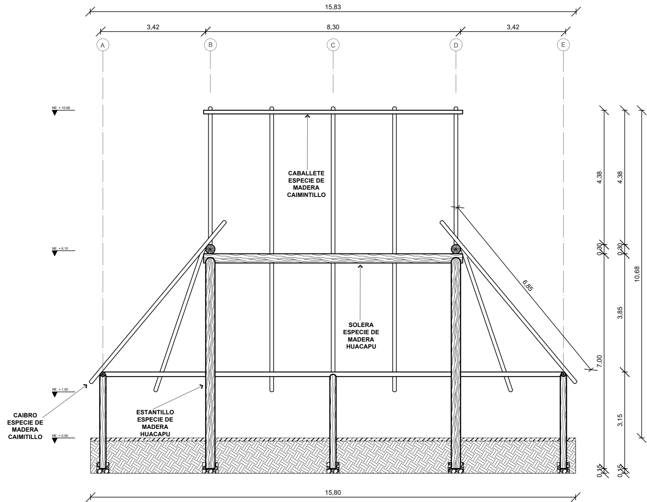
CORTE DE ESTRUCTURA DE MALOCA EJE 4 ESCALA: 1:75
