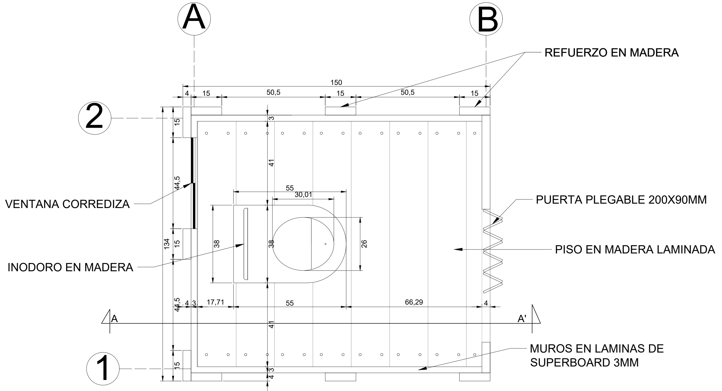
PLANTA ARQUITECTONICA DEL BAÑO
