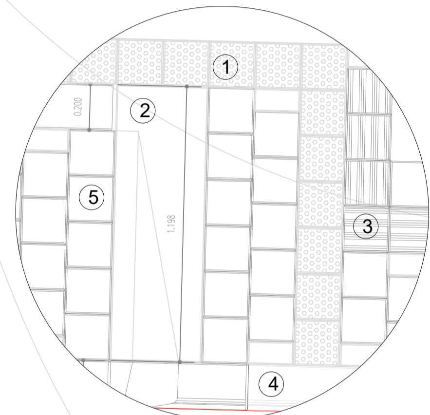
DETALLE CONSTRUCTIVO ANDEN
