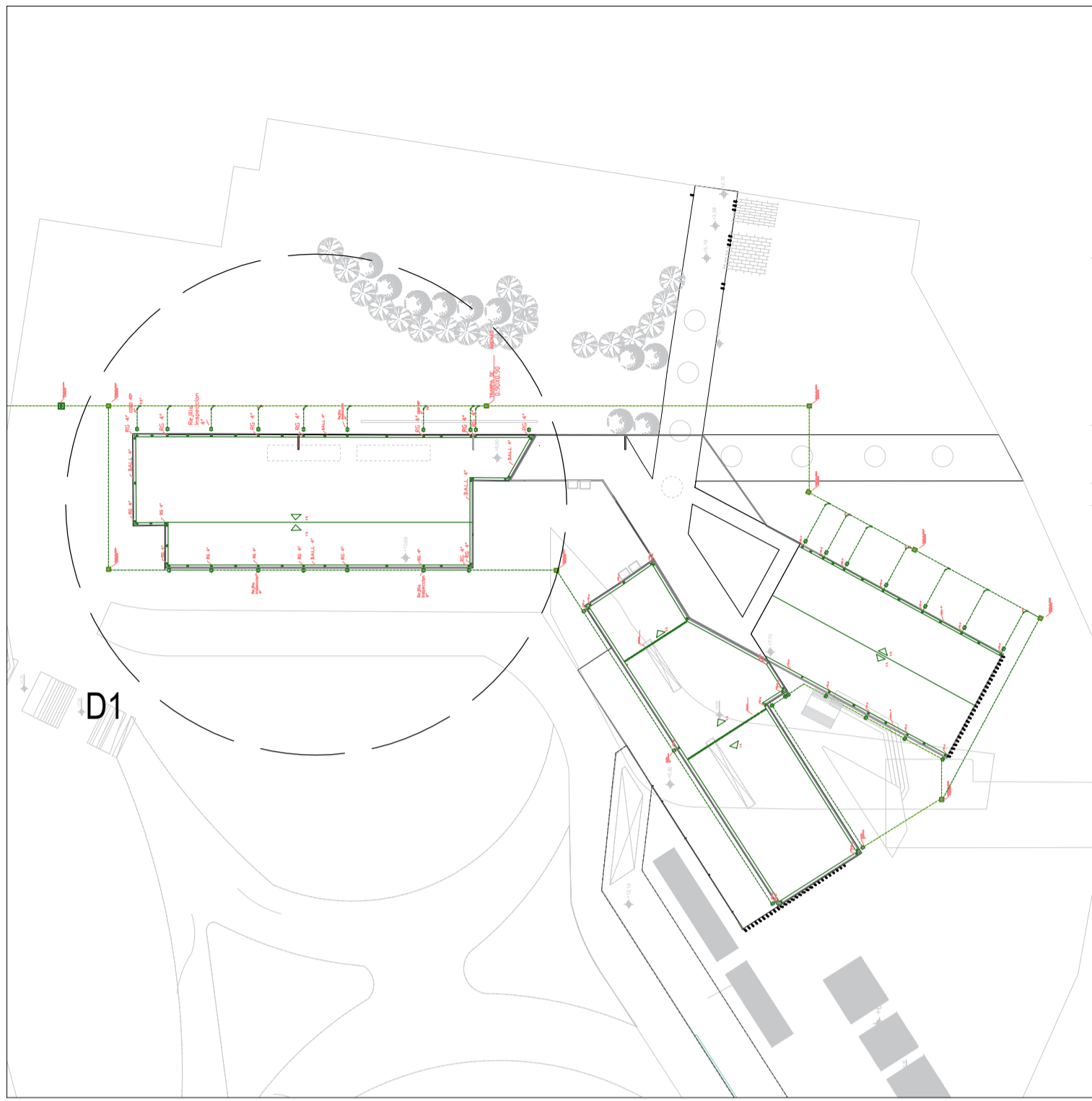
A RED DE AGUAS LLUVIAS ESC. 1:1250
