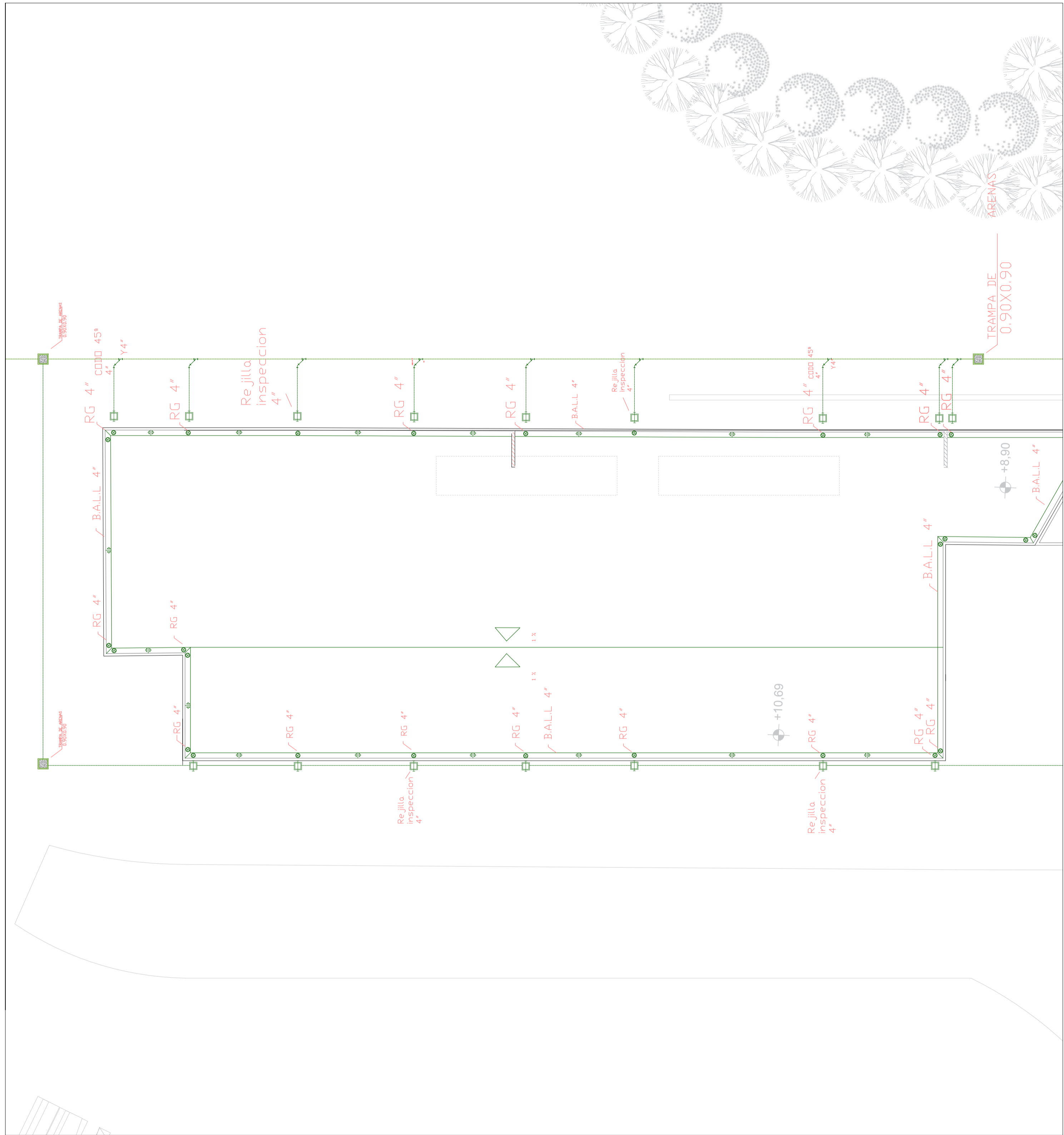
D1 DETALLE RED DE AGUAS LLUVIAS ESC. 1:250
