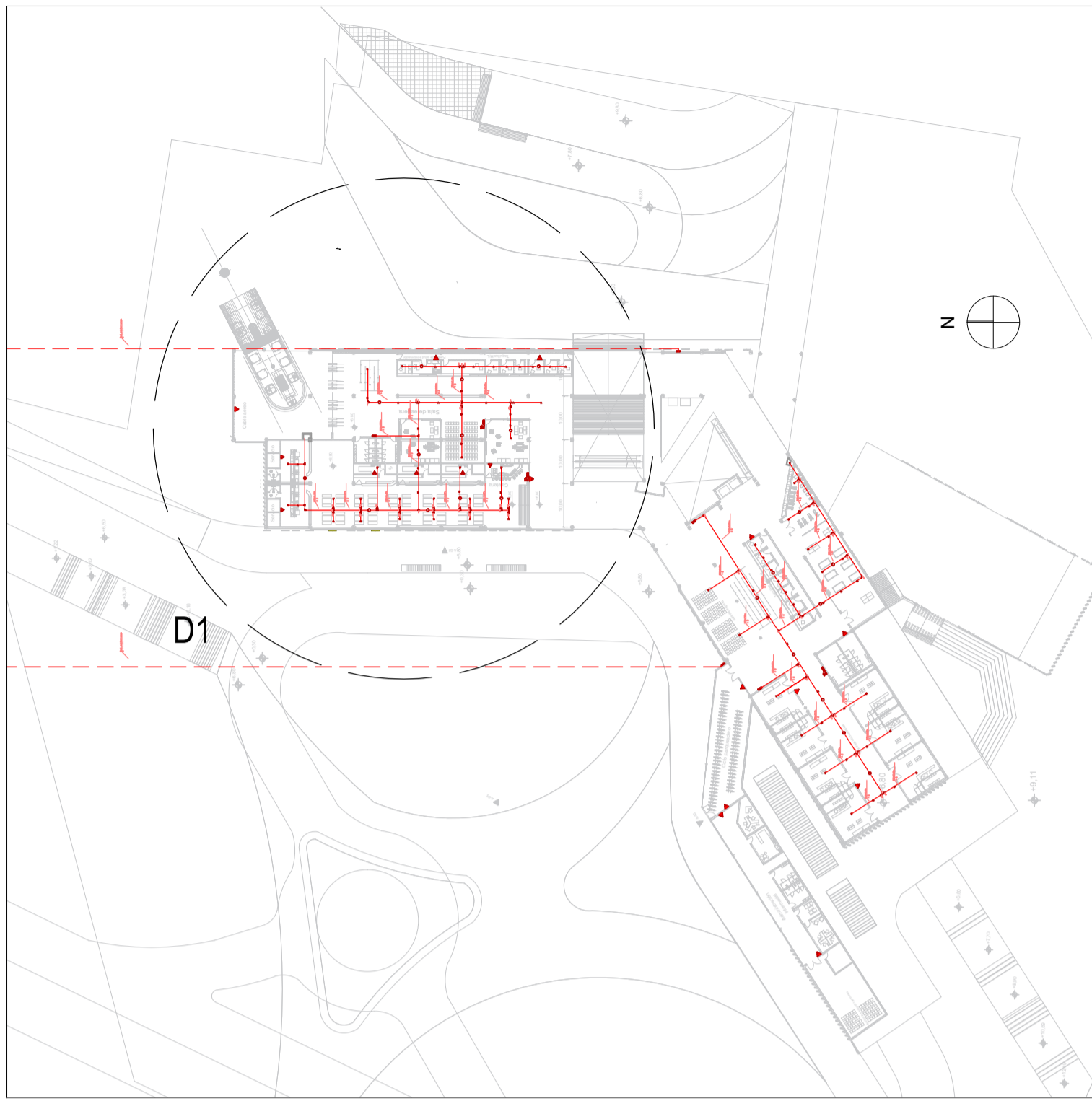
A RED CONTRA INCENDIO ESC. 1:1250
