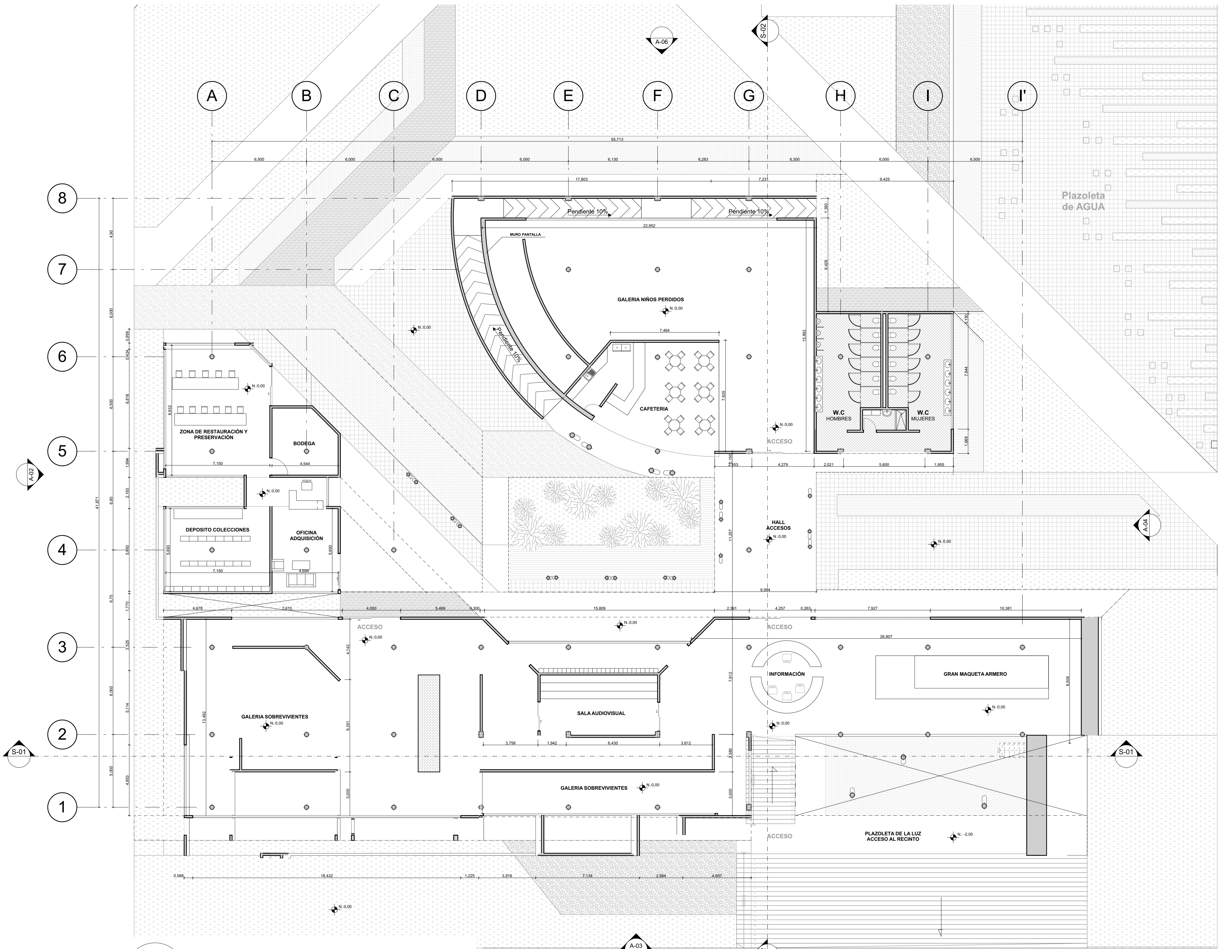
A-008 PLANTA ARQUITECTONICA Z. MUSEO 1ER PISO ESCALA 1:150
