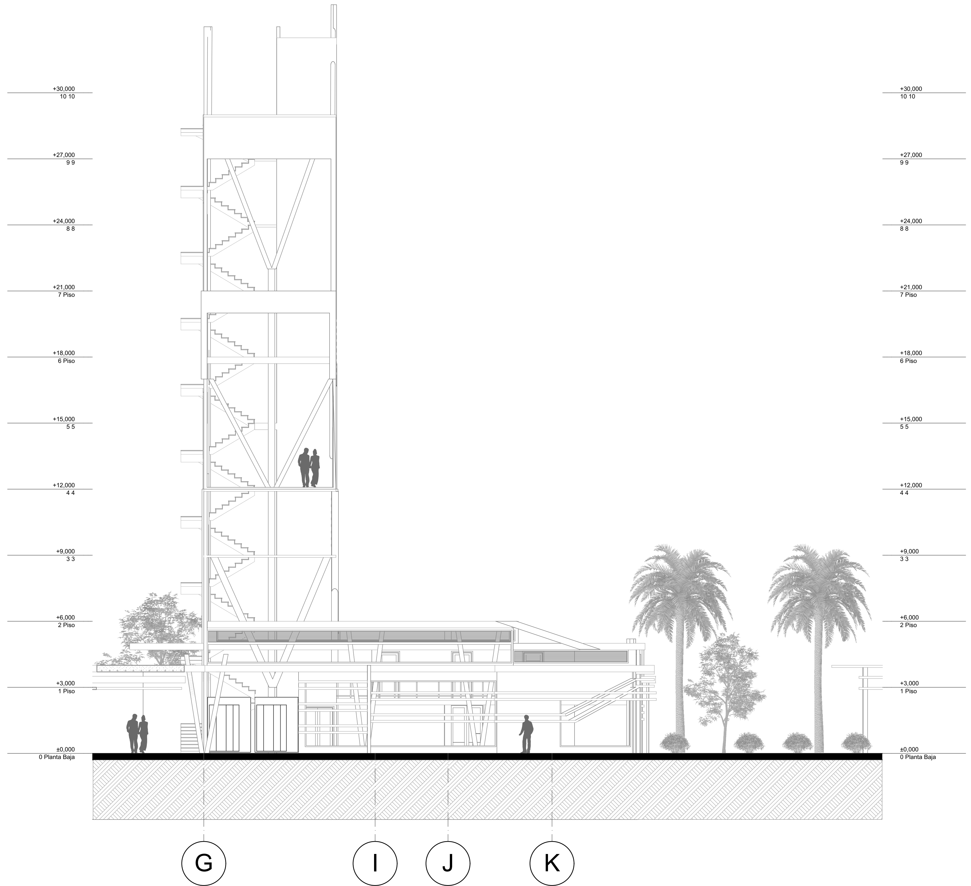
F-002 FACHADA 02 ADMIN-MIRADOR ESCALA 1:100
