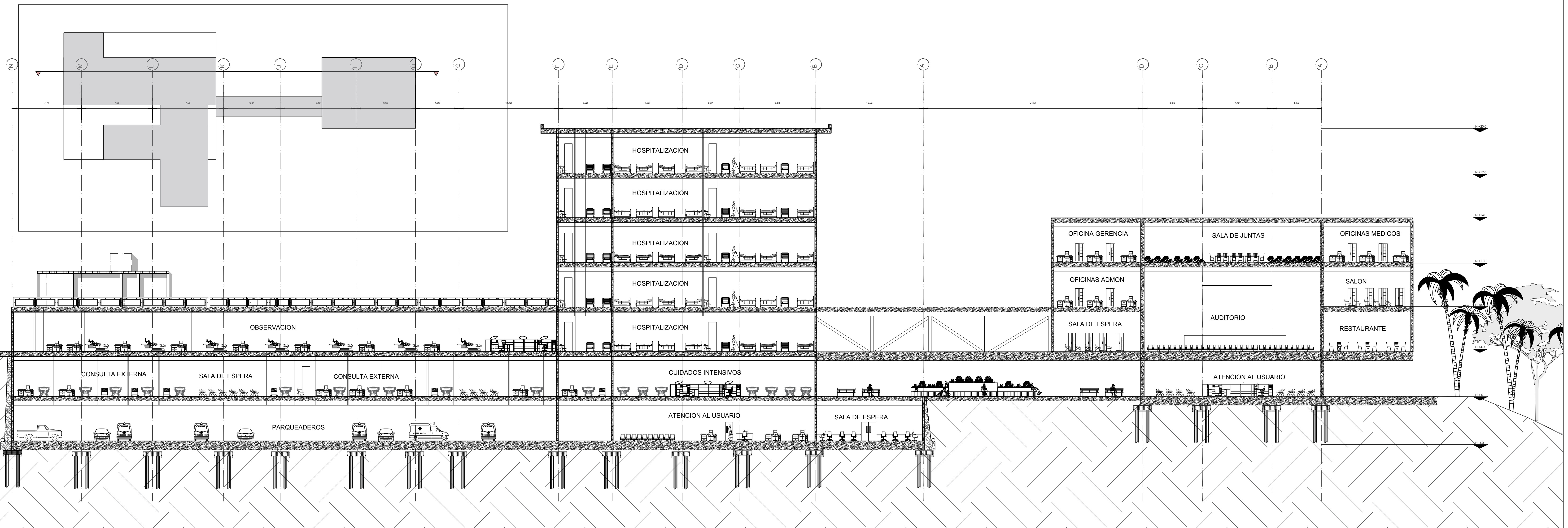
A09 Corte C-C ESCALA 1:200
