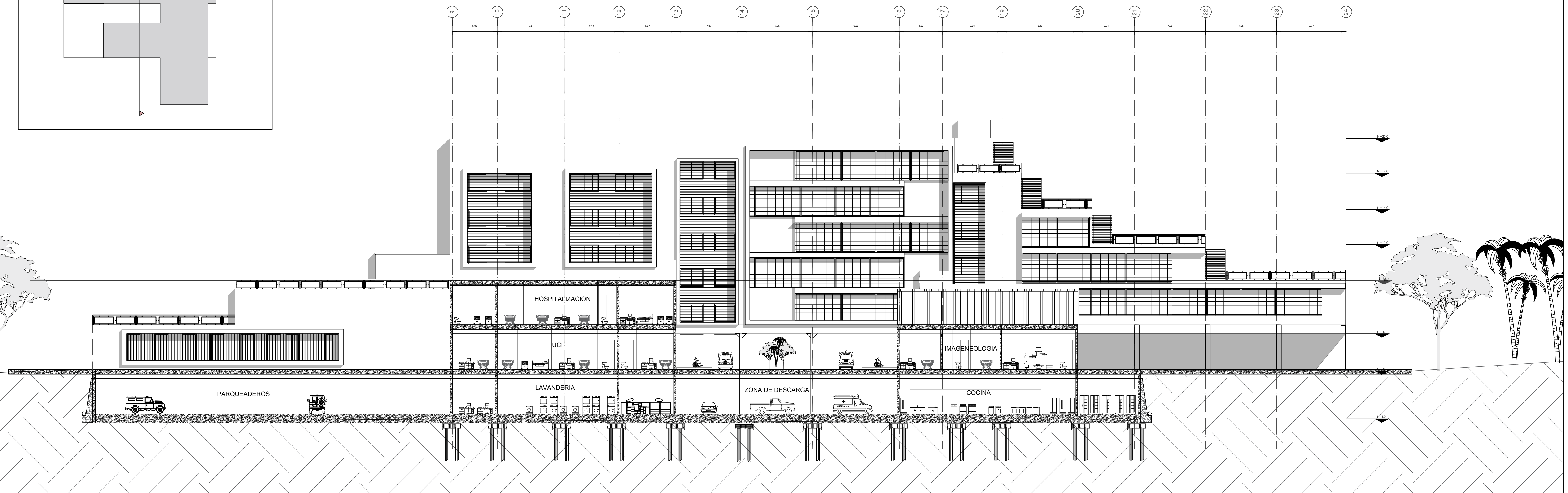
A09 Corte D-D ESCALA 1:200
