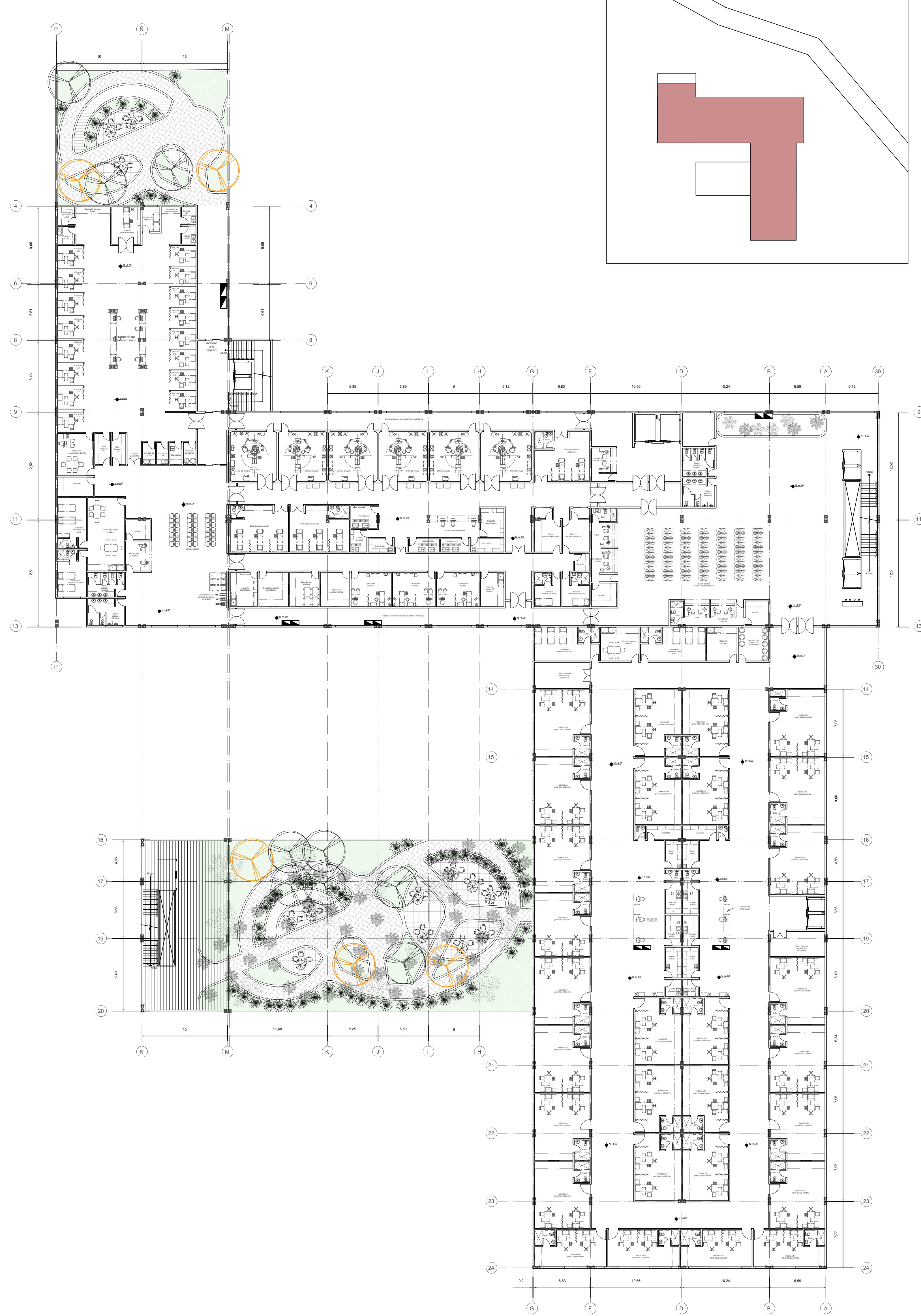
A04 Planta Segundo nivel ESCALA 1:250
