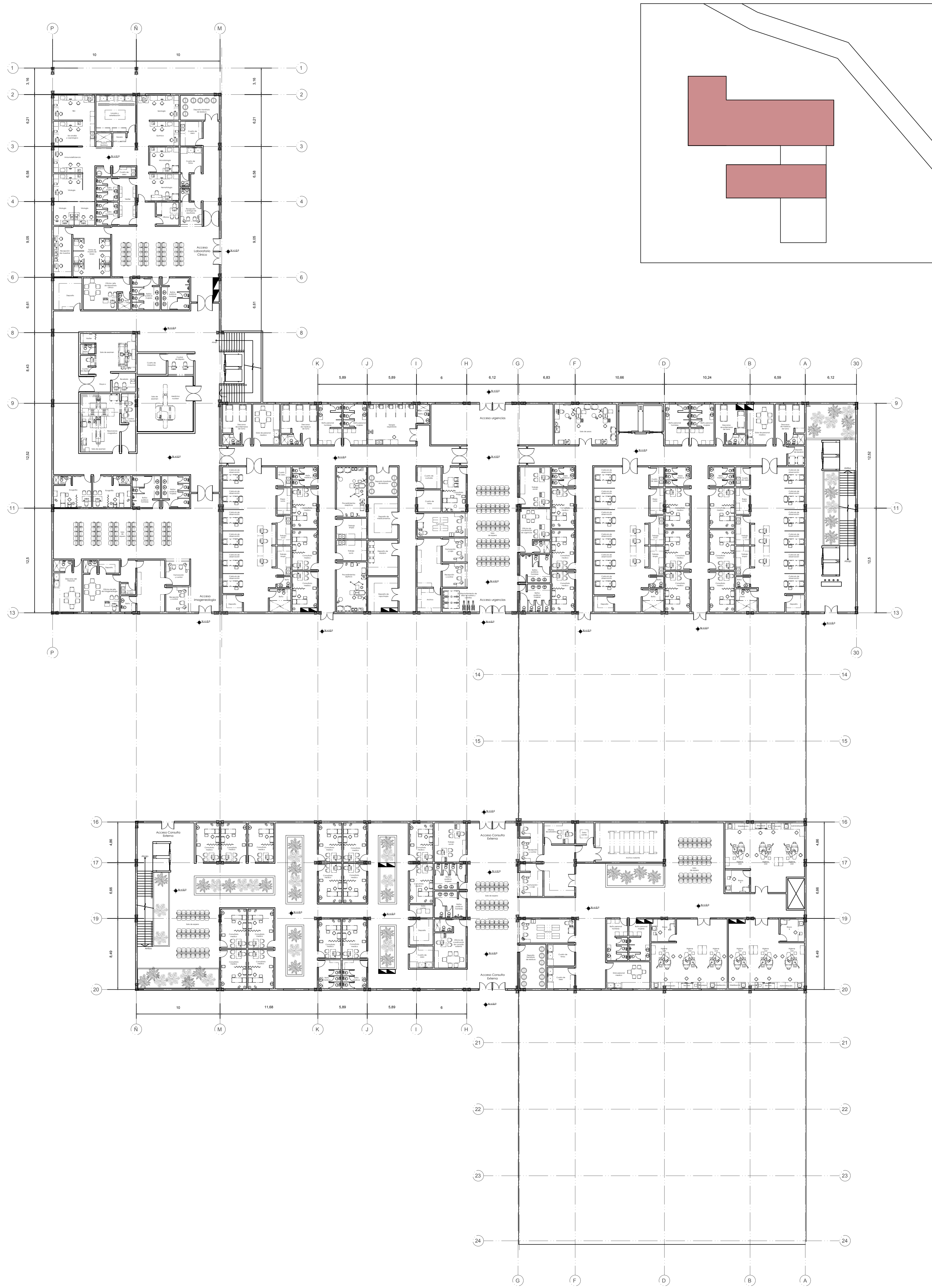
A04 Planta Primer nivel ESCALA 1:250
