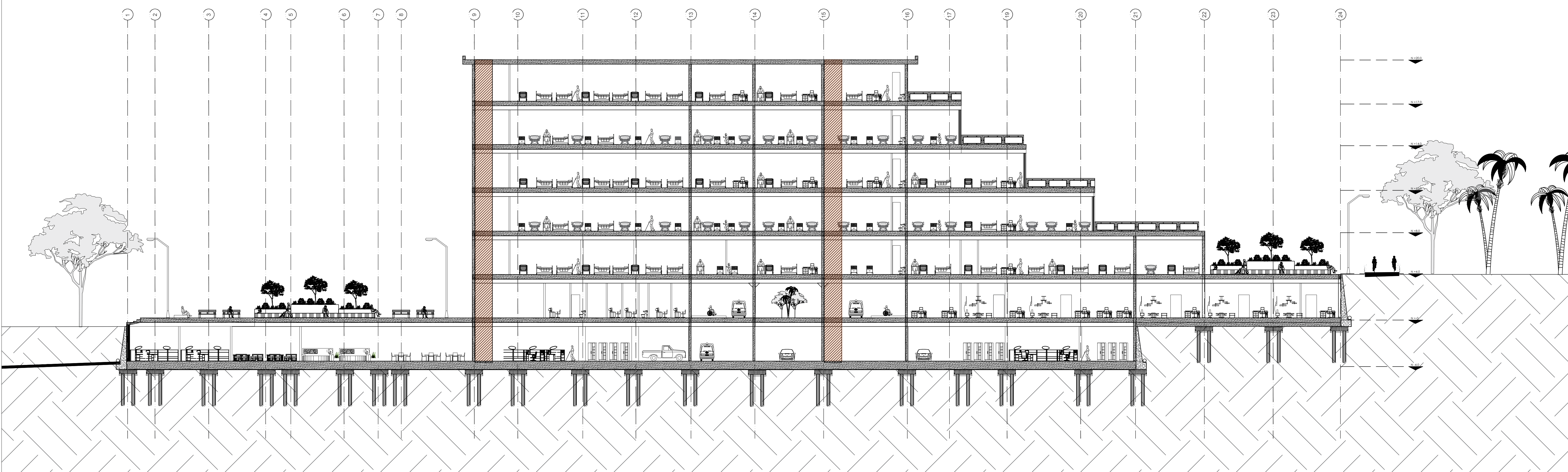
A29 Localizacion ductos de instalaciones corte longitudinal ESCALA 1:200
