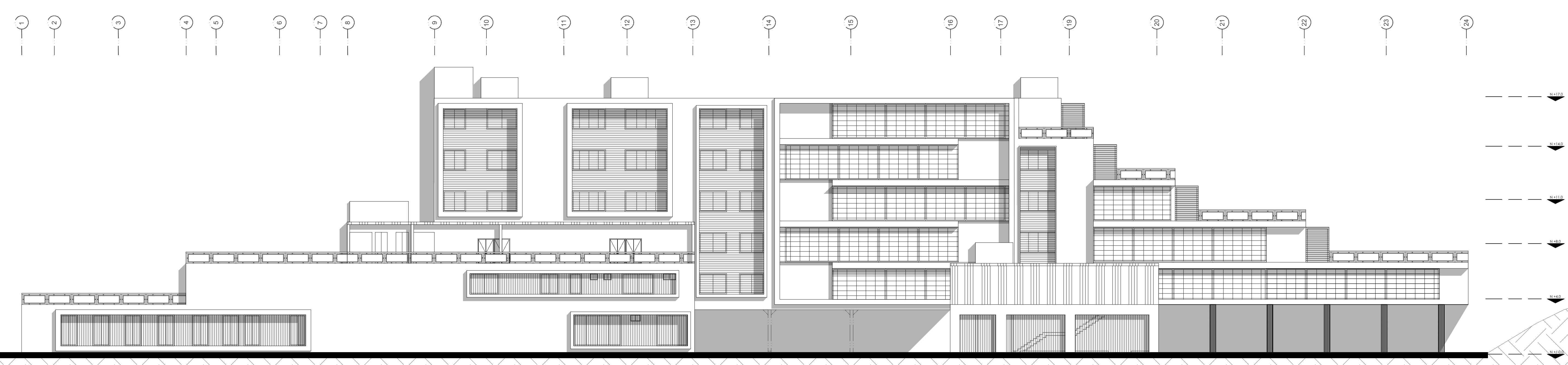
A11 Fachada Occidental ESCALA 1:200
