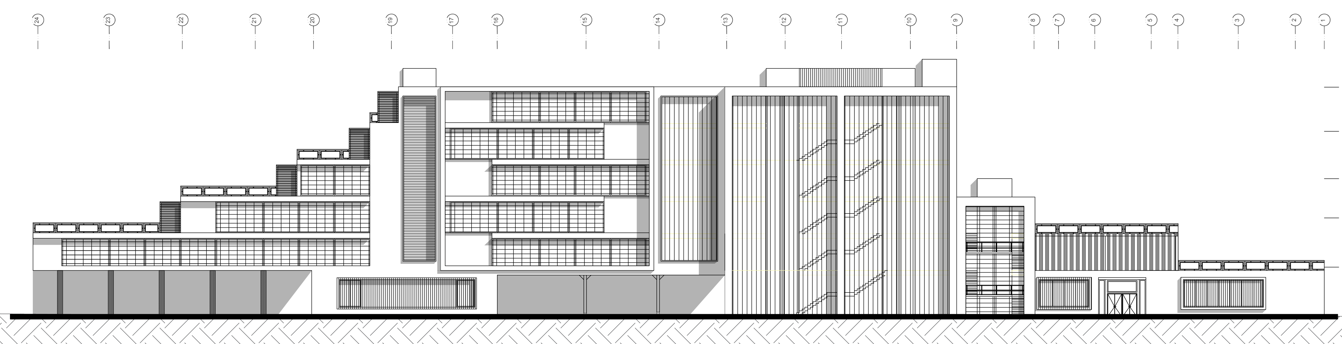
A12 Fachada Oriental ESCALA 1:200
