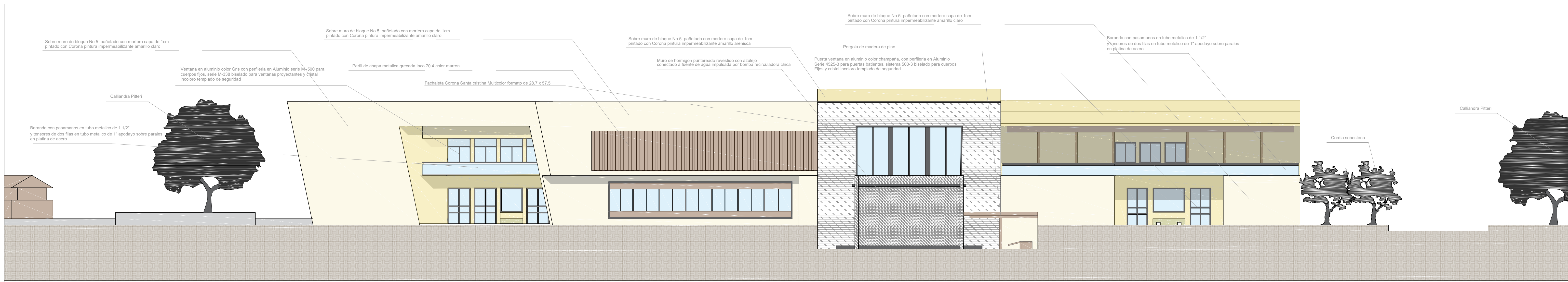
A FACHADA 1 Escala 1:50
