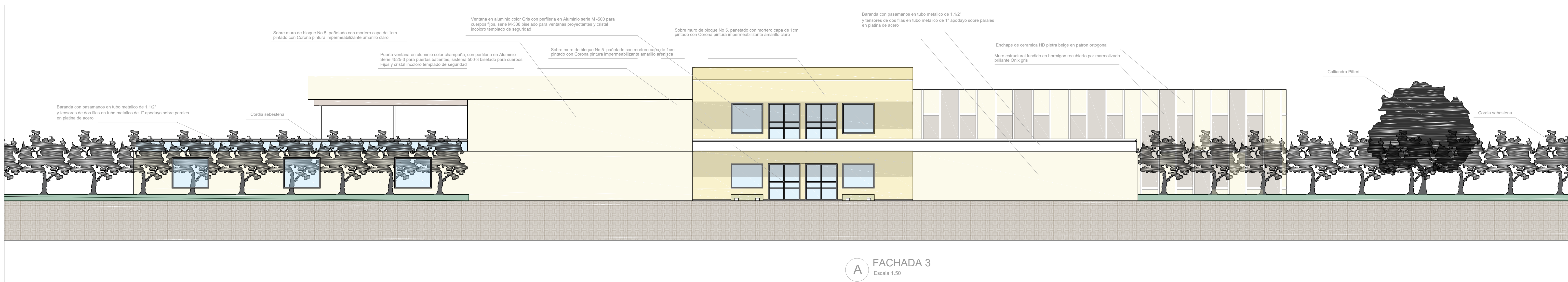
A FACHADA 2 Escala 1:50
