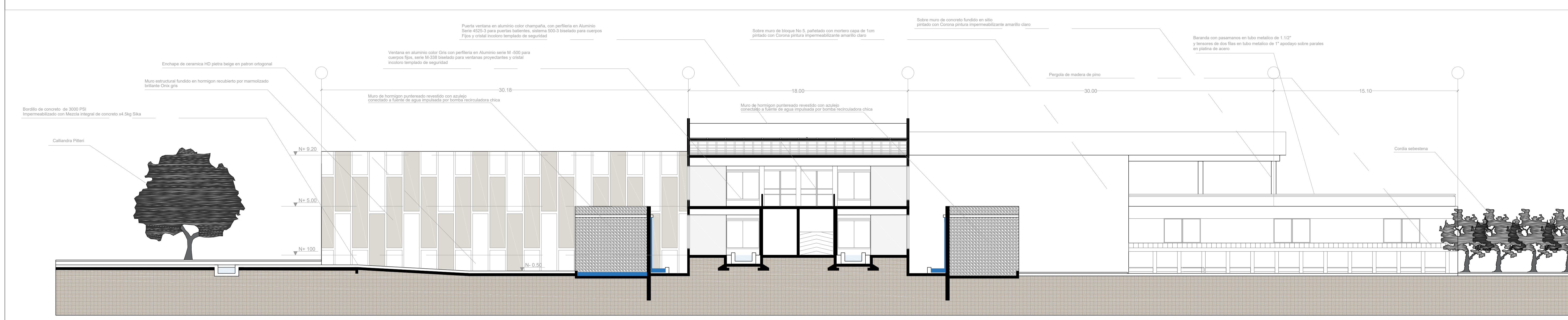
A CORTE C2 Escala 1:50
