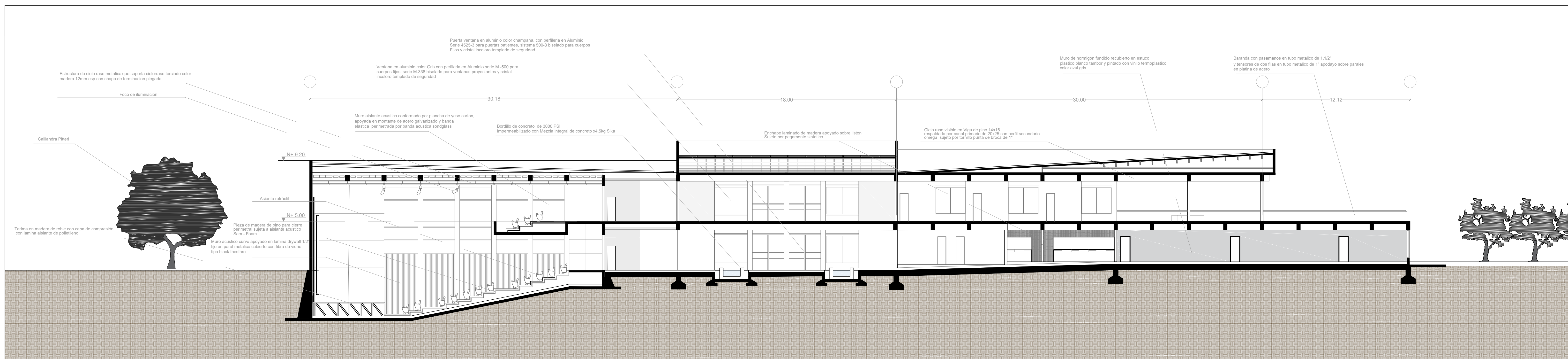
A CORTE C1 Escala 1:50
