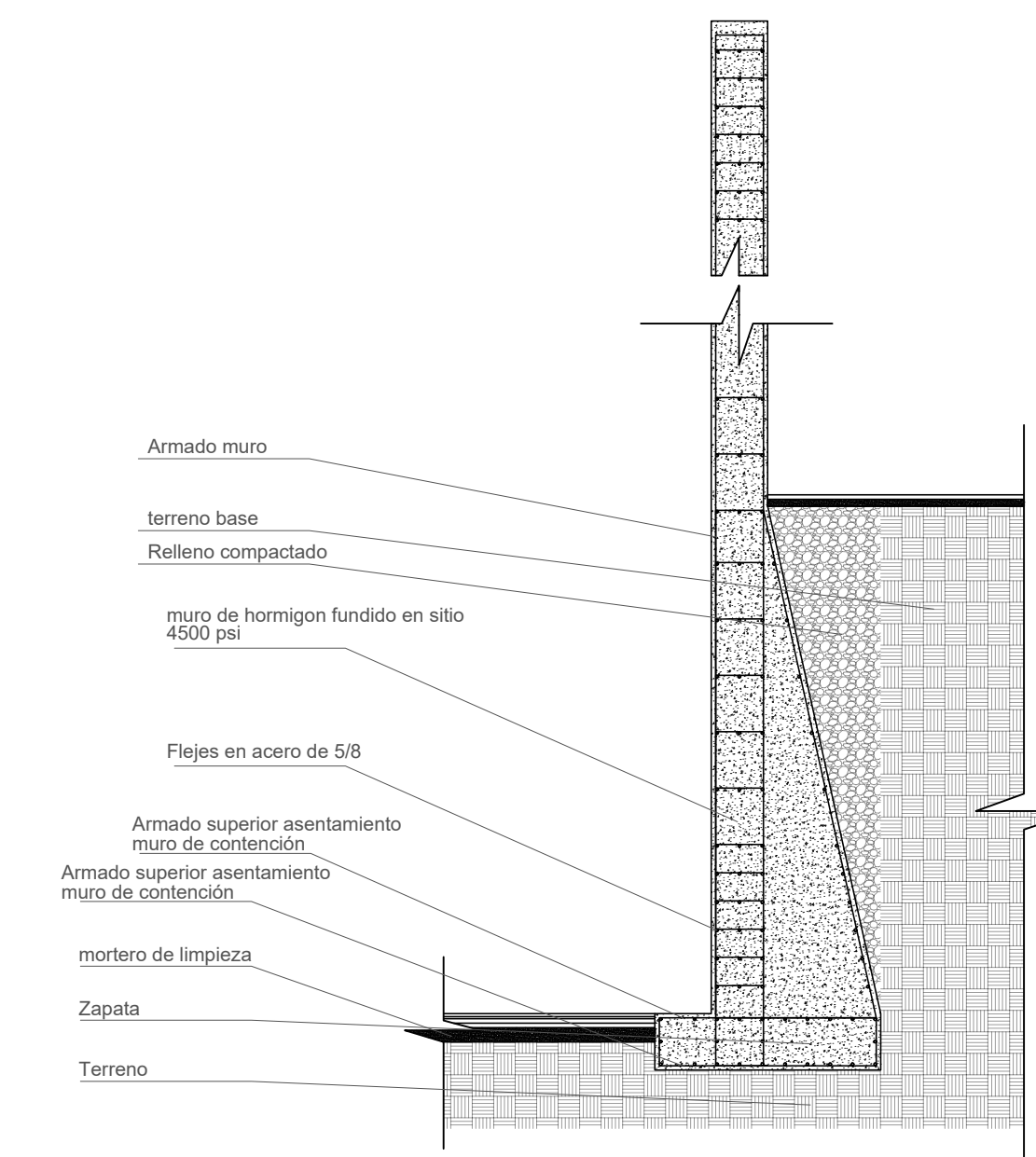
Detalle Muro de contención Escala 1:50
