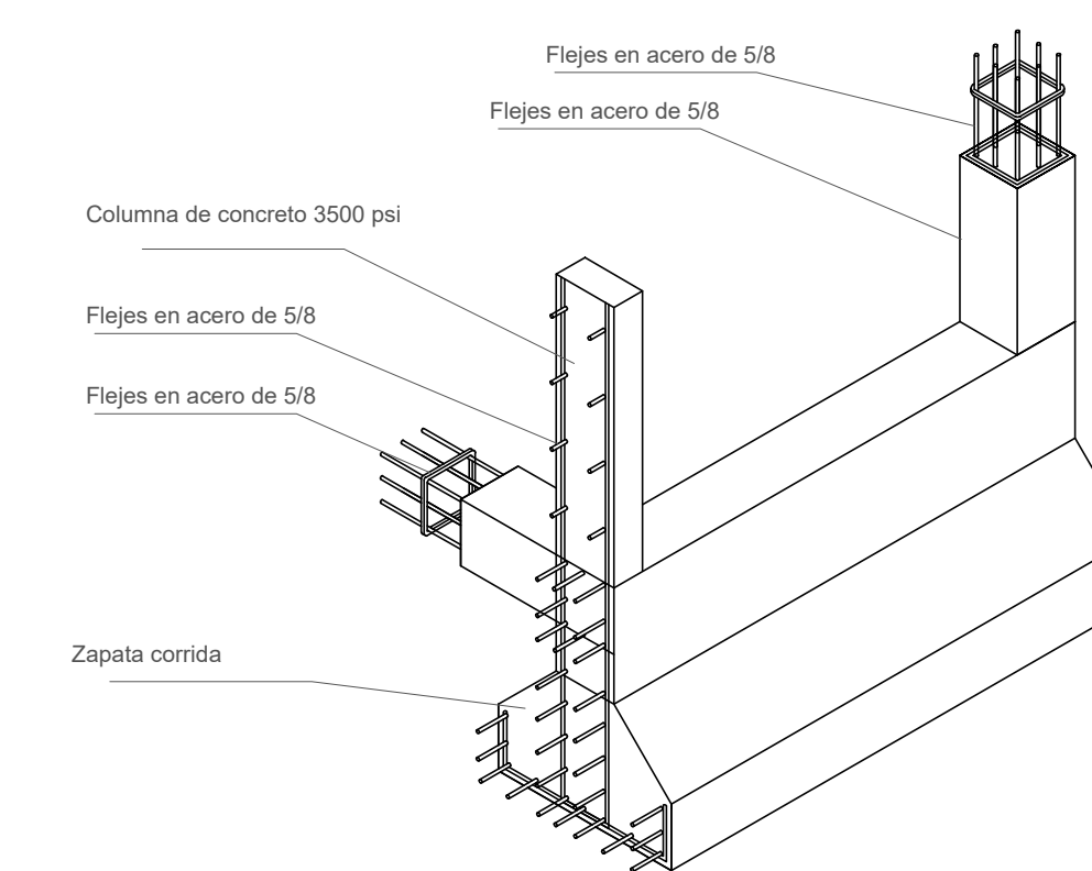
Detalle zapata corrida Escala 1:50
