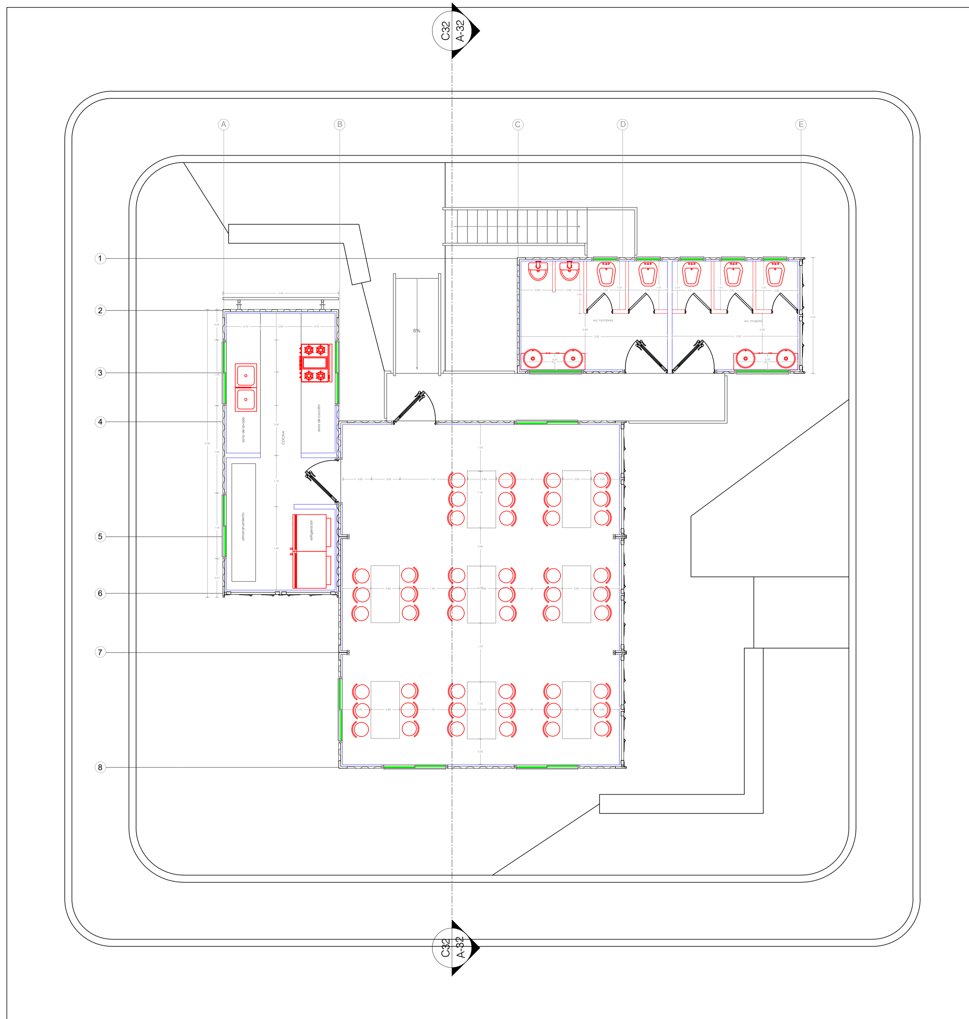
A32 PLANTA MODELO ILUSTRATIVO ESCALA 1:50
