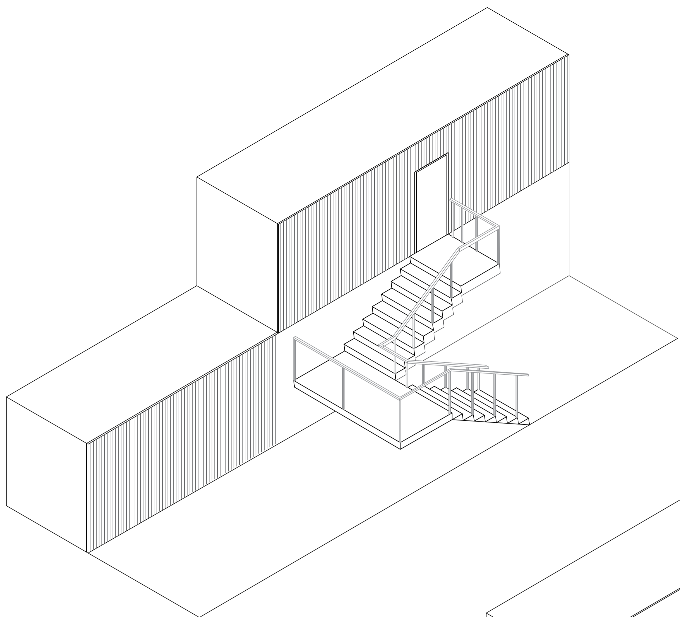
D6 ISOMETRICO ESCALERA EN U ESCALA 1:20
