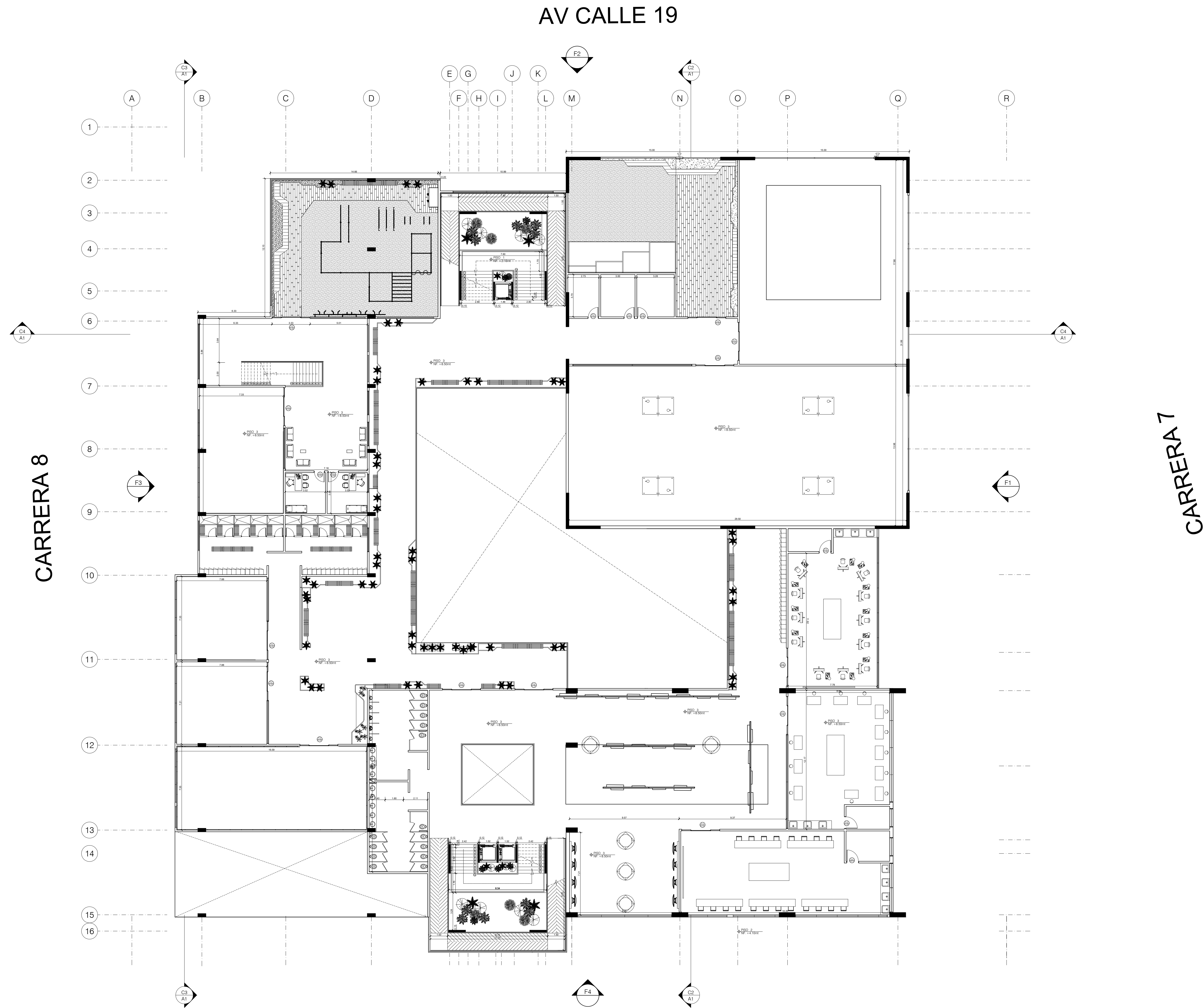
A PLANTA TERCER PISO ESCALA 1:150 CALLE 18
