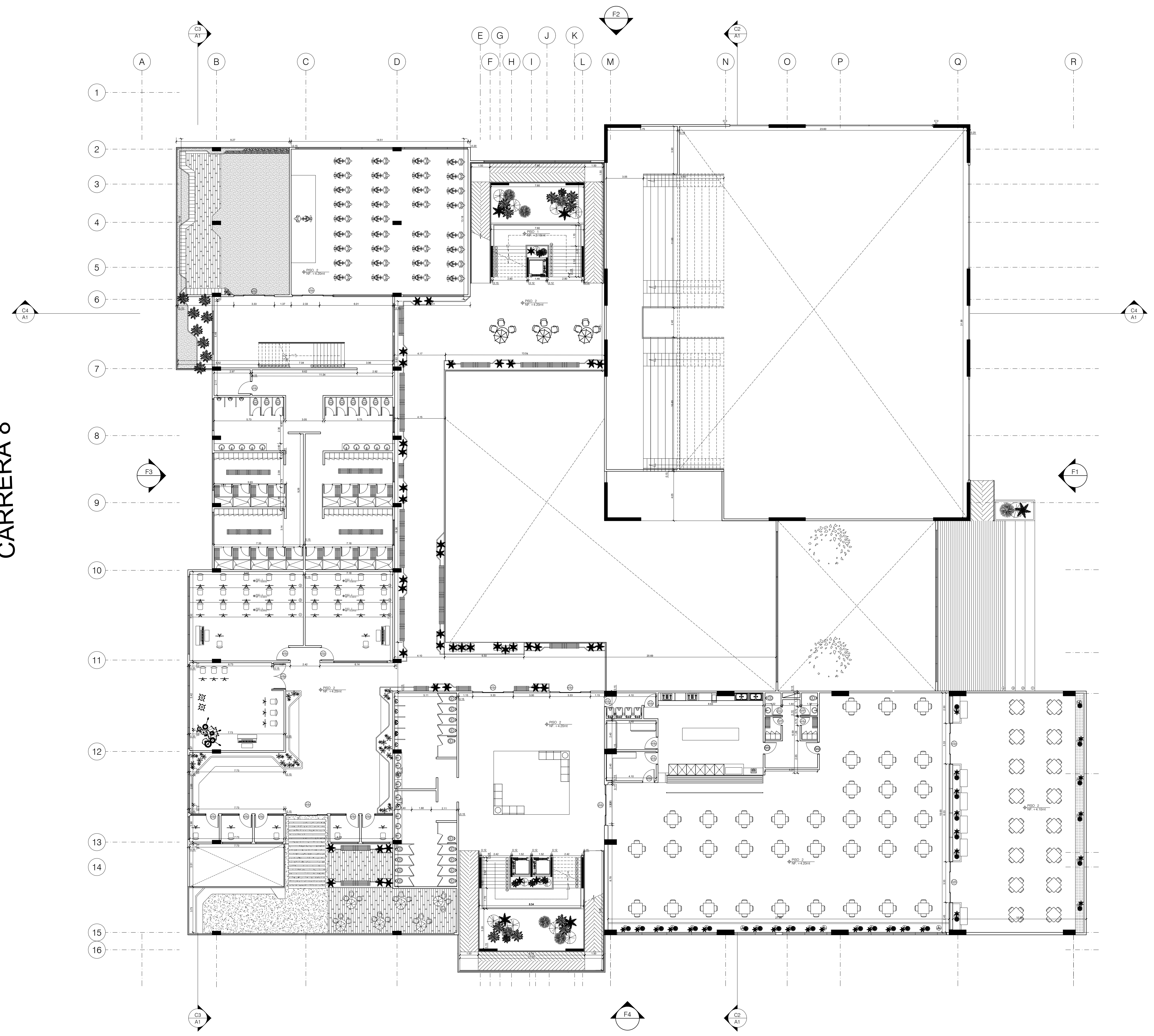
A PLANTA SEGUNDO PISO ESCALA 1:150 CALLE 18
