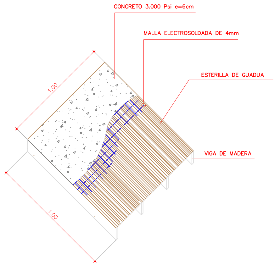
ISOMETRICO PLACA ESTERILLA DE GUADUA ESC: 1:25
