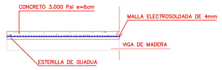
CORTE PLACA ESTERILLA DE GUADUA ESC: 1:25
