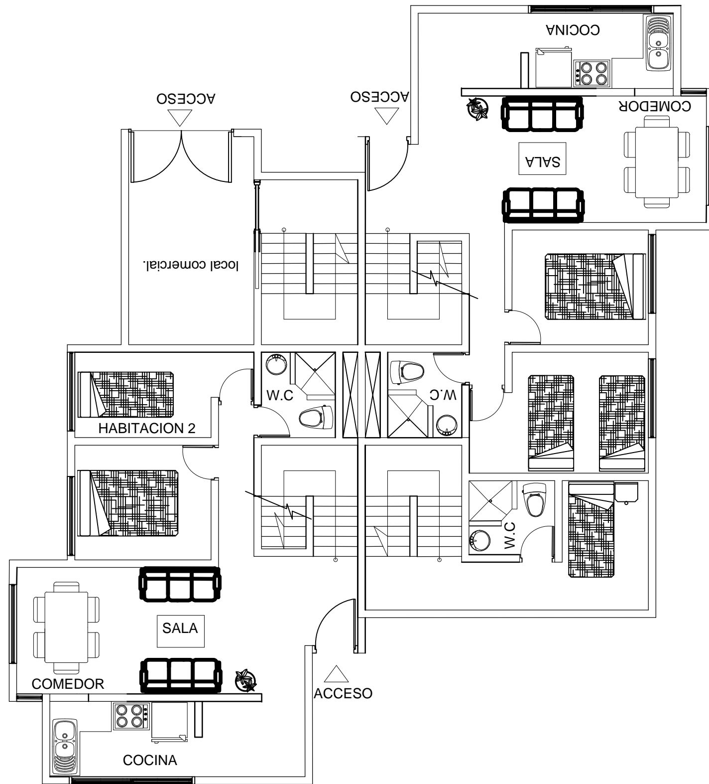
Planta con desarrollo progresivo de la vivienda Esc. 1.75
