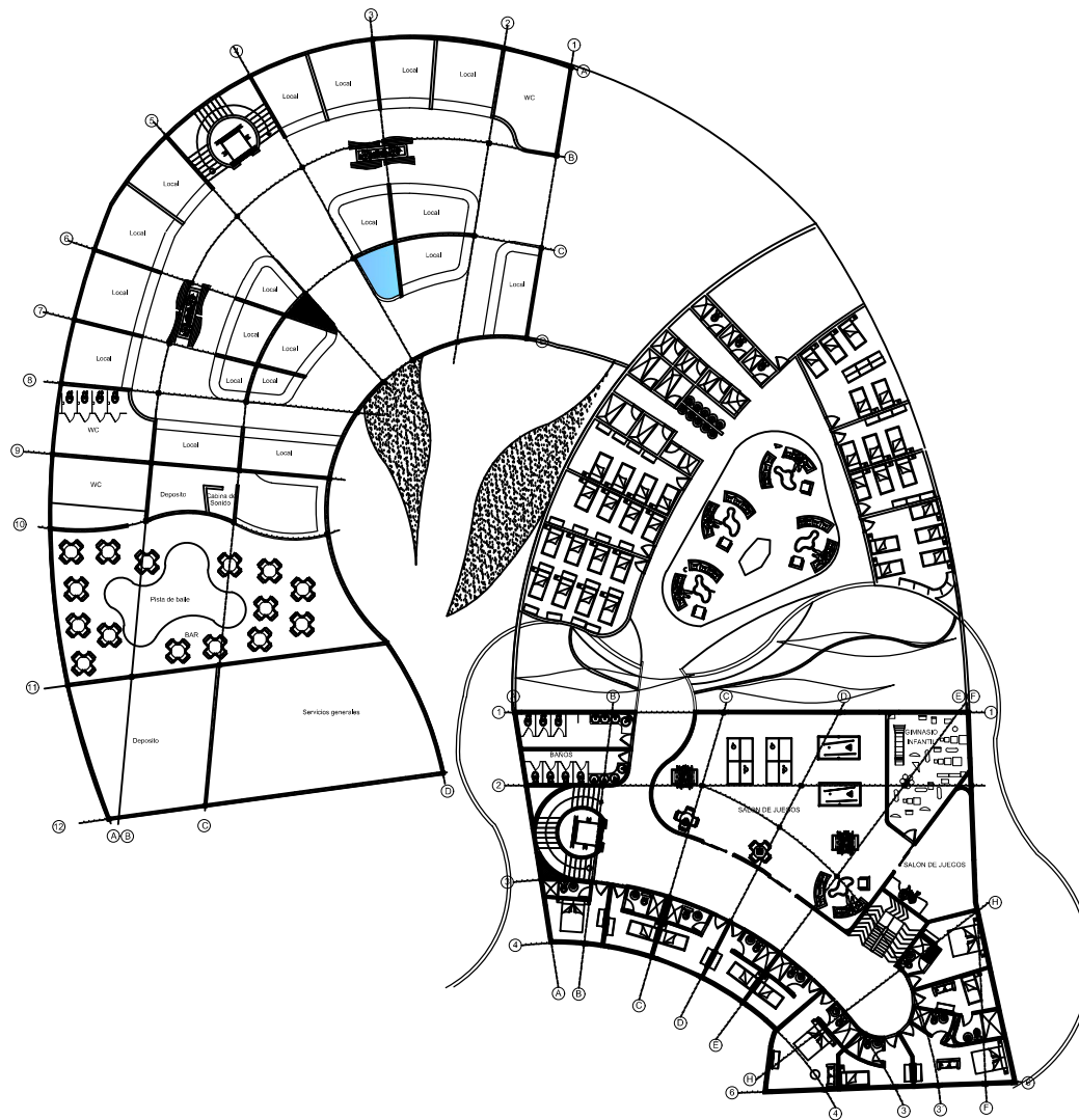
TERCER PISO
