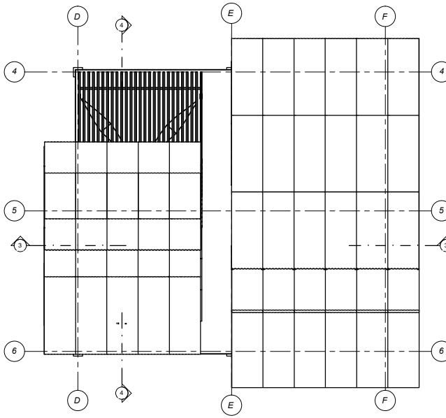
2 - Planta de cubierta A101 1:50
