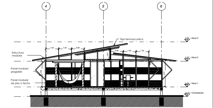
4 - Corte 2 A101 1:50
