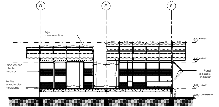
3 - Corte 1 A101 1:50
