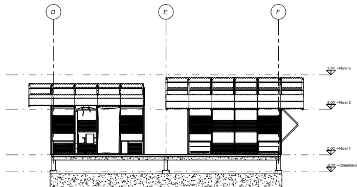
8 - Fachada Frontal A101 1:50
