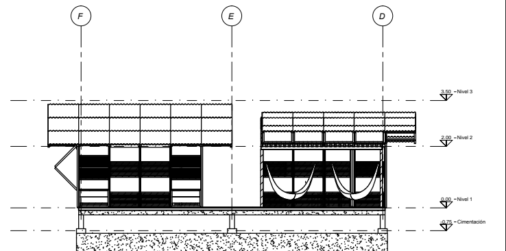
9 - Fachada Posterior A101 1:50
