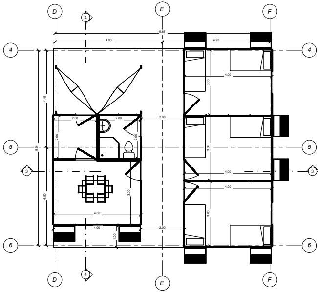
1 - Nivel 1 A101 1:50
