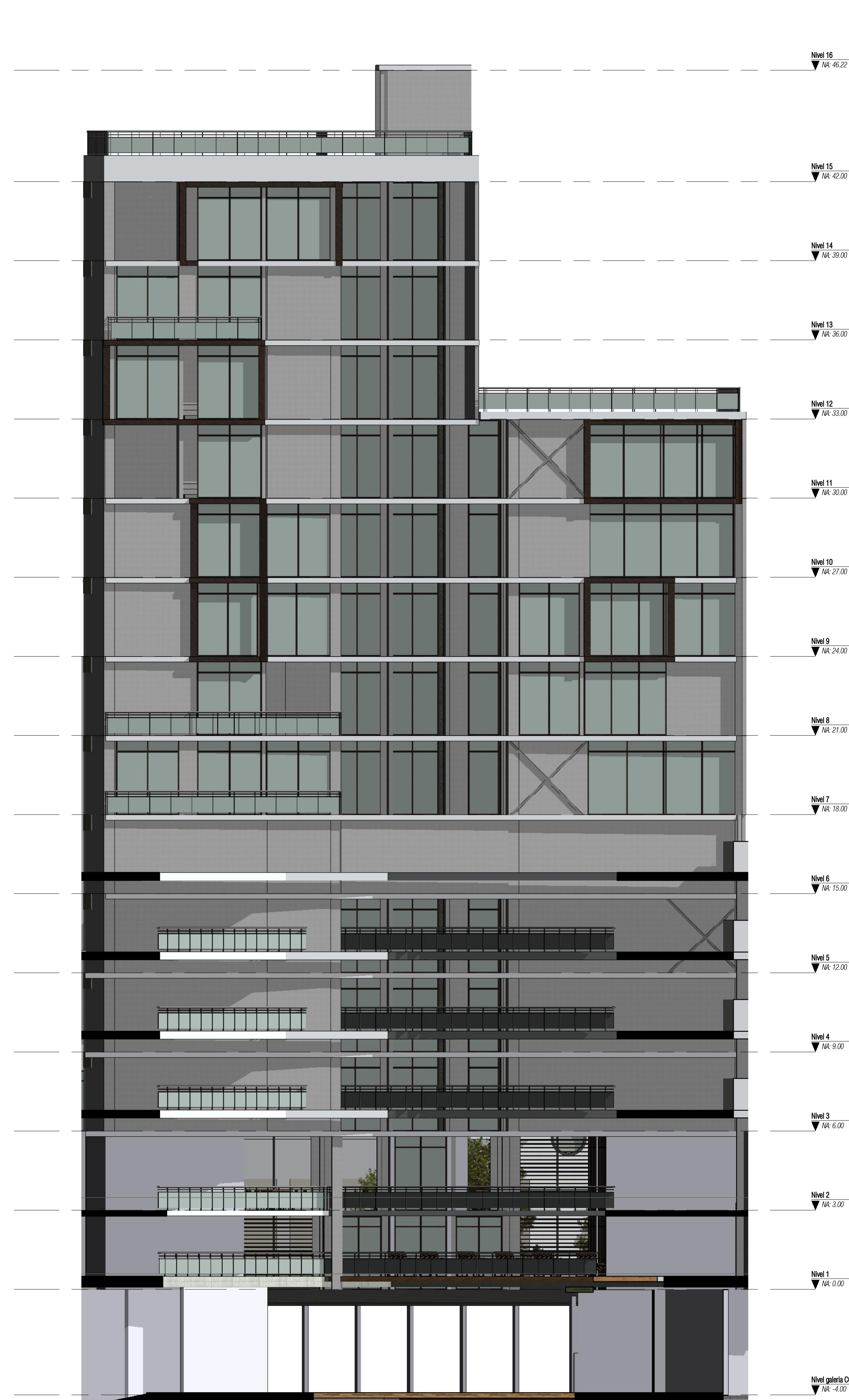
25 FACHADA POSTERIOR ESCALA: 1 : 100
