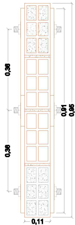
VISTA LATERAL
