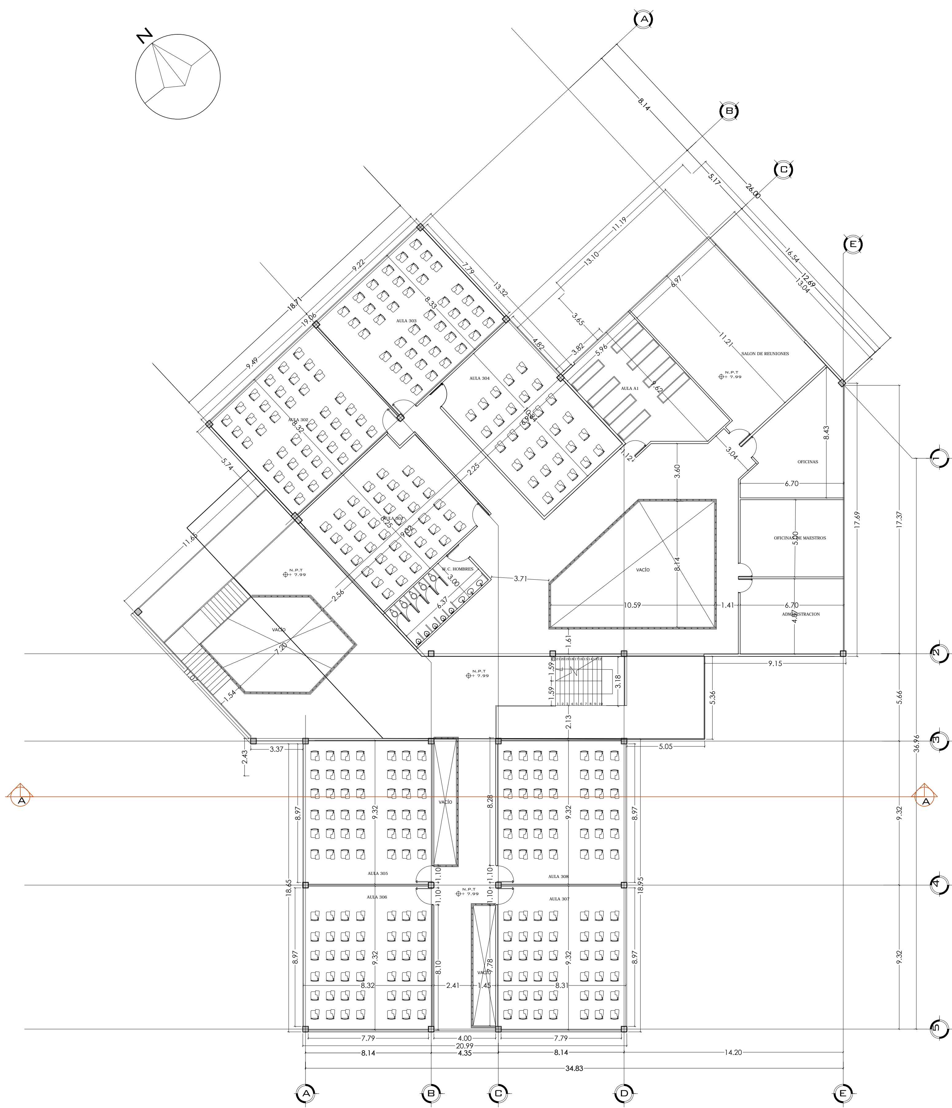
3 PISO Esc: 1.150
