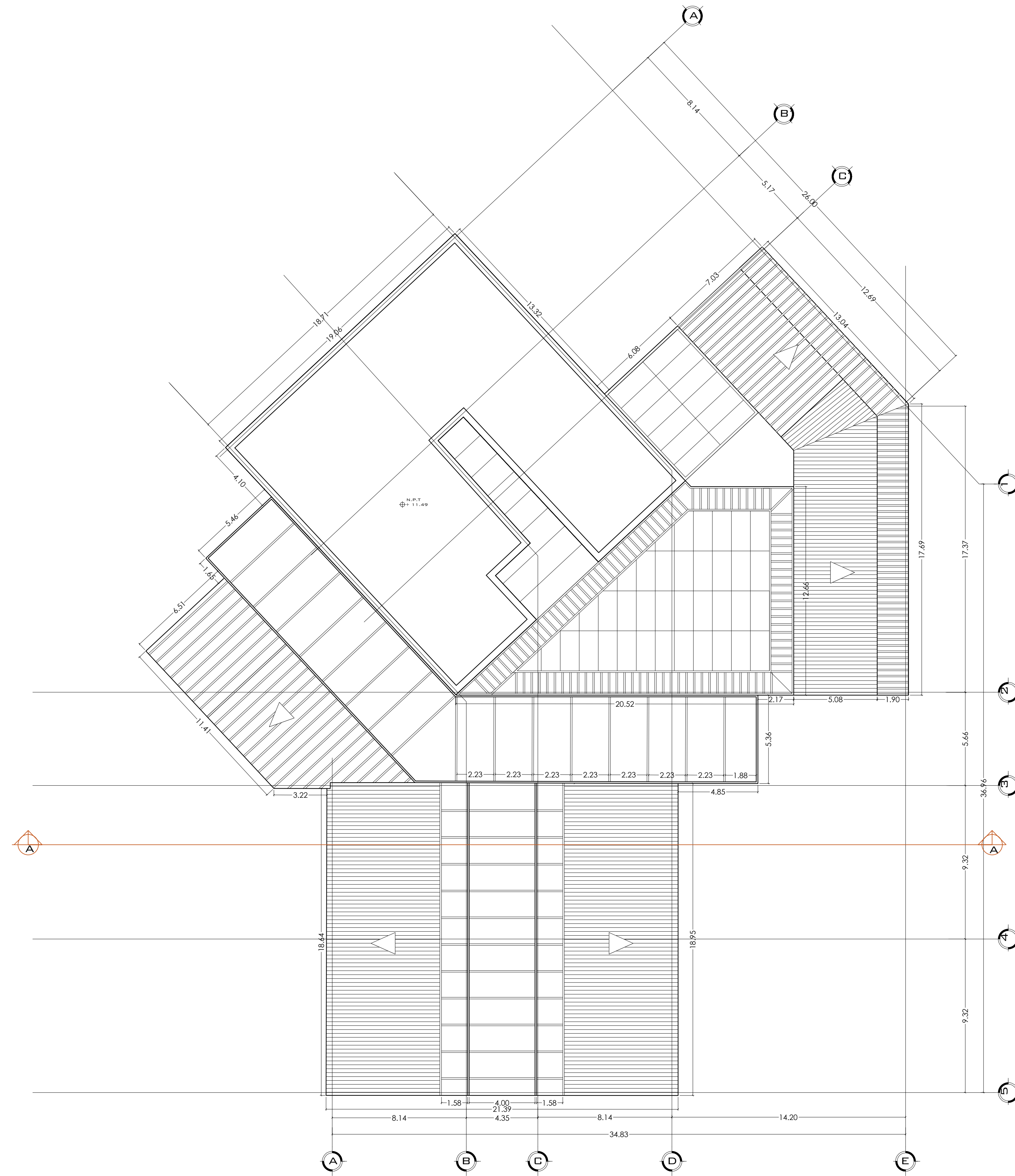
PLANTA CUBIERTAS Esc: 1.150
