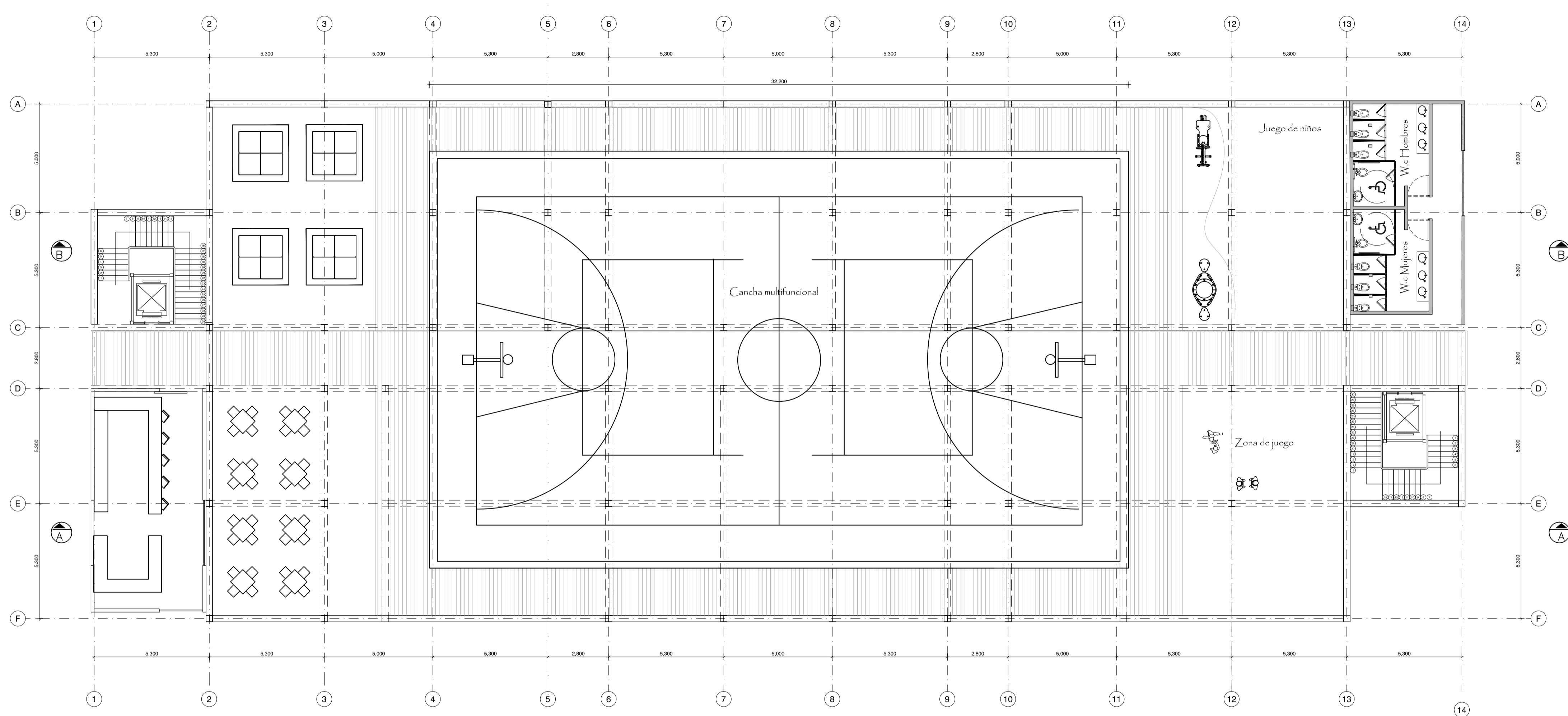
PLANTA CUBIERTA TRANSITABLE
