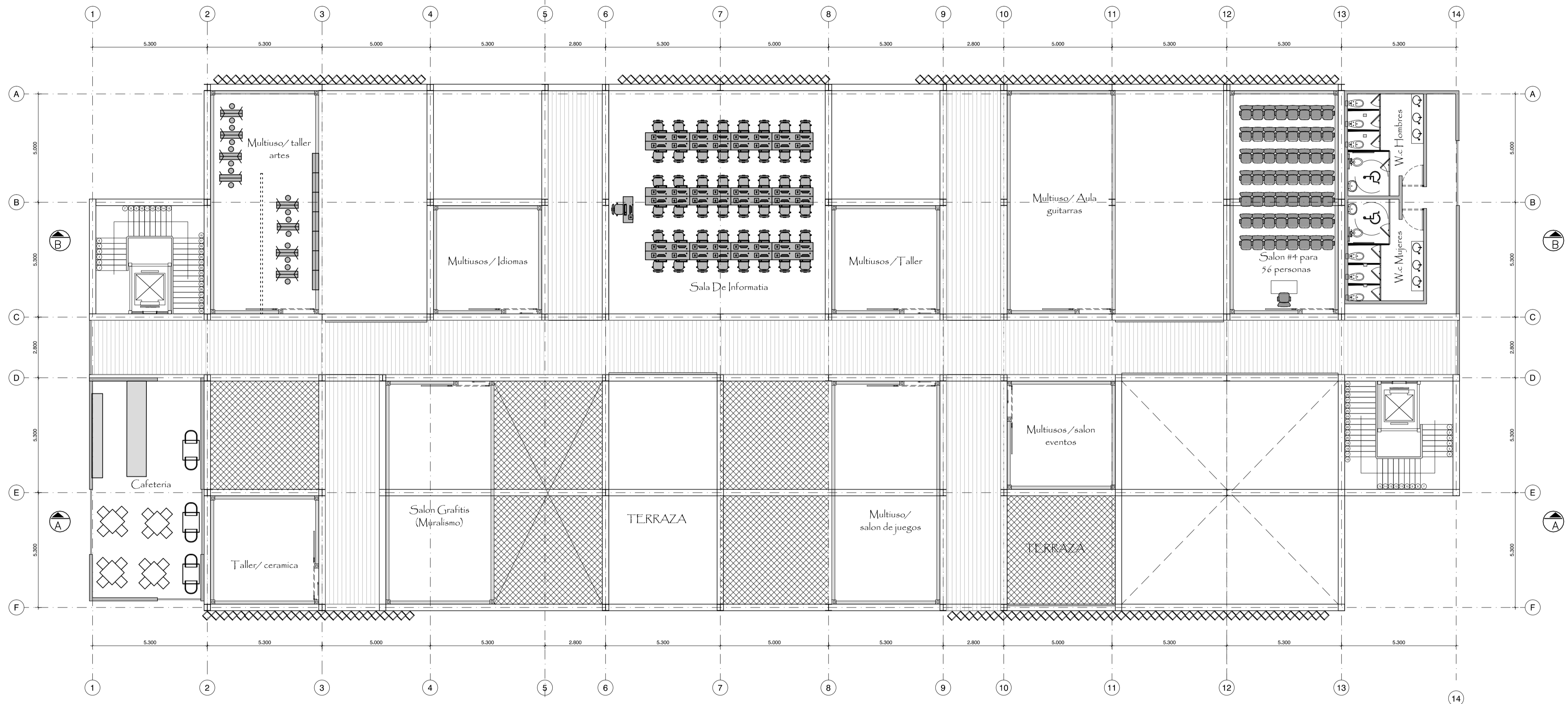
PLANTA CUARTO NIVEL
