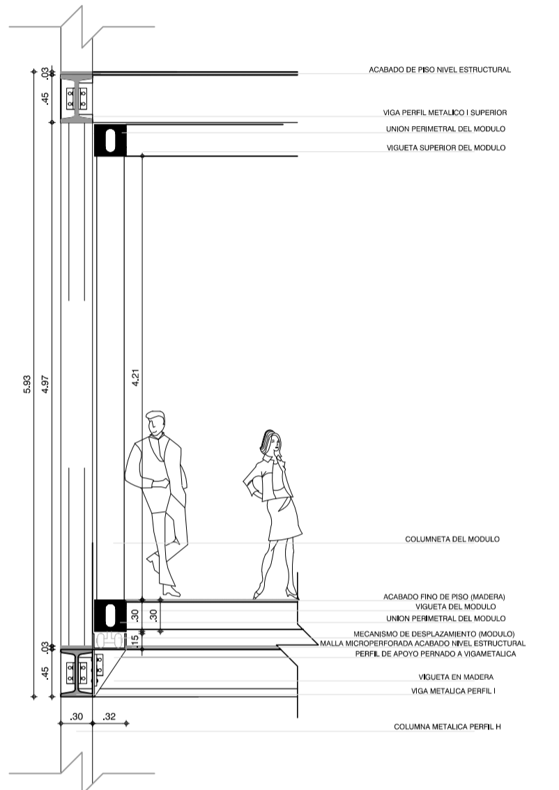
DETALLE MODULO HORIZONTAL Eac: 1:50
