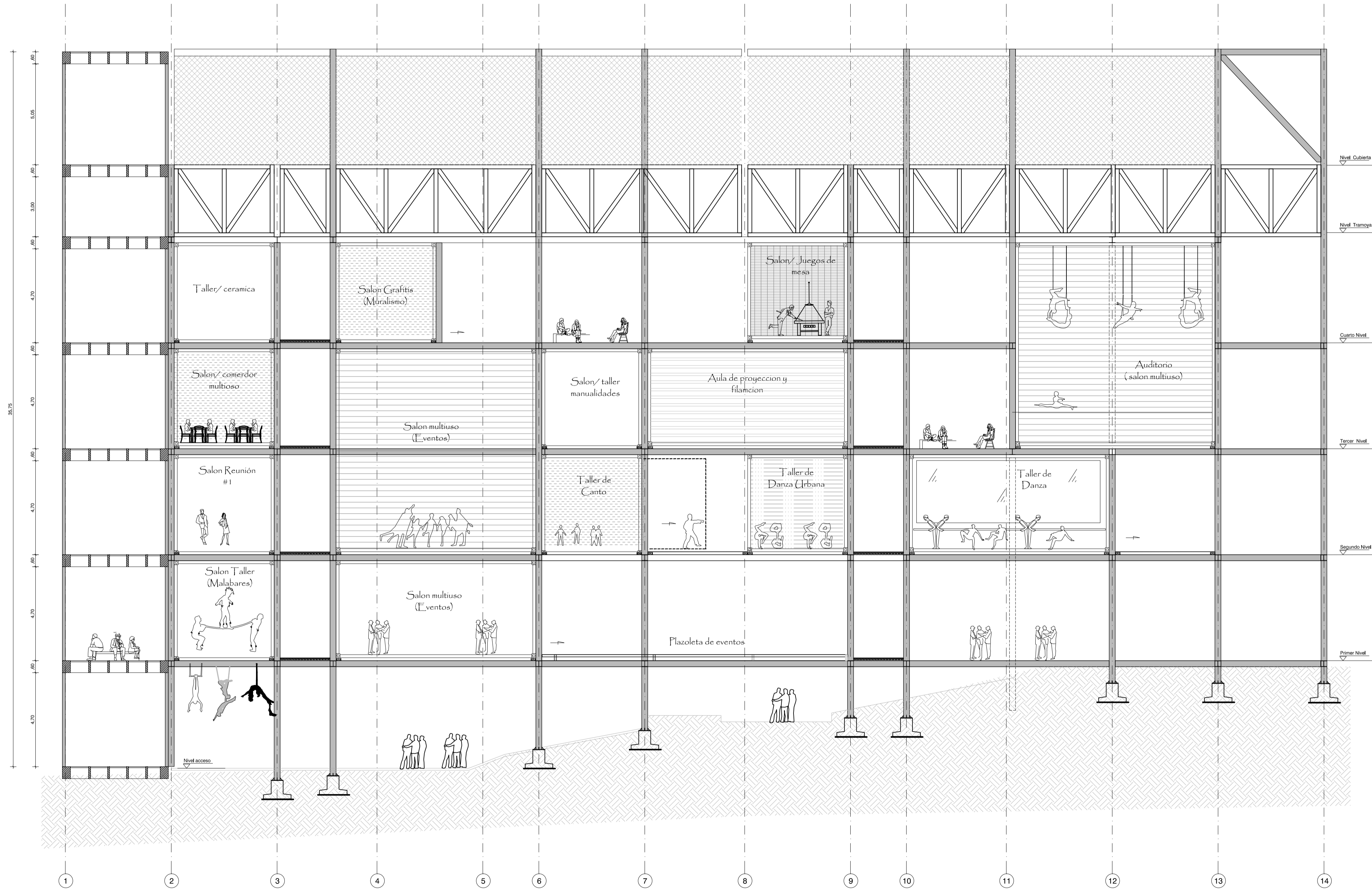
CORTE A-A
