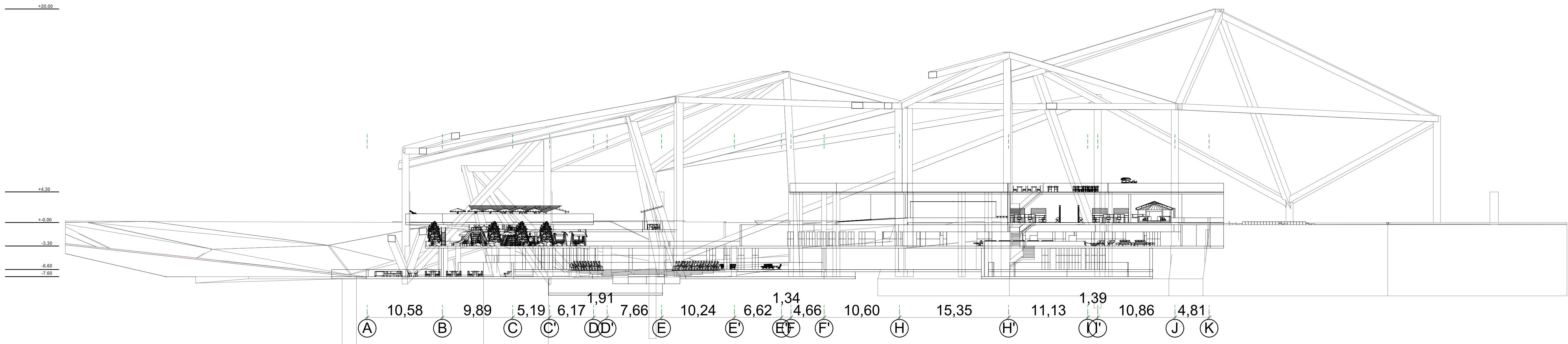
C2 CORTE 2 - 2 ESC. 1:300
